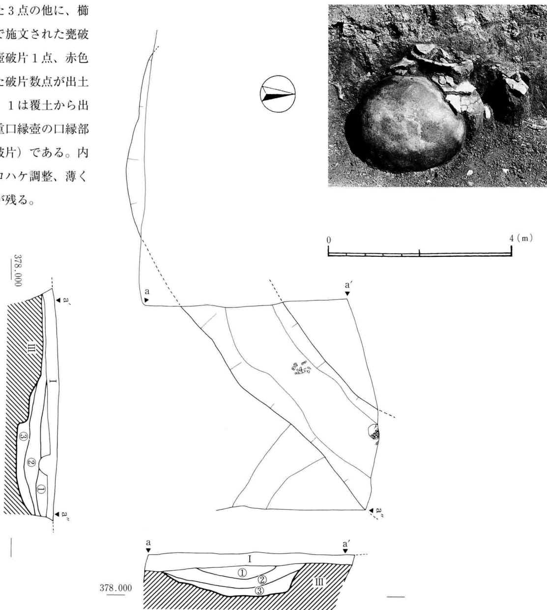
図6 SD1遺構図・壁面図(1:80)
