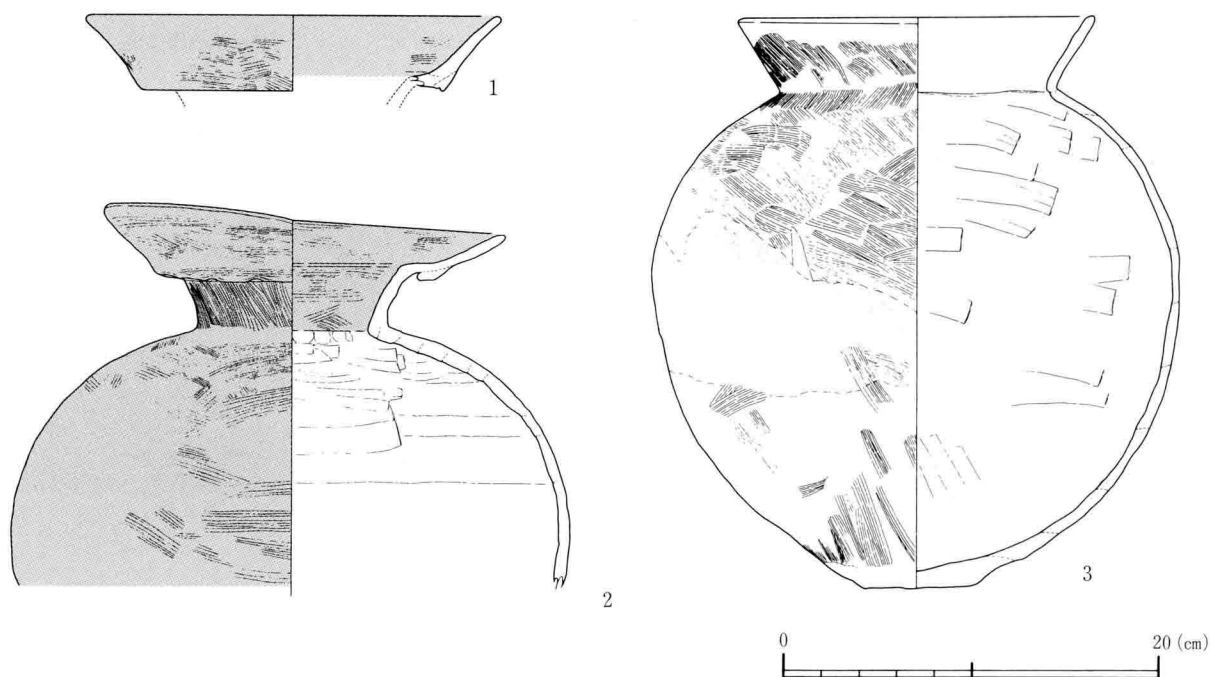
図7 SD1出土土器実測図(1:4)
