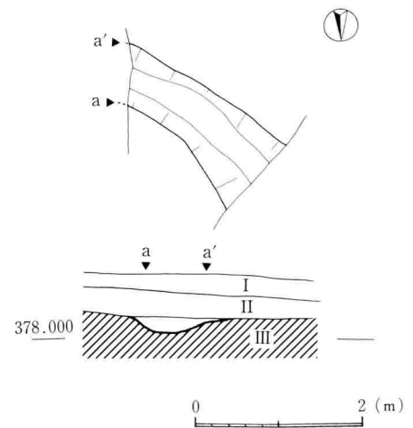
図 8 SD 2 遺構・壁面図 (1:80)
