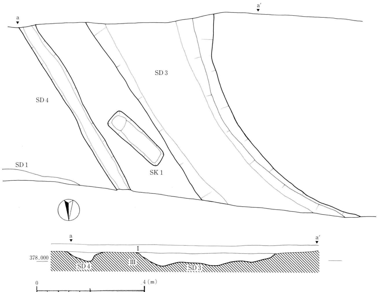
図 9 SD 3・4、SK 1 遺構図・壁面図 (1:80)
