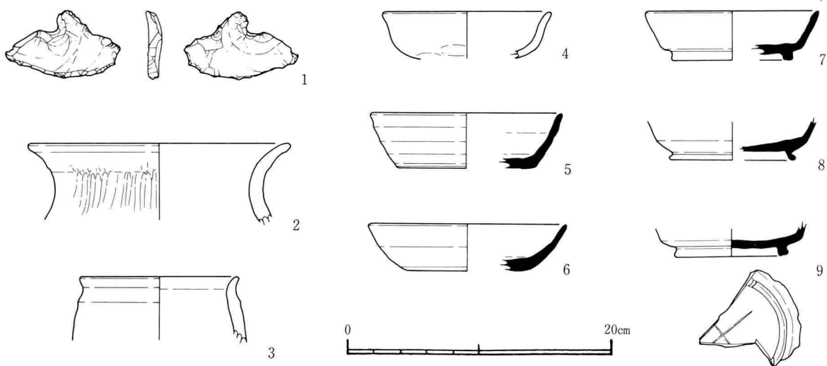
図11 SD3出土遺物実測図 (石器1:2・土器1:4)
