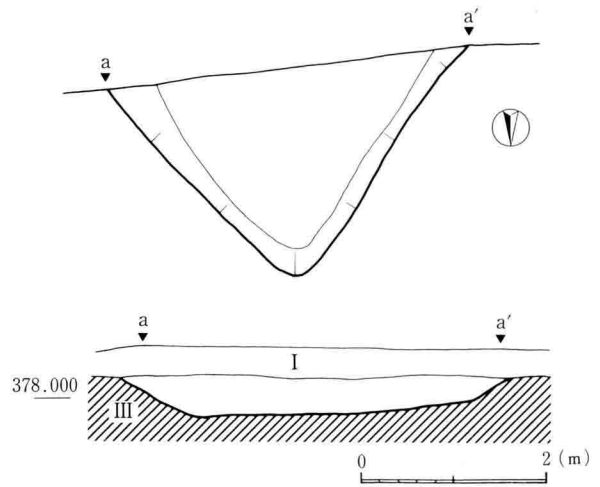
図10 SK2遺構実測図・壁面図 (1:80)
