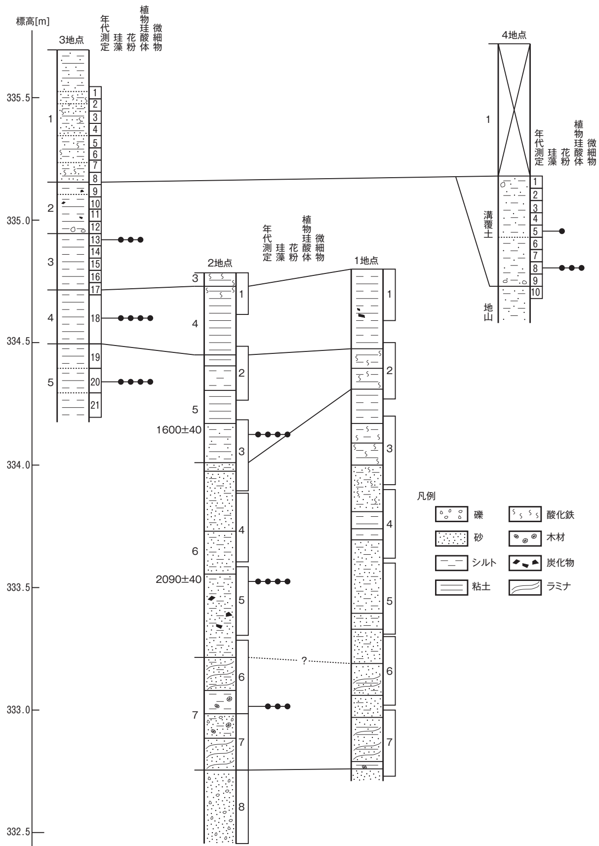
図2 各地点の対比図・試料採取位置図および分析層位
