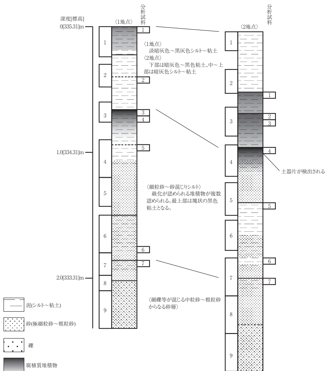
図1 ボーリング調査地点柱状図
