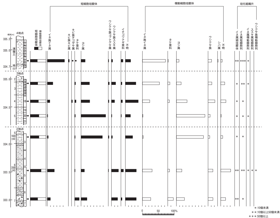
図5 物珪酸体群集と珪化組織片の産状
