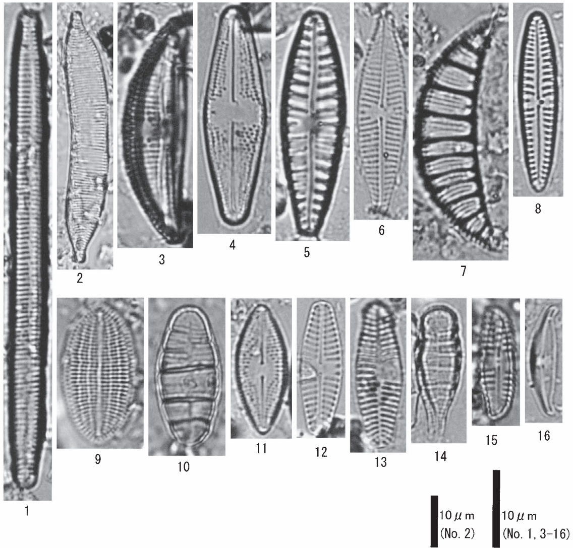
图版1 珪藻化石
