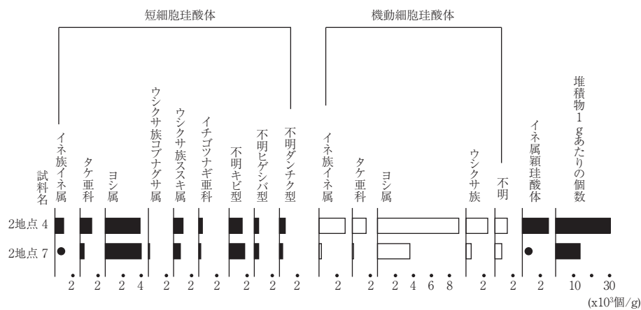
図5 植物珪酸体含量
