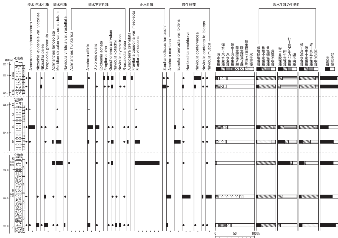
図3 主要珪藻化石群集の層位分布
