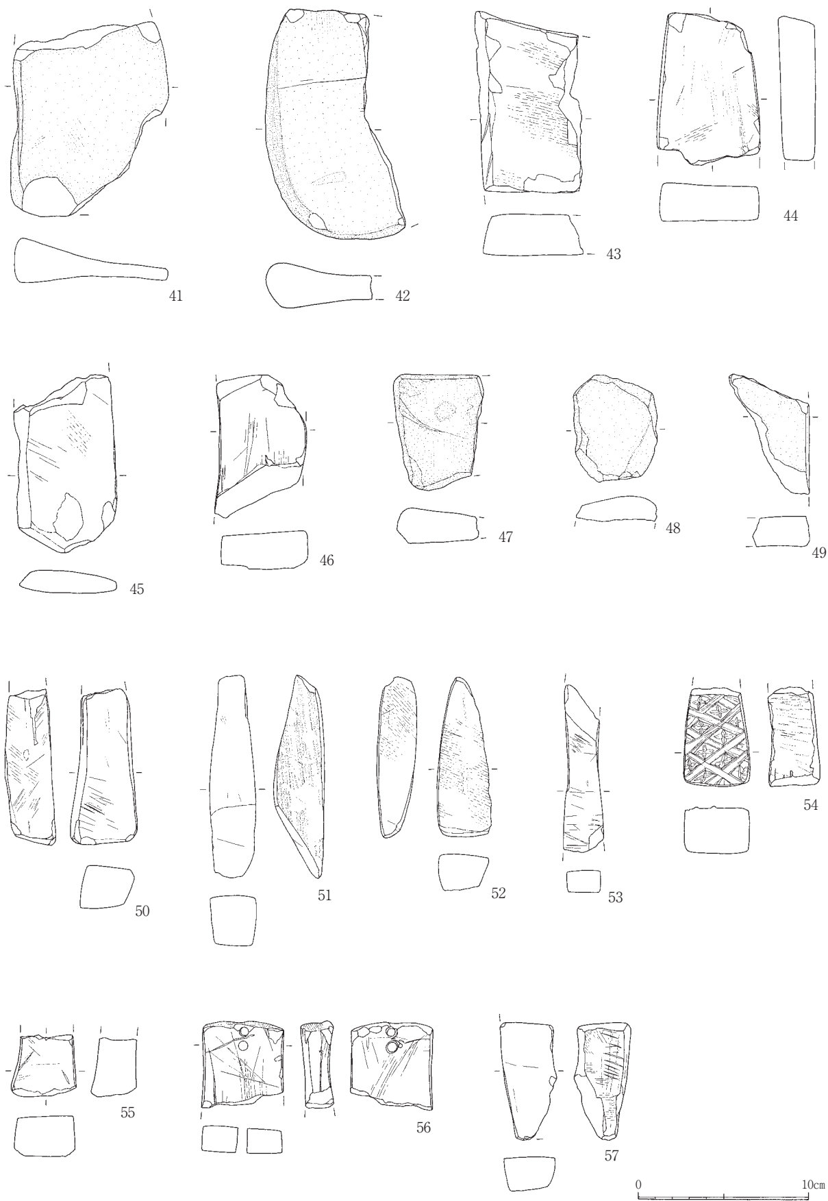
图51 石製品実測図① (1 : 3)
