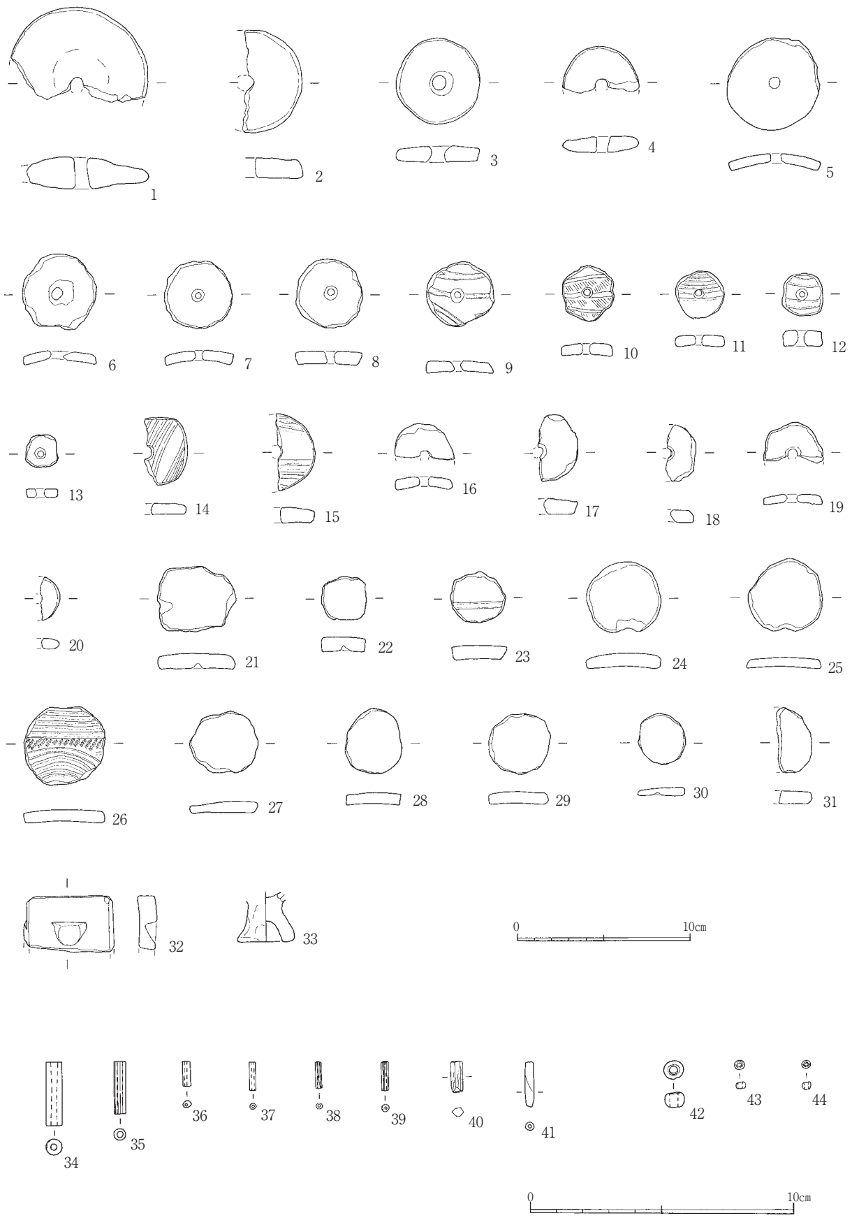
图53 土製品・玉類実測図（土製品=1:3、玉類=1:2）
