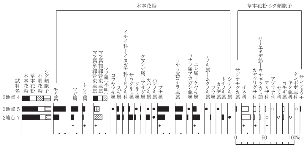
出現率は、木本花粉は木本花粉化石総数、草本花粉・シダ類胞子は総数より不明花粉を除く数を基数として百分率で算出した。なお、●○は1%未満、+は木本花粉100個体未満の試料について検出した種類を示す。
