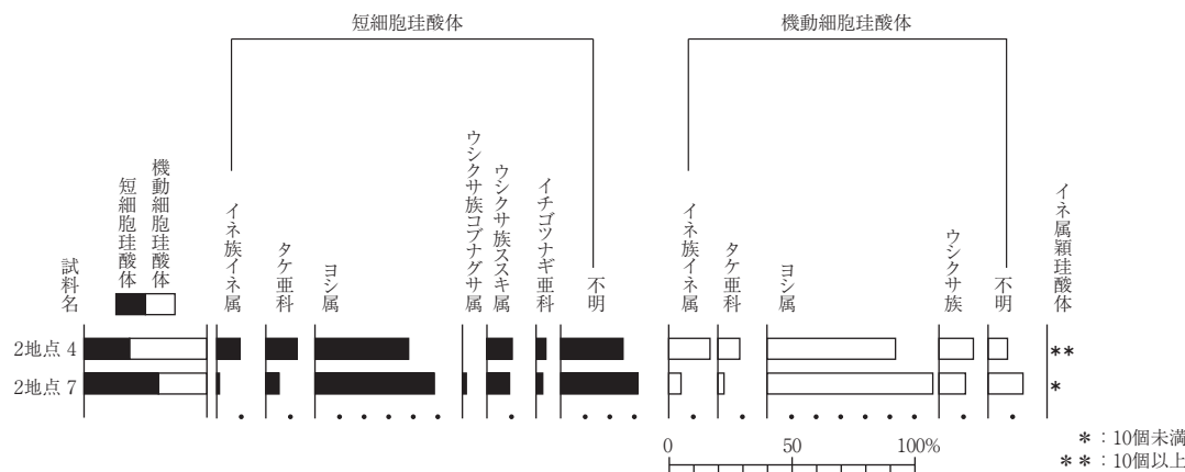
図4 植物珪酸体群集
