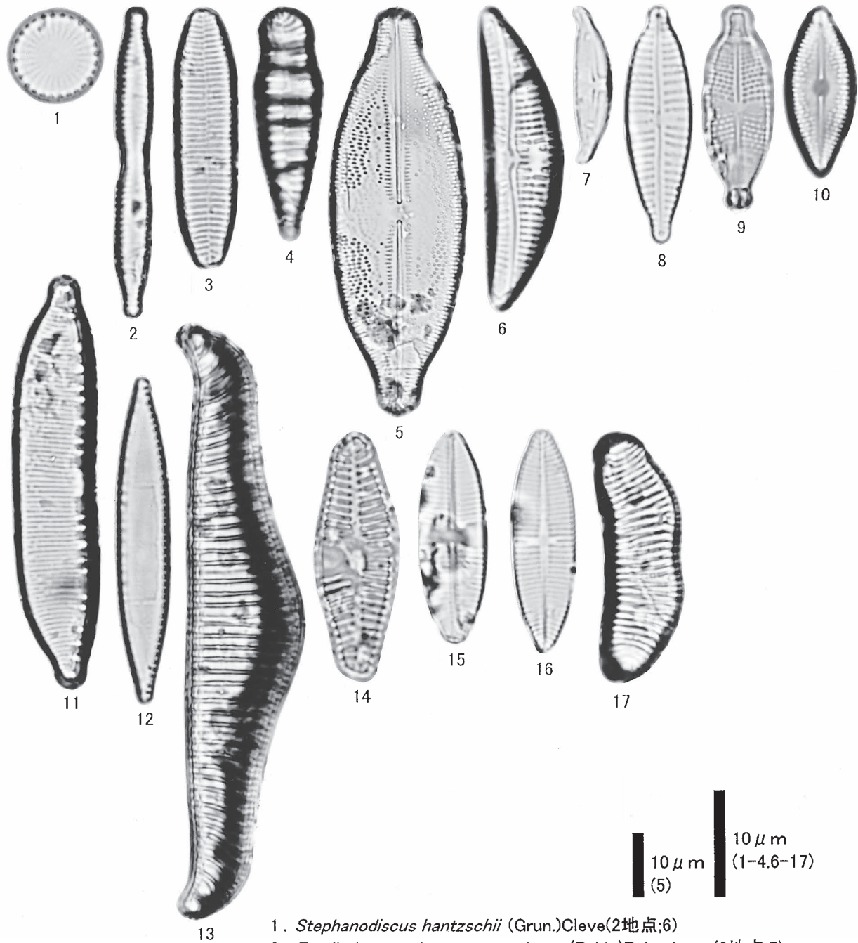
图版1 珪藻化石
