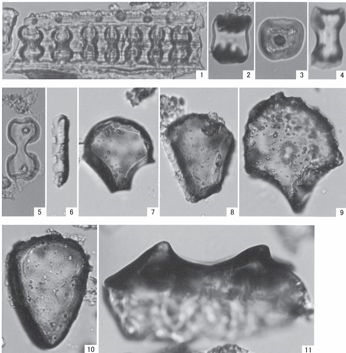
図版3 植物珪酸体
