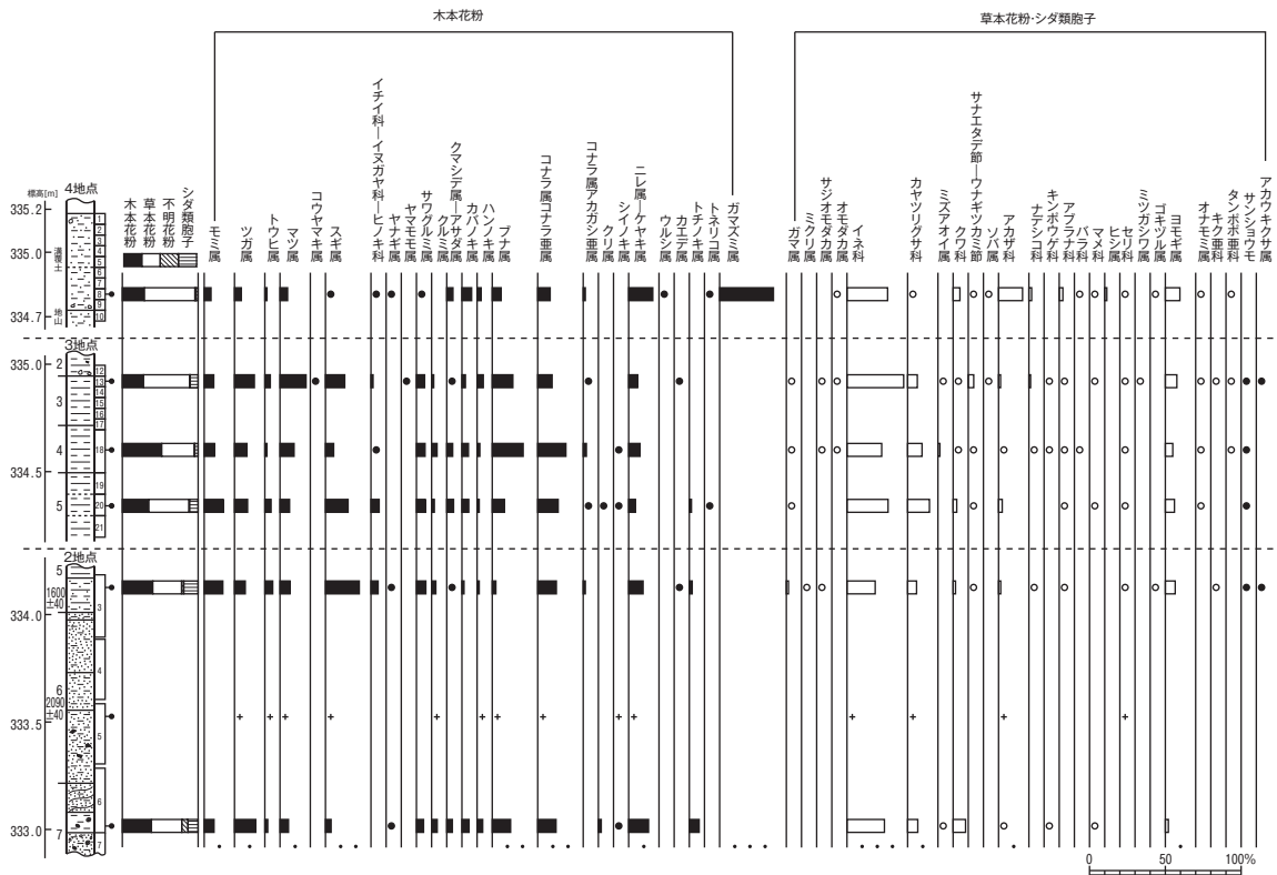
図4 主要花粉化石群集の層位分布
