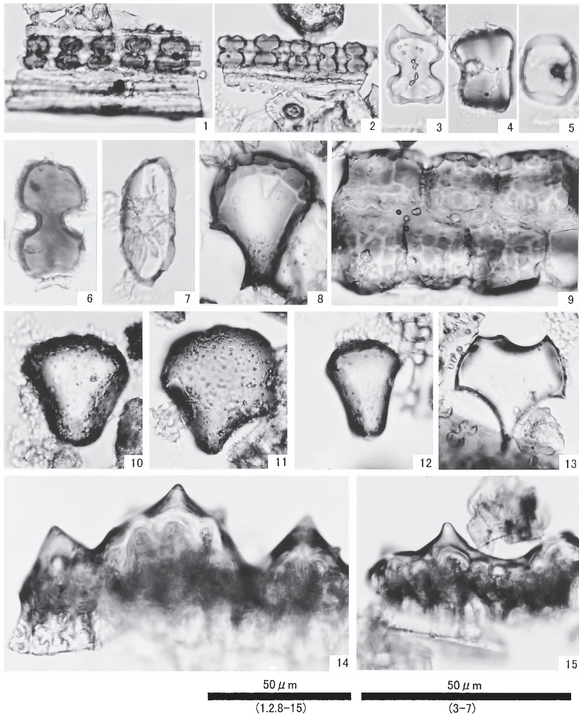
図版3 植物珪酸体
