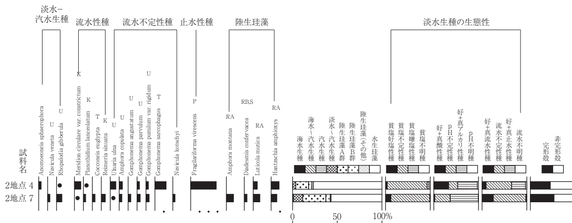
汽水-淡水生種産出率・各種産出率・完形殻産出率は全体基数、淡水生種の生態性の比率は淡水生種の合計を基数として百分率で算出した。いずれも100個体以上検出された試料について示す。なお、●は2%未満の産出を示す。 (K: 中～下流性河川指標種, O: 沼沢湿地付着生種, P: 高層層原指標種, S: 好汚濁性種, U: 広域適応性種, T: 好清水性種, RA: 陸生珪藻A群, RB: 陸生珪藻B群, RI: 未区分陸生珪藻)
