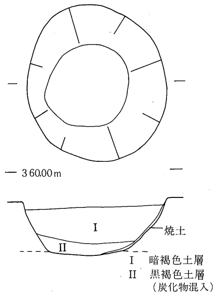
第10図 2号土壌(1/40)
