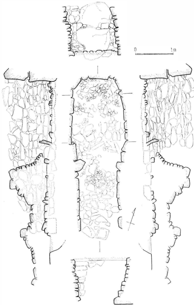
第4図 長原第5号墳石室実測図 (1:60)
