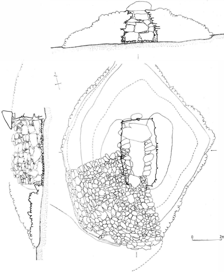
第9図 長原第7号墳墳丘実測図 (1:120)
