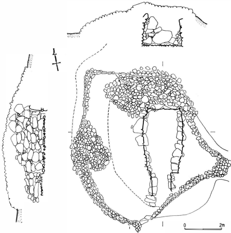
第16図 長原第11号墳墳丘実測図 (1:120)
