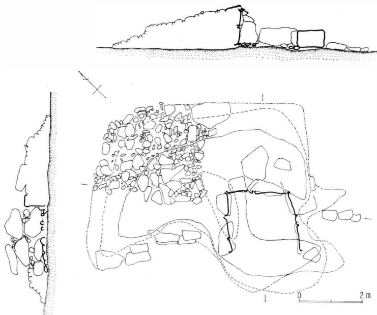
第6図 長原第6号墳墳丘実測図 (1:120)
