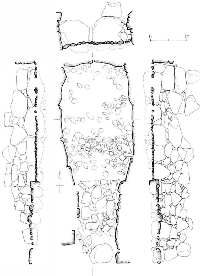
第24図 長原第13号墳石室実測図 (1:60)
