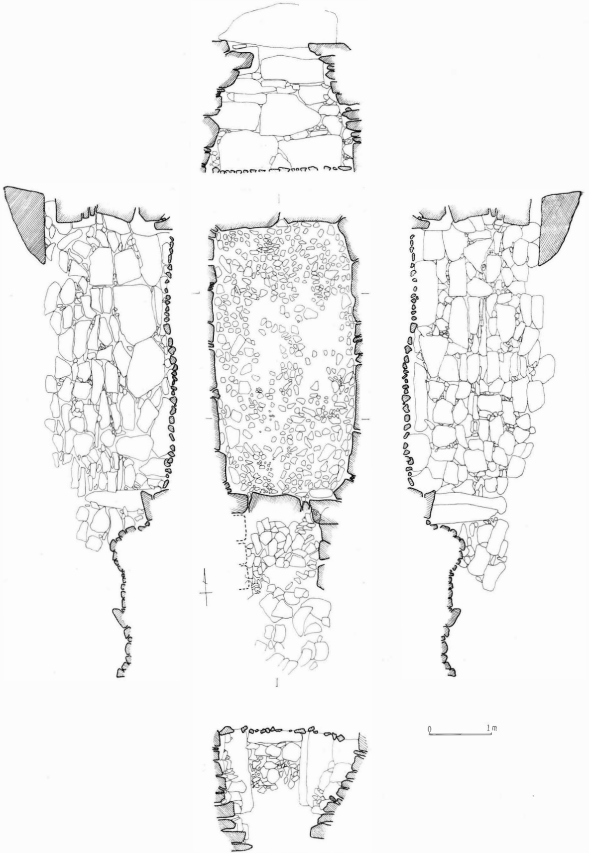
第10図 長原第7号墳石室実測図 (1:80)
