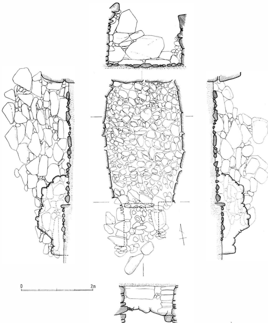
第17図 長原第11号墳石室実測図 (1:60)
