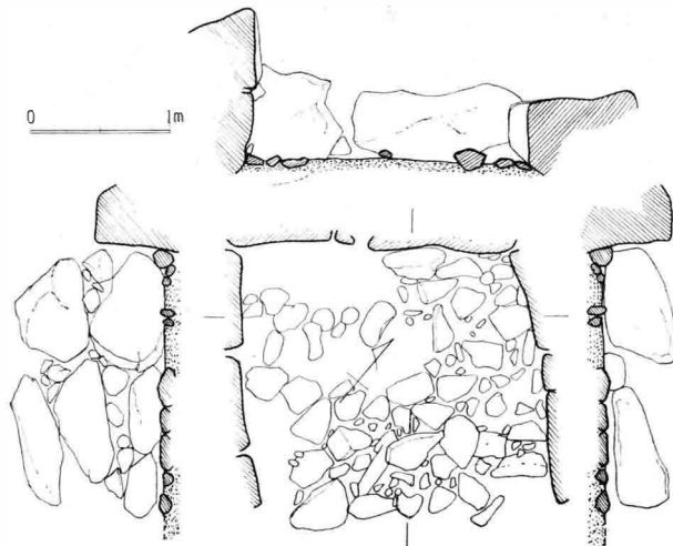
第7図 長原第6号墳石室実測図 (1:6)
