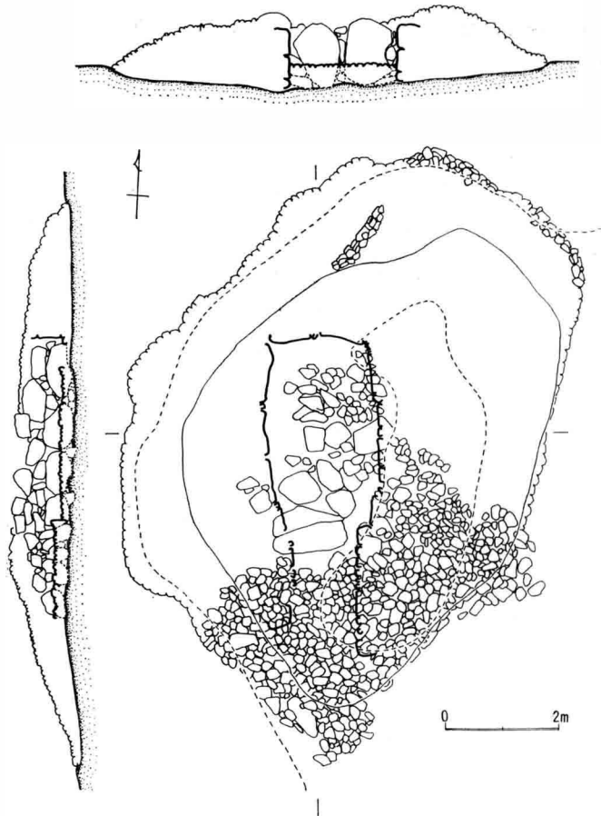
第23図 長原第13号墳墳丘実測図 (1:120)
