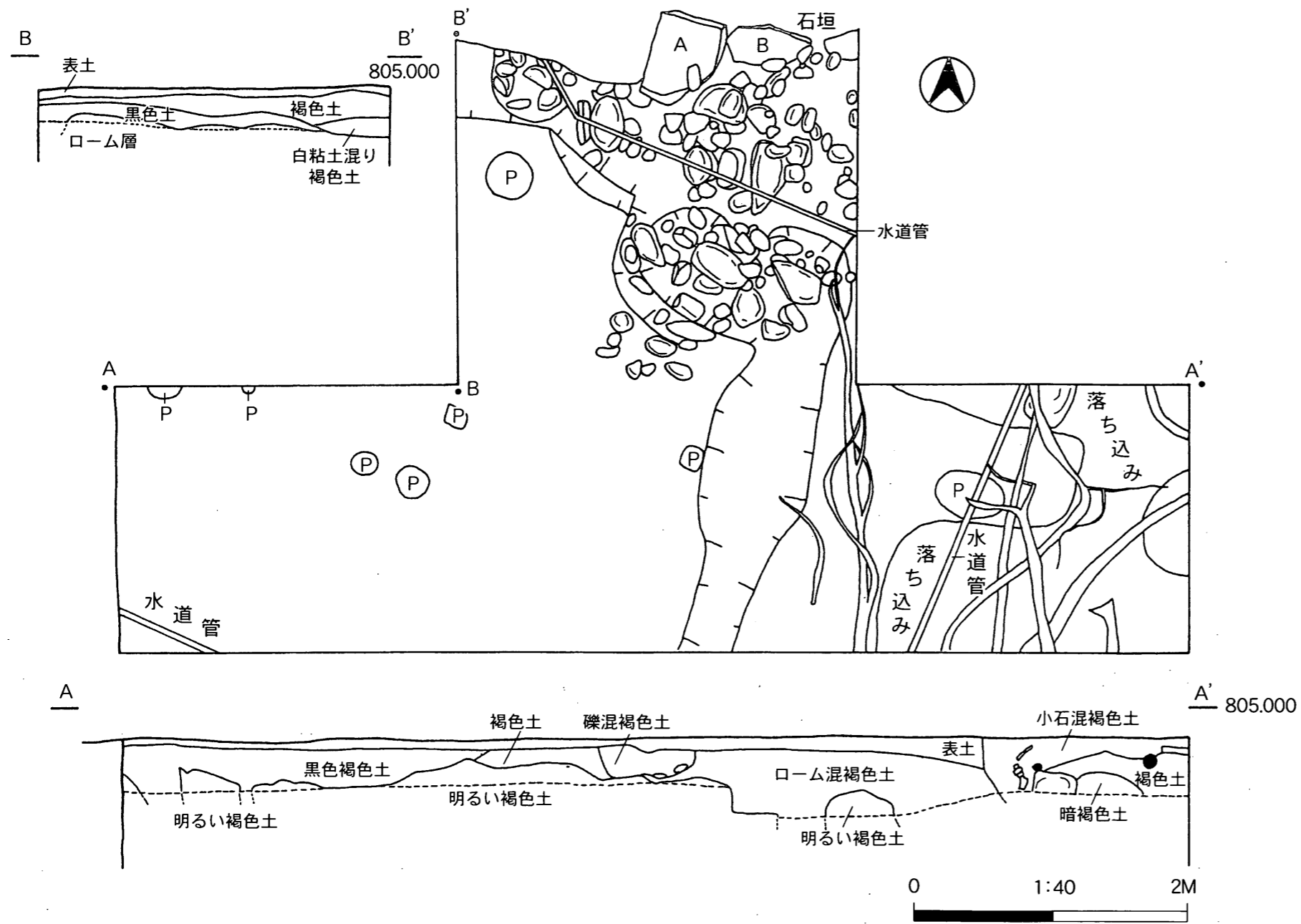
第7図 第1トレンチ平面・断面実測図(1-4~1-6)
