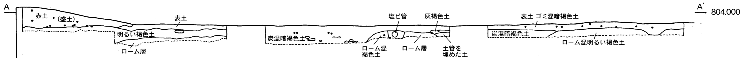
第9図 第2トレンチ平面・断面実測図(2-1~2-3)
