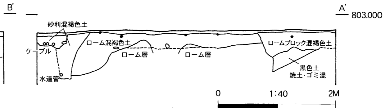
第12図 第3トレンチ平面・断面実測図(3-1~3-2)
