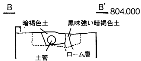
2-2区 土管断面図
