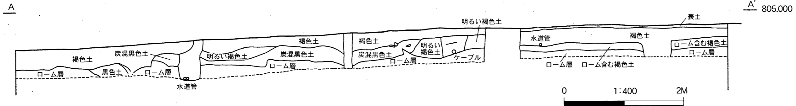
第6図 第1トレンチ平面・断面実測図(1-0~1-3)
