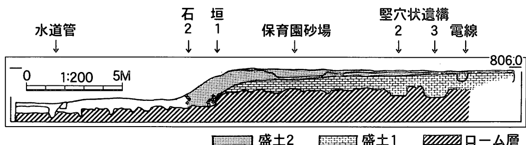
第13図 高遠閣周辺土層断面図
