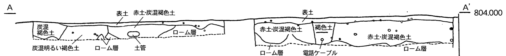
第10図 第2トレンチ平面・断面実測図(2-4~2-5)
