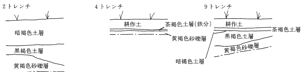
第5図 峯遺跡土層断面図 (1/40)
