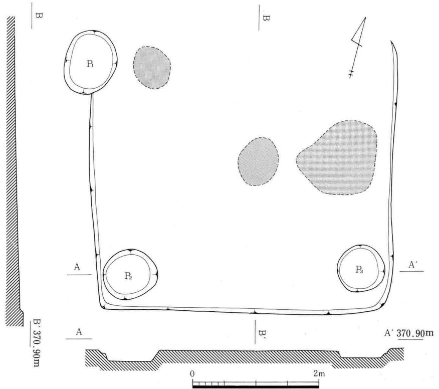
III-197 B19号住居址実測図
