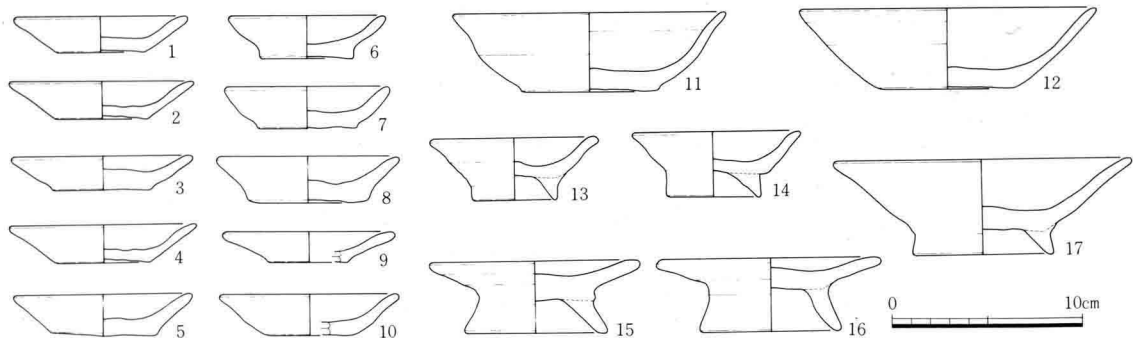
Ⅲ-154 B 2 号住居址出土土器実測図
