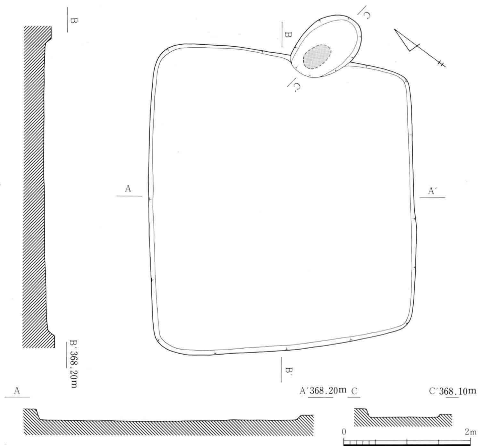
Ⅲ-214 A 2号集石址実測図
