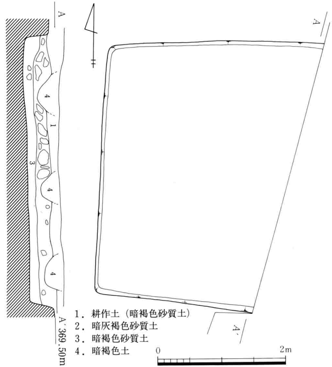
Ⅲ-158 B 4 号住居址実測図
