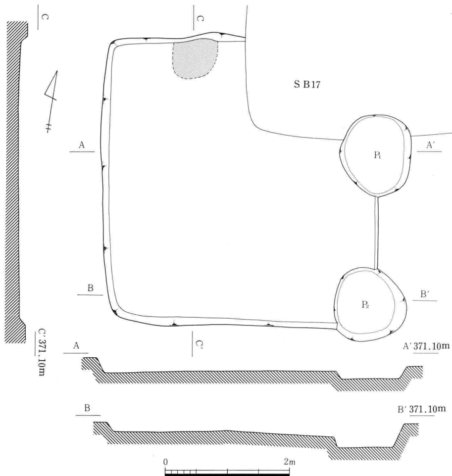
III-195 B18号住居址実測図
