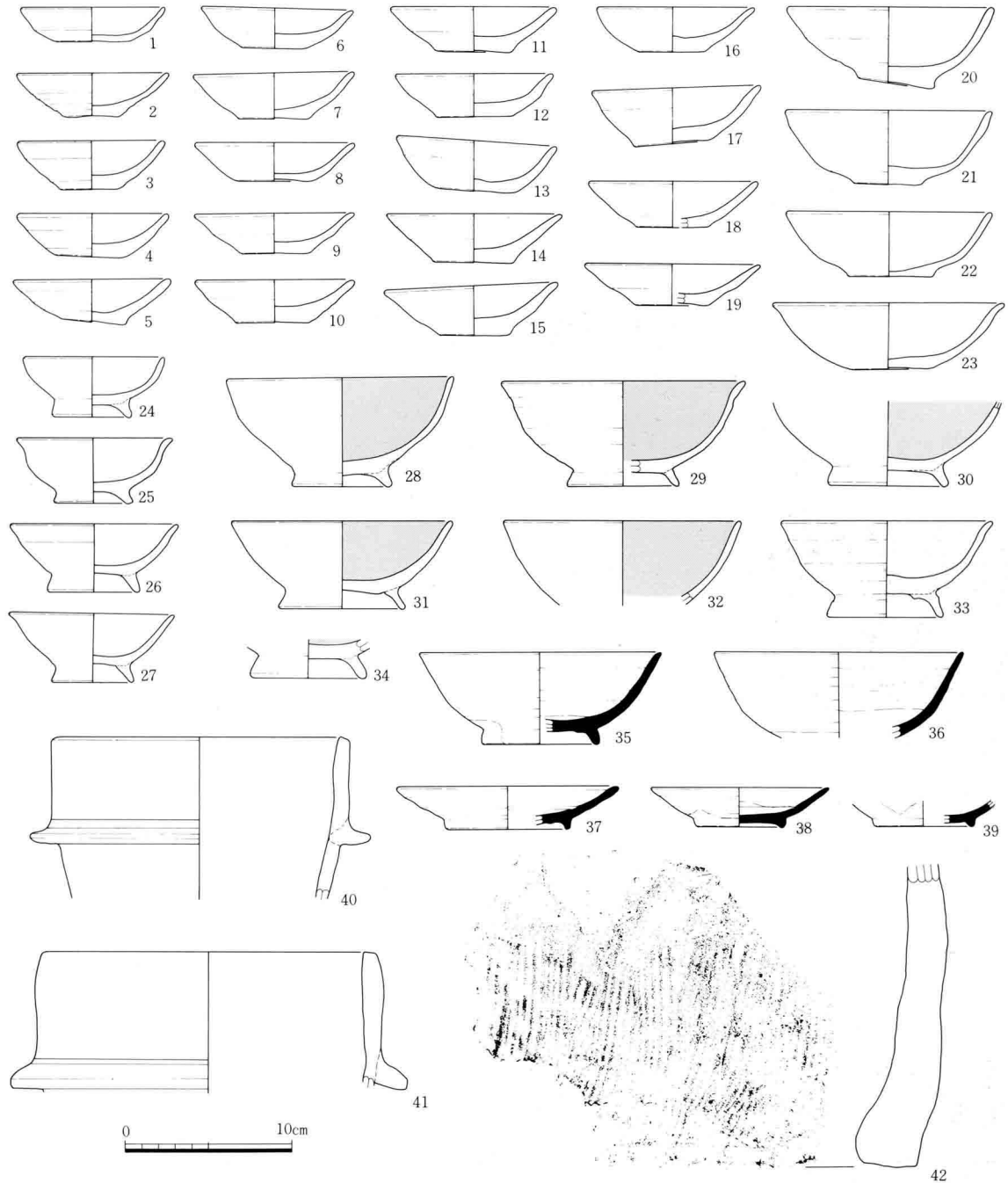
III-194 B17号住居址出土土器実測図
