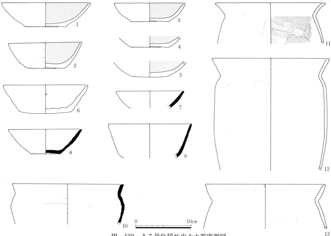
III-132 A 7号住居址出土土器実測図
