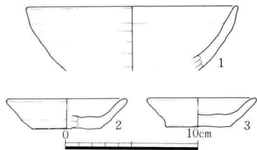
Ⅲ-151 B 1 号住居址出土土器実測図
