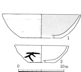
III-189 B16号住居址出土土器实测图
