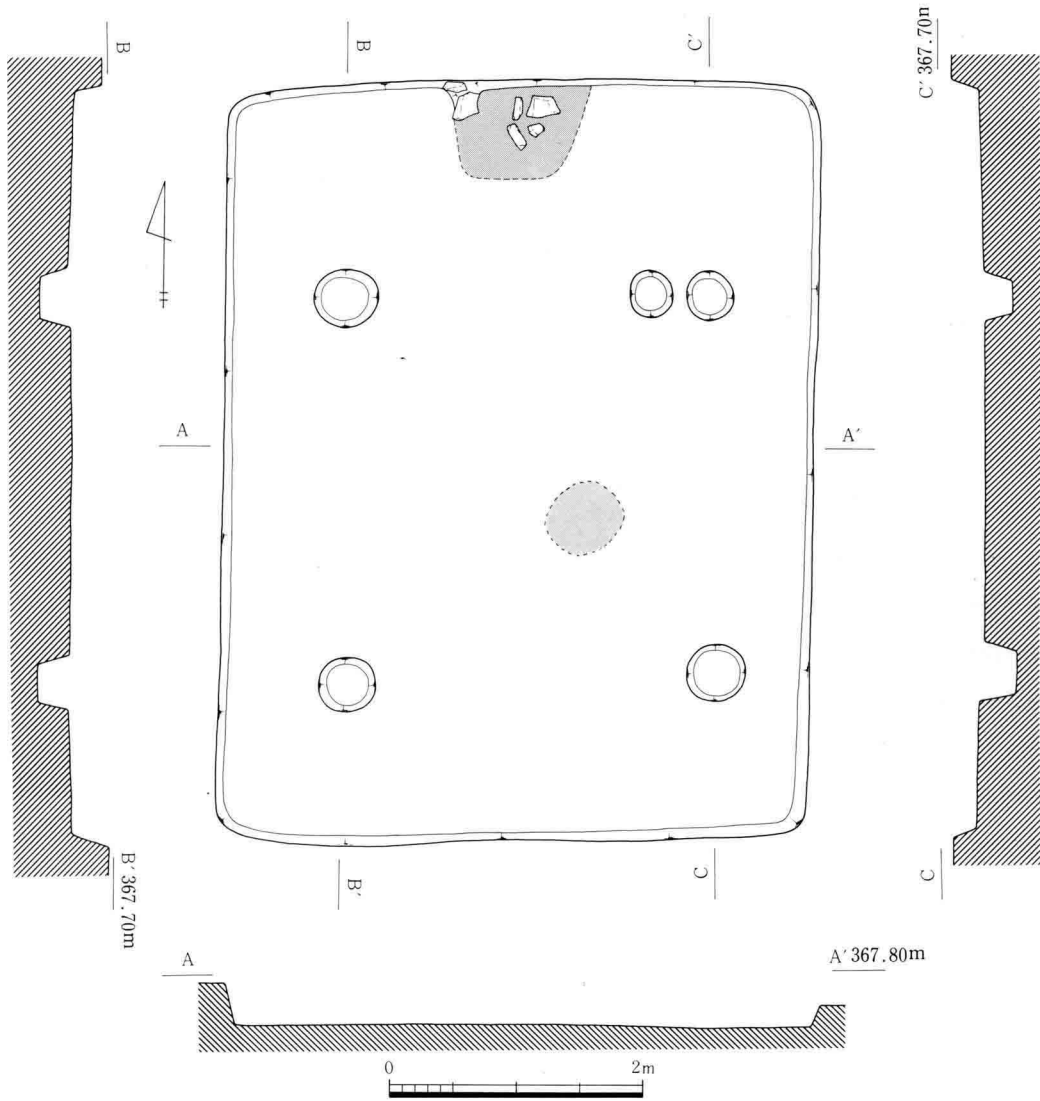
III-139 A20号住居址实测图
