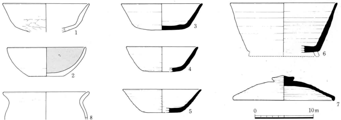
III-148 A22号住居址出土土器実測図
