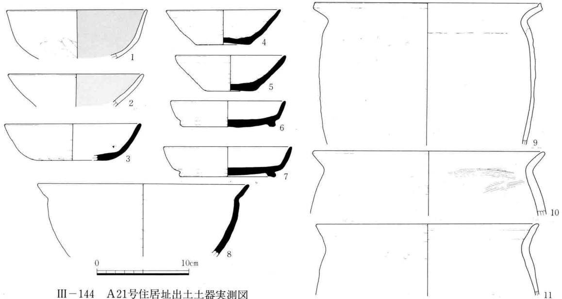
III-144 A21号住居址出土土器実測図
