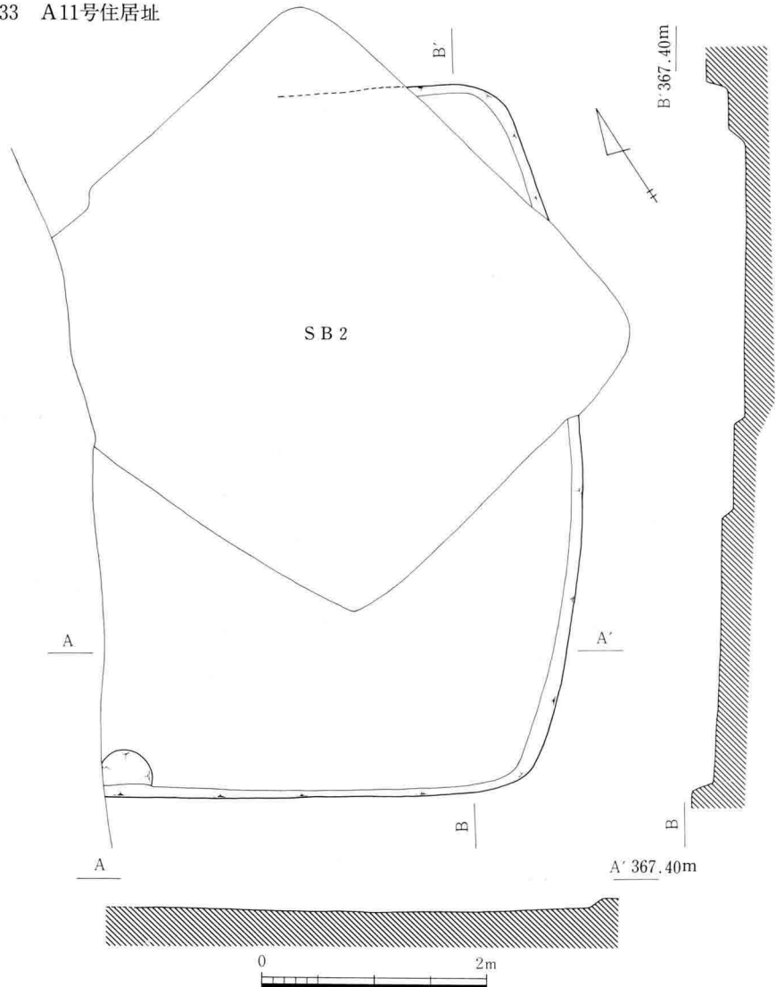
III-135 A13号住居址実測図
