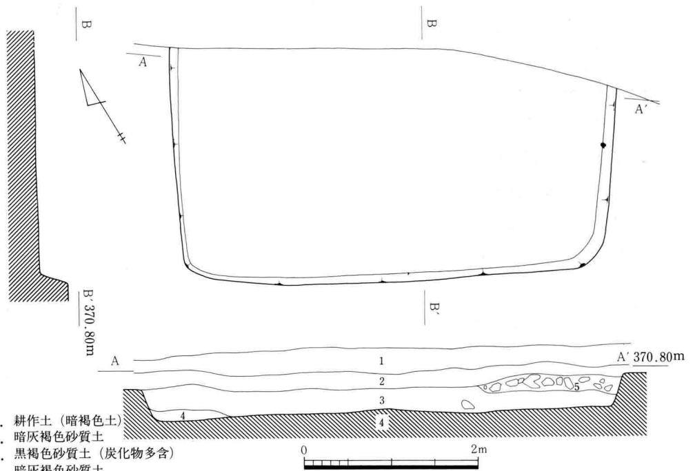
III-175 B11号住居址実測図
