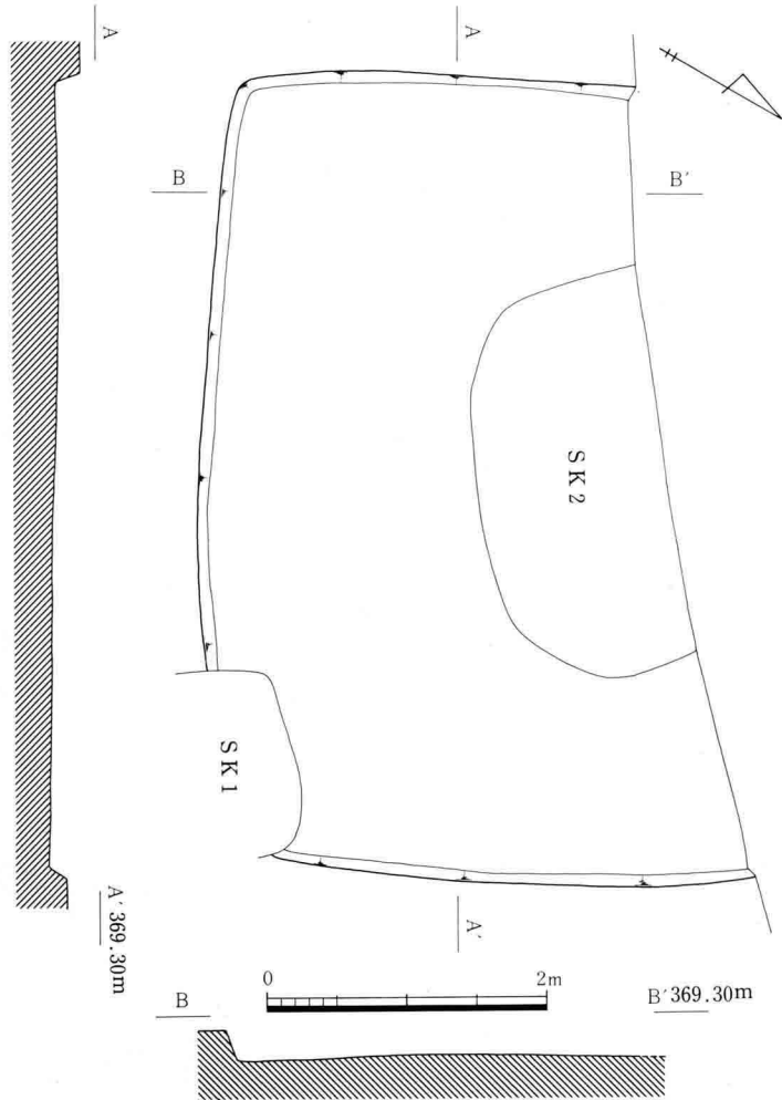
Ⅲ-152 B 2 号住居址実測図
