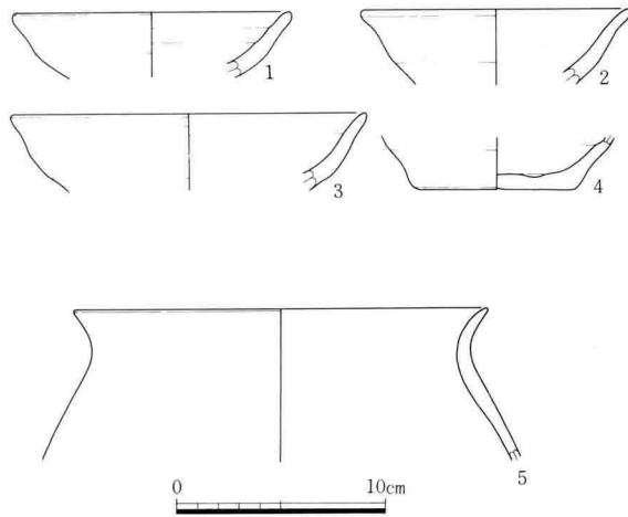
III-123 A 3号住居址出土土器実測図
