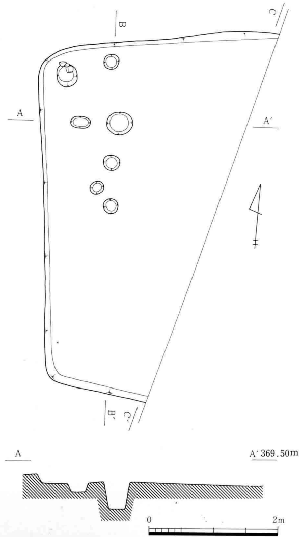
III-156 B 3号住居址実測図
