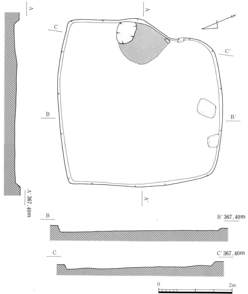
III-126 A 5号住居址実測図
