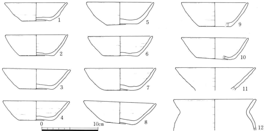
III-198 B19号住居址出土土器実測図
