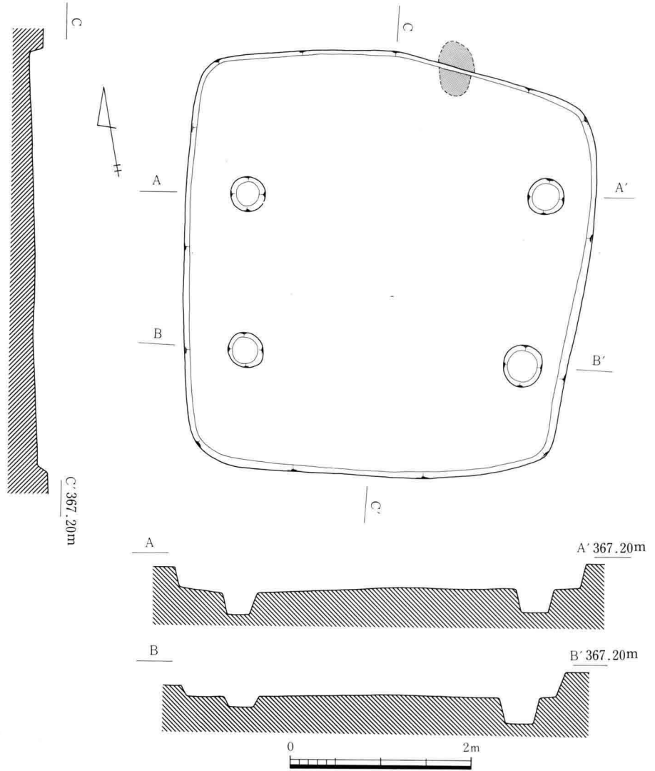
III-137 A17号住居址実測図
