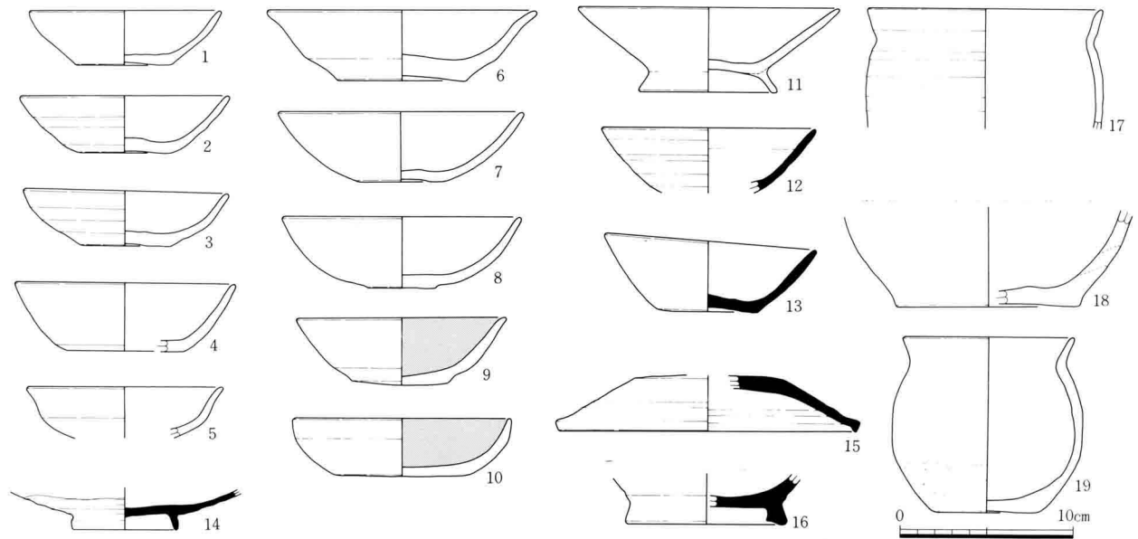
III-173 B10号住居址出土土器実測図
