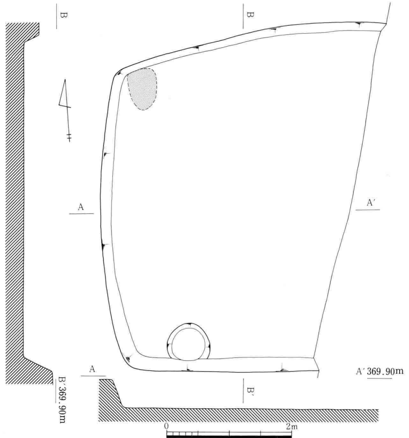
III-201 B22号住居址実測図
