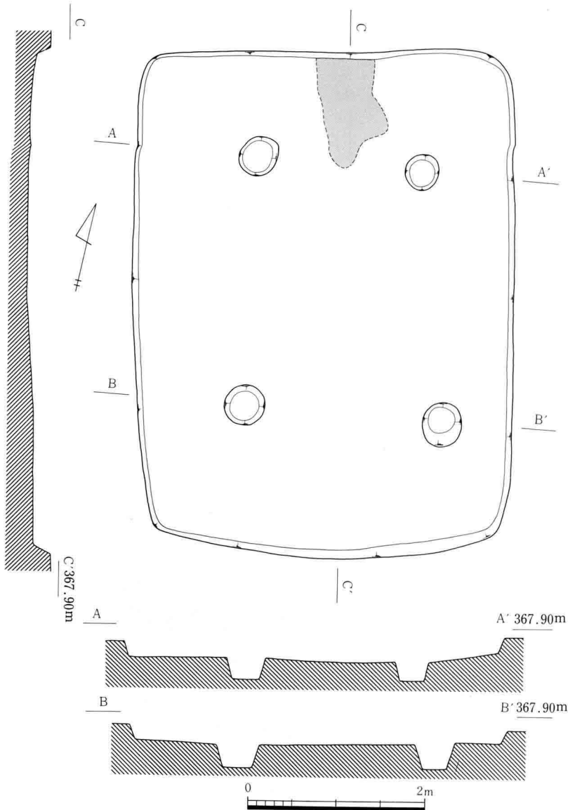
III-142 A21号住居址実測図
