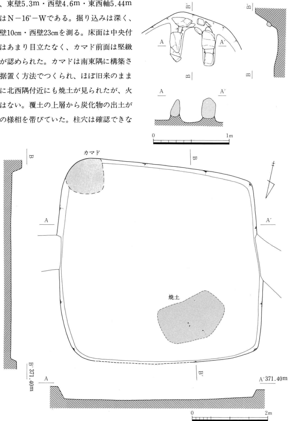
III-204 B26号住居址・カマド実測図
