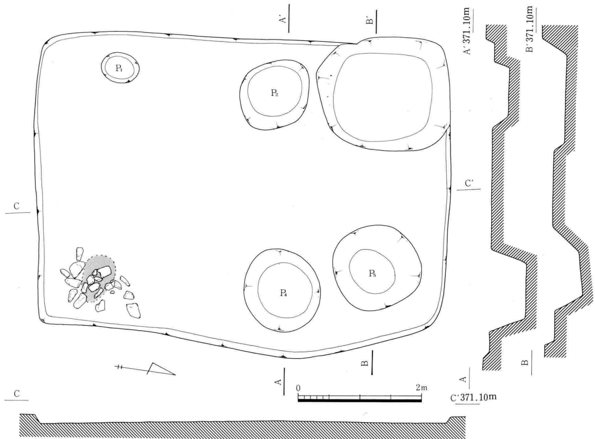
III-191 B17号住居址実測図
