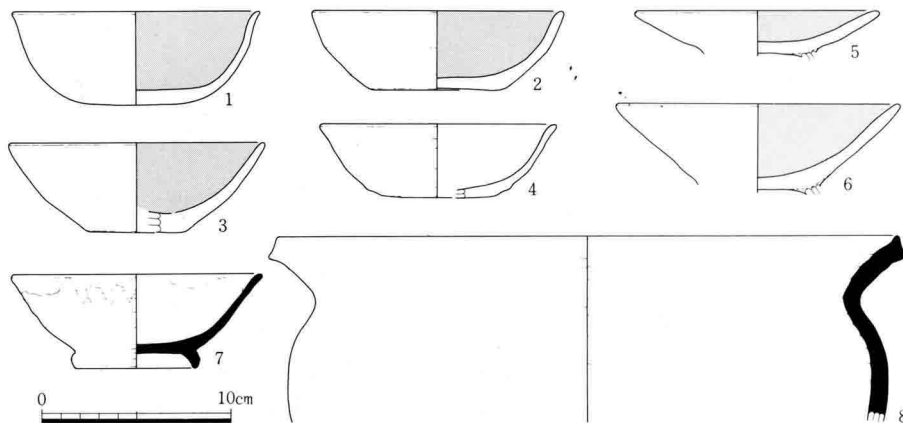
III-196 B18号住居址出土土器実測図
