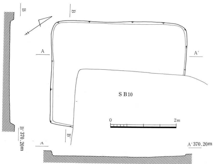
III-190 B16号住居址实测图
