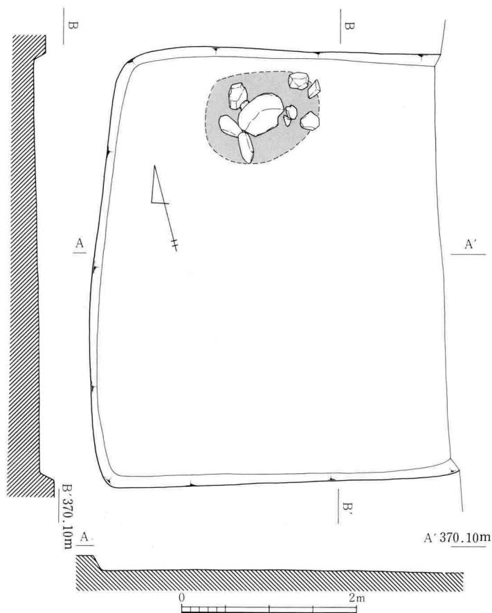
III-209 B27号住居址实测图
