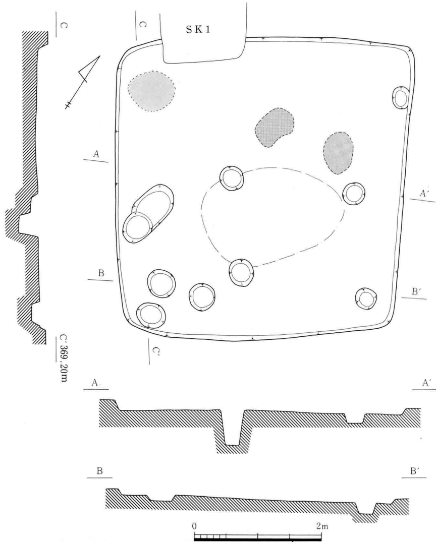
III-149 B1号住居址実測図
