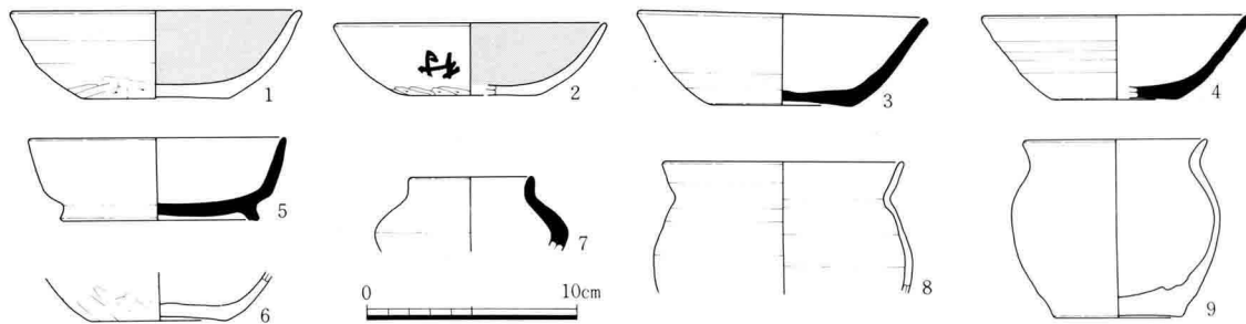
III-141 A20号住居址出土土器実測図
