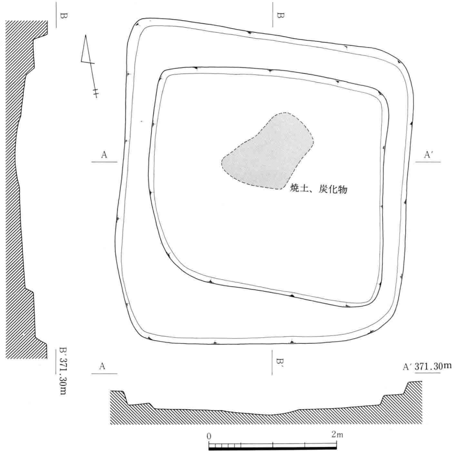
III-178 B12号住居址実測図
