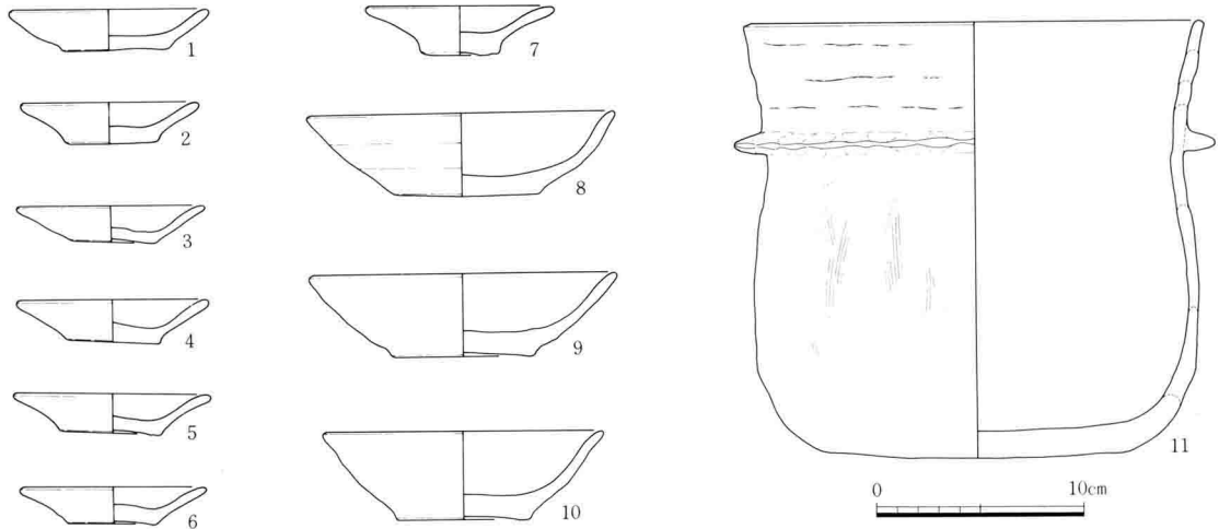
III-171 B9号住居址出土土器実測図
