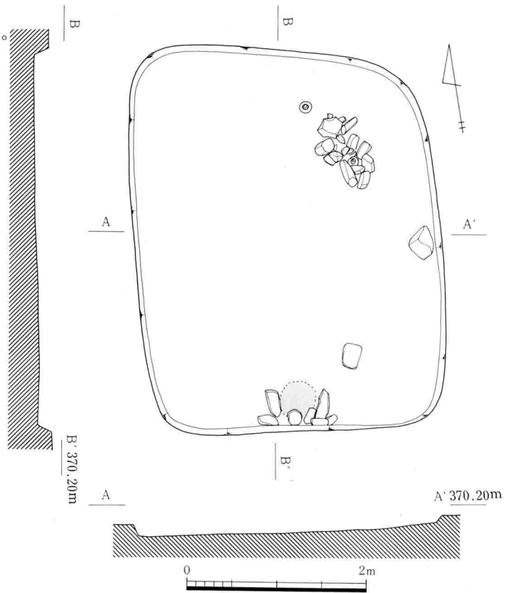
III-185 B15号住居址実測図
