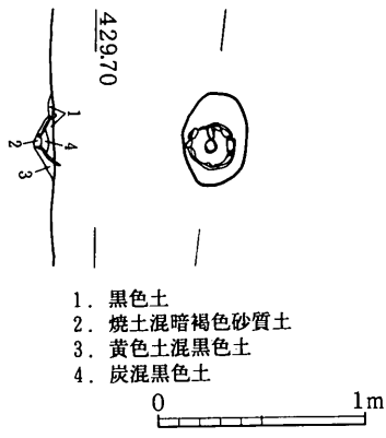
SB 283 炉
