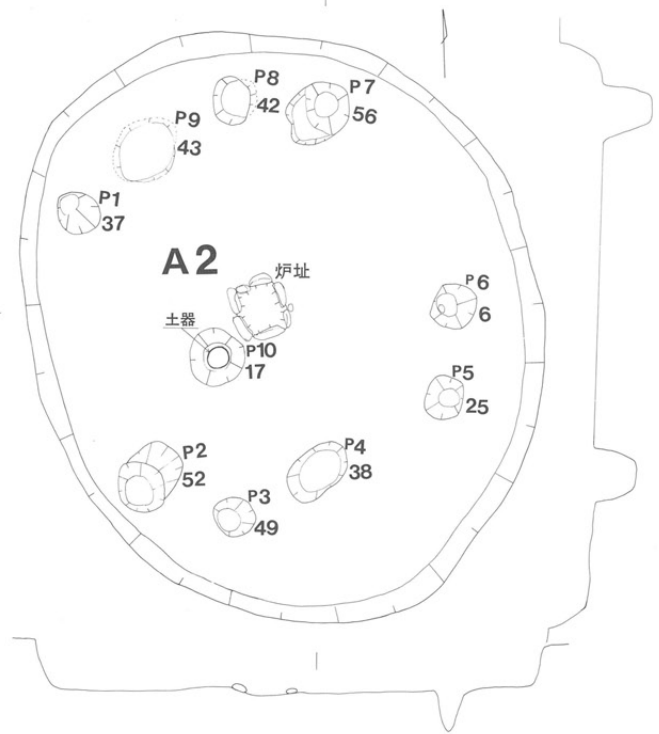
第 5 図 A 2 号住居址 (1 : 60)
