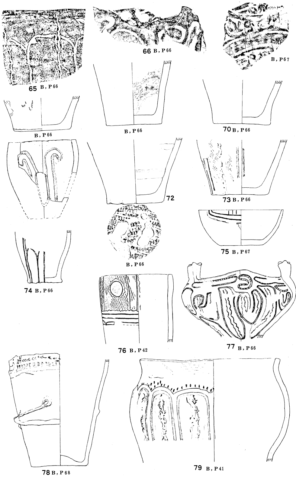
第19图 土器实测图(1:4)
