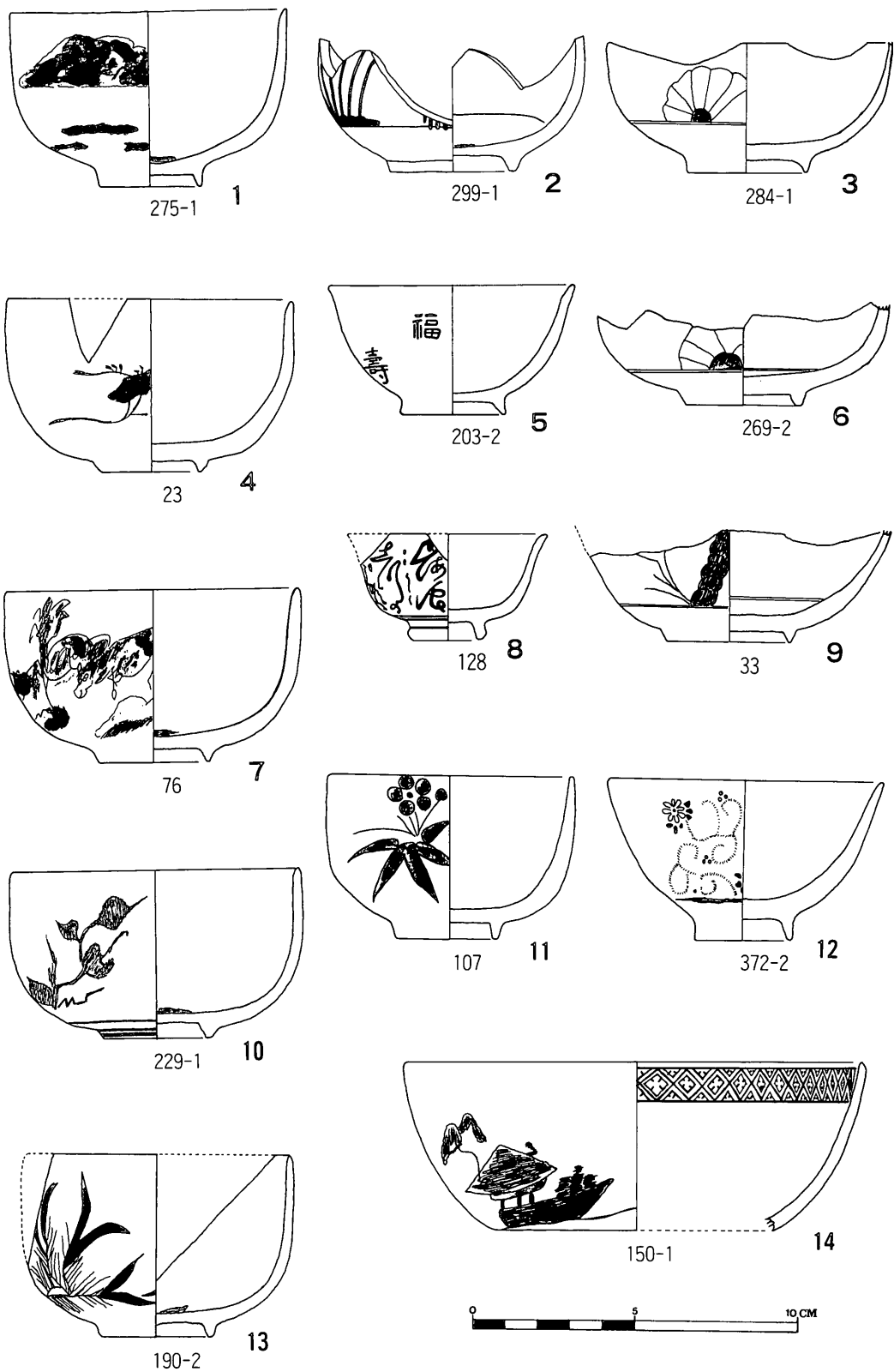
第10図 高遠城跡出土遺物実測図(1)
