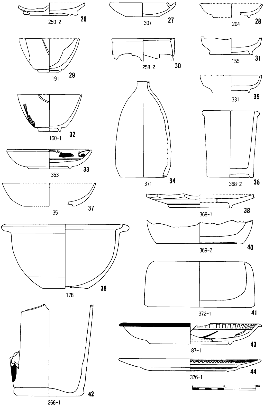
第12图 高遠城跡出土遺物実測図(3)
