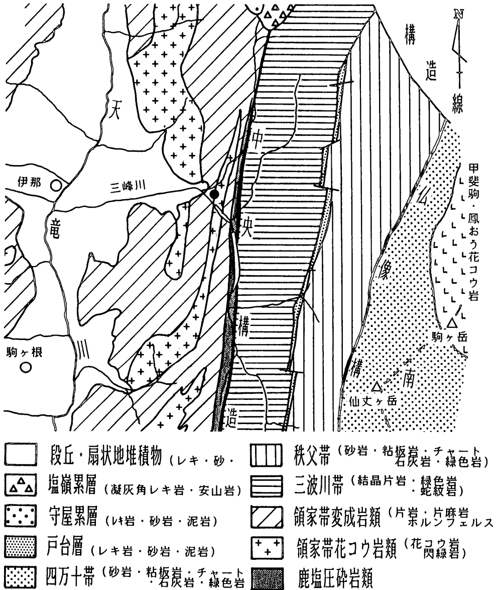
第4図 高遠城跡地質概界図
