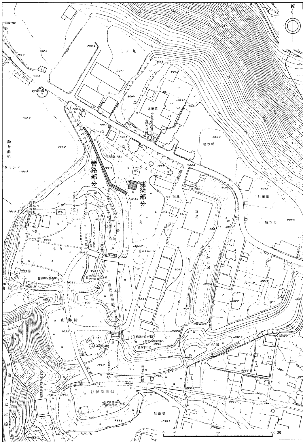
第3図 高遠城跡発掘調査箇所位置図
