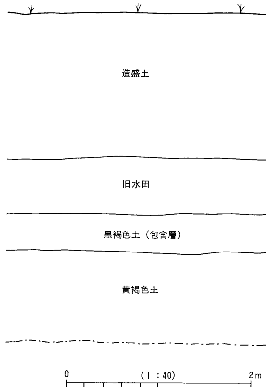
第16図 更埴条里水田址土層断面図
