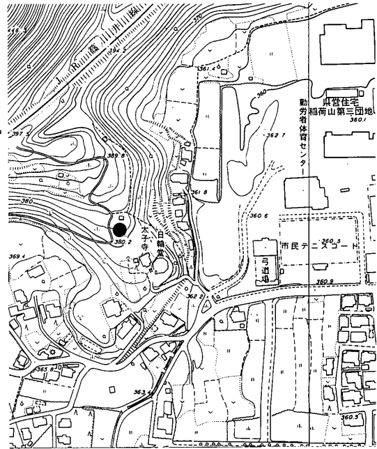
第22図 湯ノ崎遺跡調査位置図
