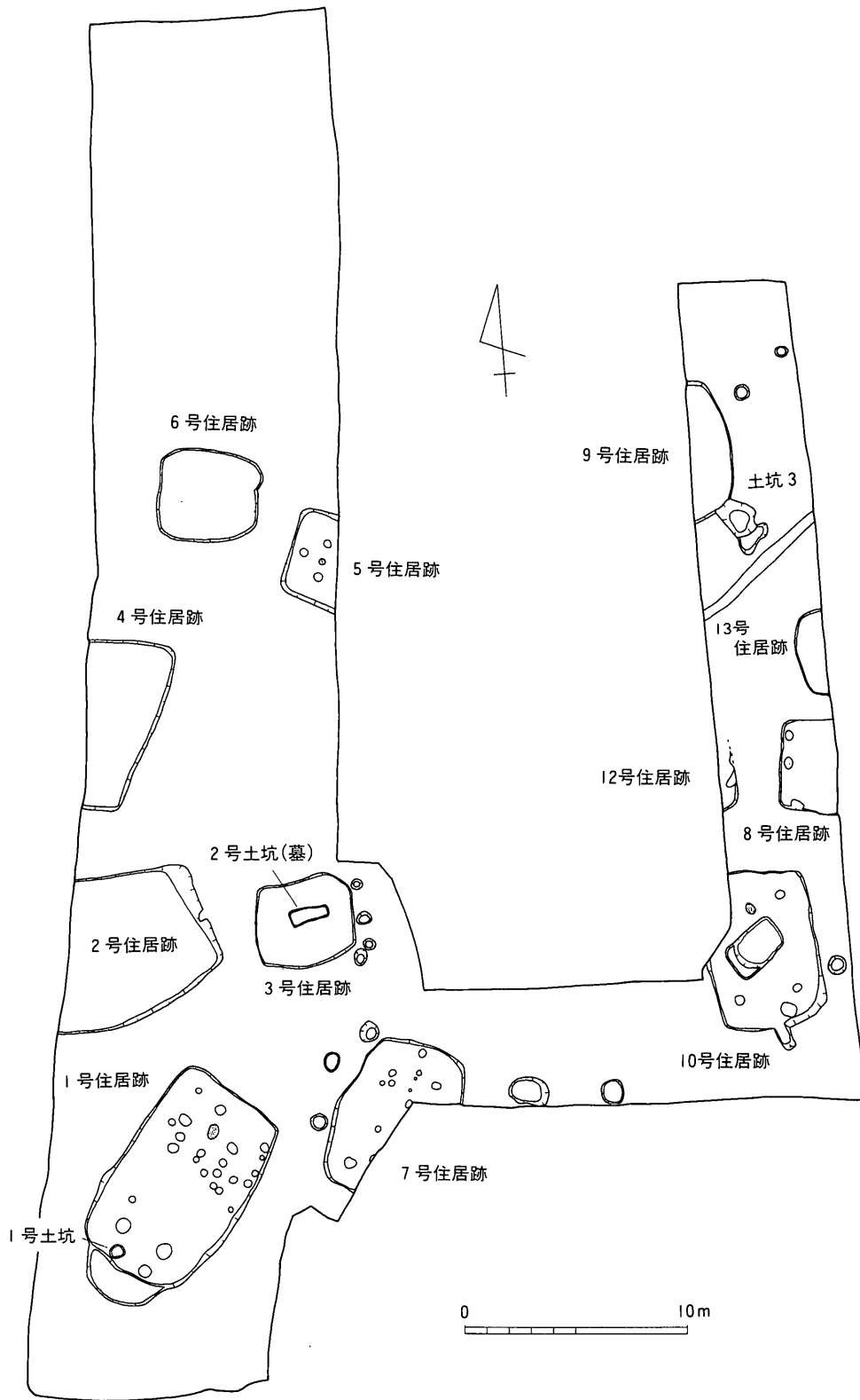
第21图 南棄水遺跡全体图
