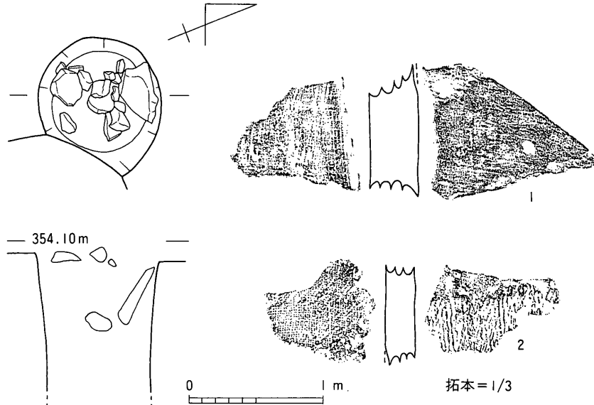
第29図 大宮遺跡3号土坑及び出土遺物
