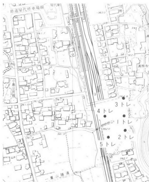
第37図 屋代城跡位置図
