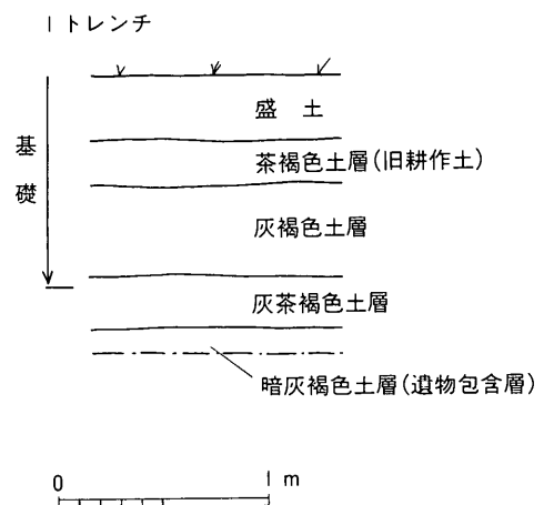
第40図 唐崎遺跡土層断面図
