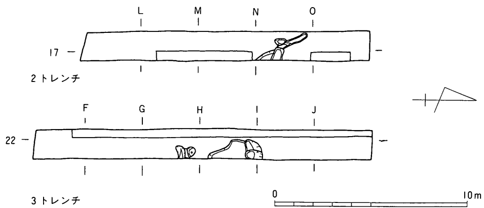
第10図 遺構全体図1
