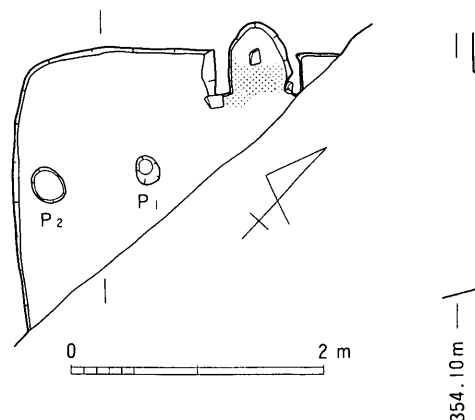
第27図 大宮遺跡1号住居跡
