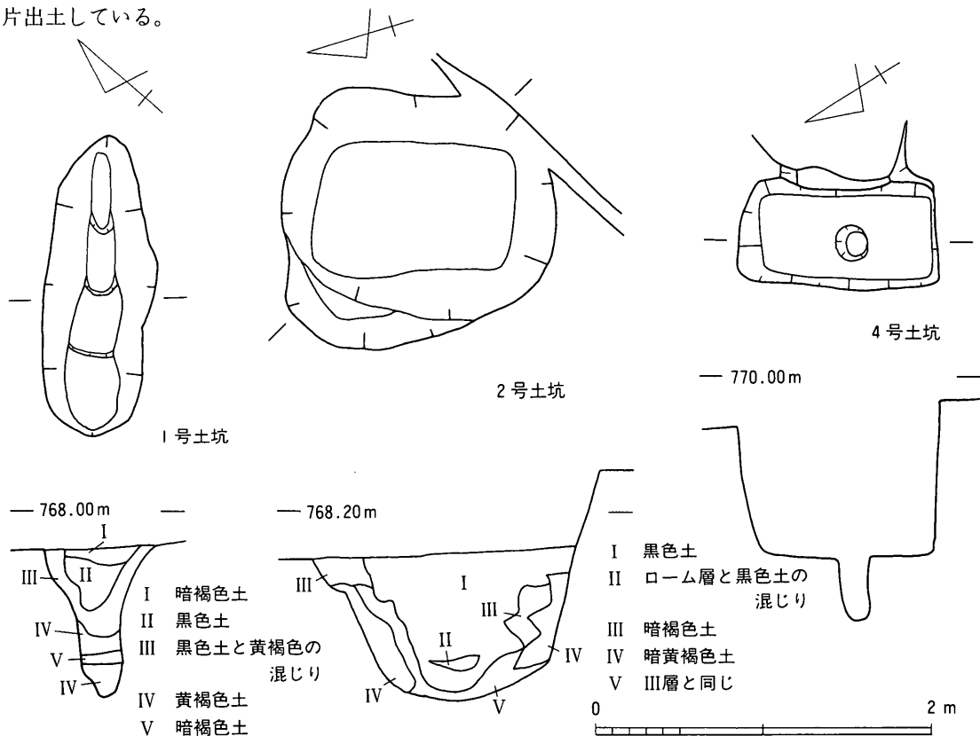
第12図 池尻遺跡1・2・4号土坑
