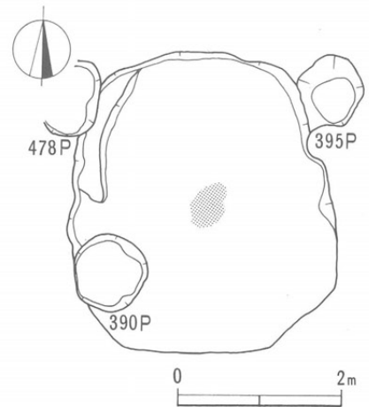
第61図 6号住居跡平面図 (1:80)
