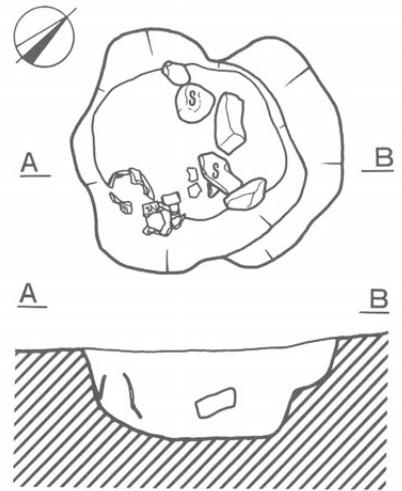
第74図 532P 平・断面図 (1:30)
