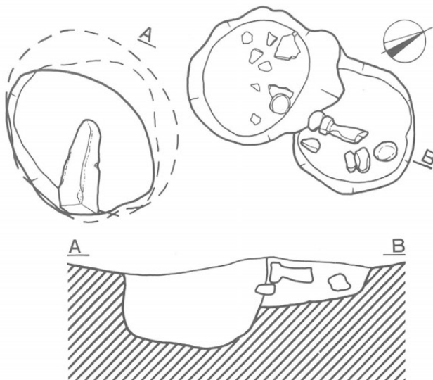
第69図 476P・477P 平・断面図 (1:30)
