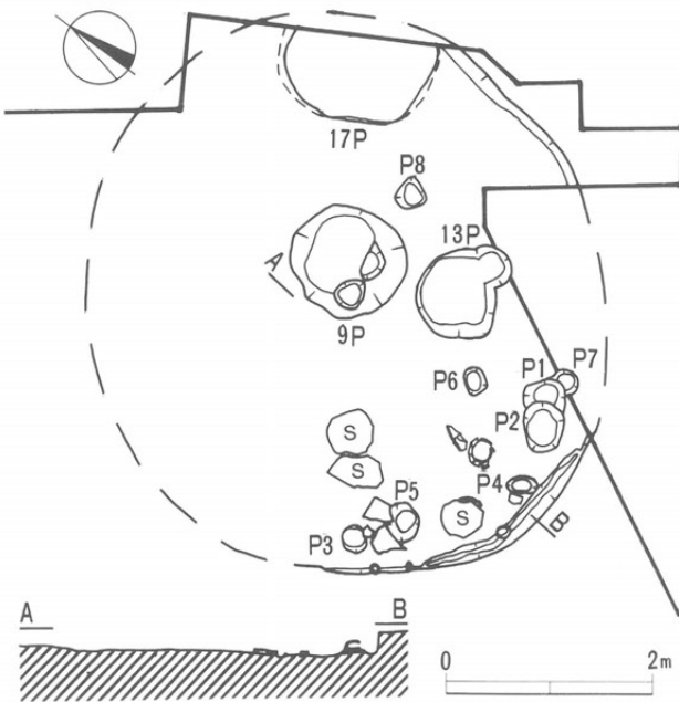
第25図 16号住居跡平面図 (1:80)
