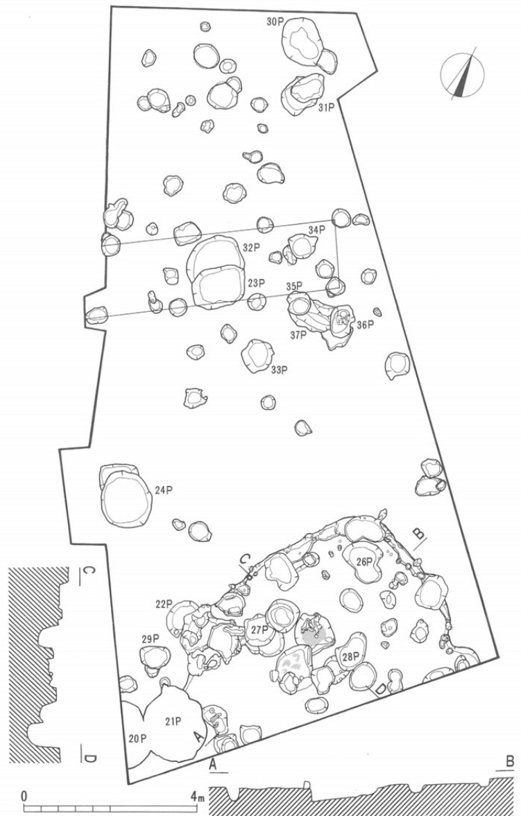
第47図 長塚遺跡遺構全体図 (1 : 120)
