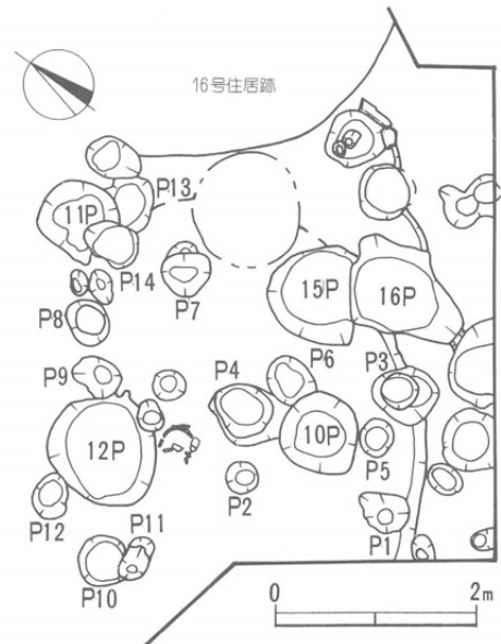
第29図 21号住居跡平面図 (1:80)
