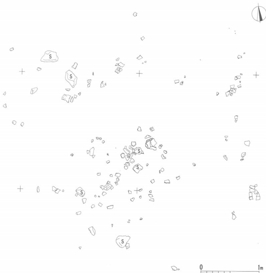
第53図 包含層遺物出土状態 (1 : 40)
