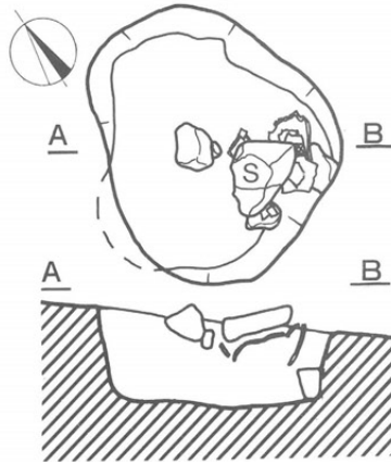
第75図 536P 平・断面図 (1:30)
