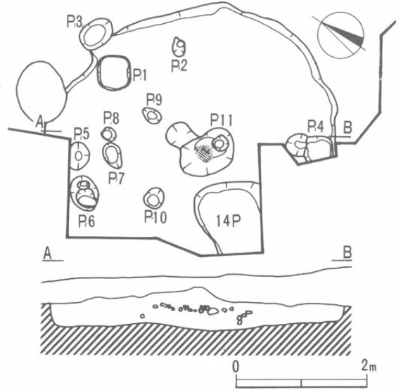
第23図 15号住居跡平面図 (1:80)
