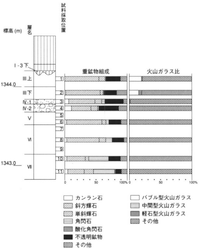
図14 1d区27グリッド南壁深掘地点の重鉱物組成および火山ガラス比
