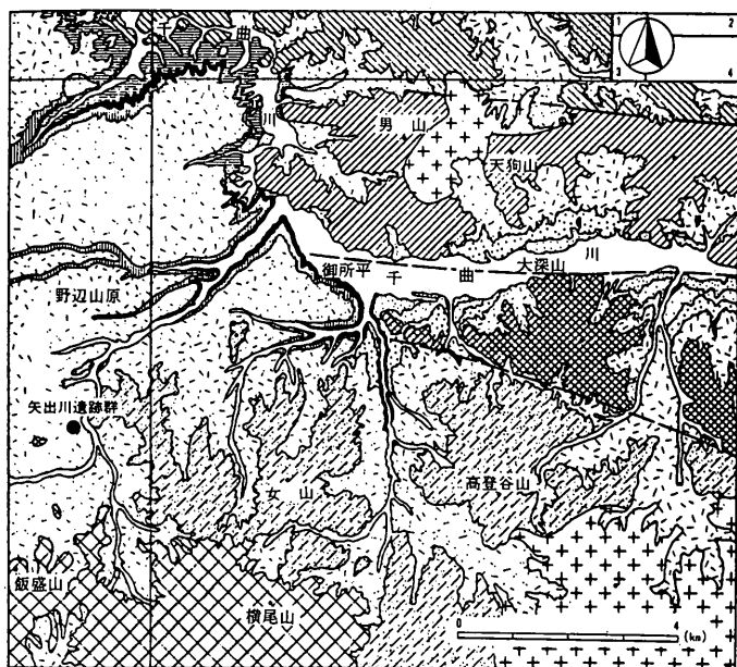
1: 沖積層 2: 小川口面 3: 馬場平面 4: 秋山原面 5: 野辺山原面(2-5: 段丘堆積物) 6: 野辺山原層上部 7: 野辺山原層中部 8: 野辺山原層下部および本沢溶岩・スコリア 9: 高石川層 10: 海の口火砕岩 11: 飯盛山火山岩類 12: 石英閃緑岩類 13: 高登谷山層群 14: 川上層群 15: 合羽坂層群 16: 天狗山層群 17: 地送り堆積物 18: (推定)断層 なお、右肩枠内の数字は対応する図幅名、1: 穂科山、2: 十石峠、3: 八ヶ岳、4: 金峯山
