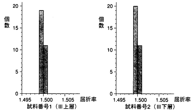
図15 火山ガラスの屈折率
