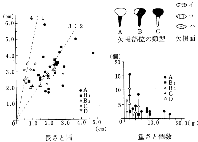
図165 石錐法量相関
