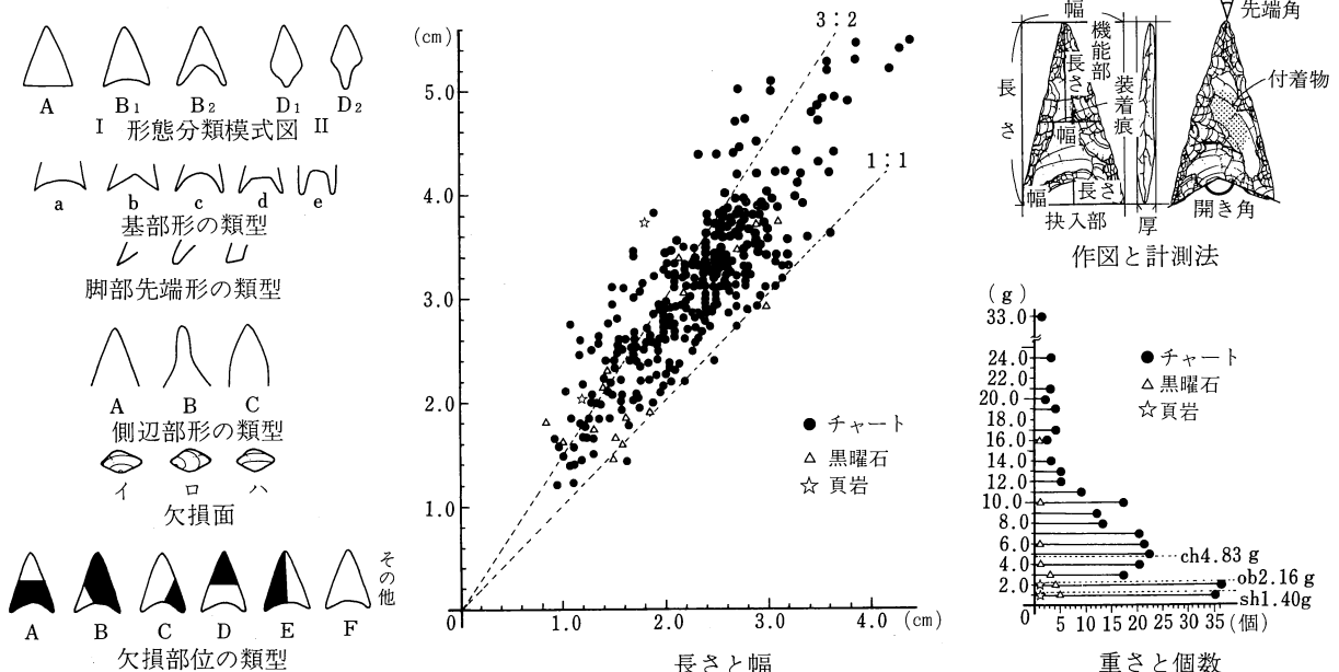
図152 石鏃法量相関(材質別)
