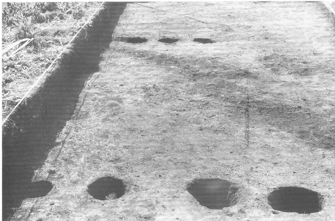
写真17 柱 穴
