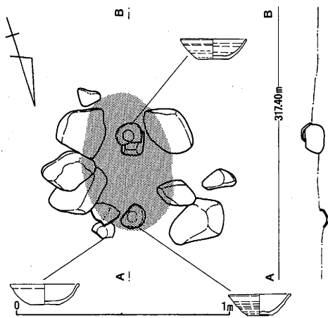
図6 H19号住居址カマド実測図 (1:20)
