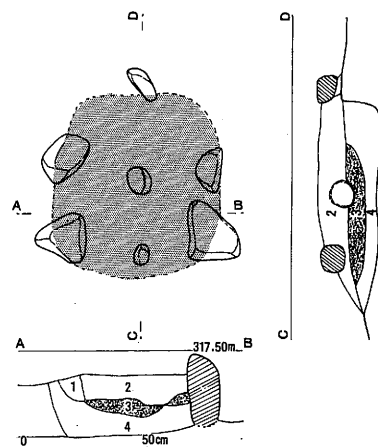
図8 H20号住居址カマド断面図 (1:30)
