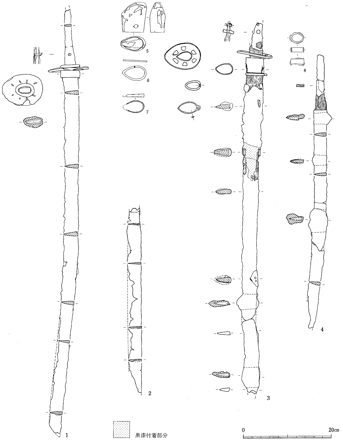
第51図 金属製品(1) 直刀(1~4) 刀装具(5~8)
