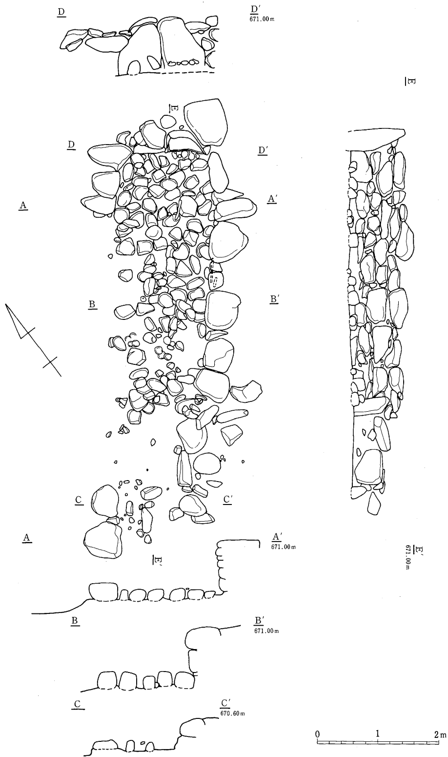
第41图 南方古墳石室平面図及び断面図
