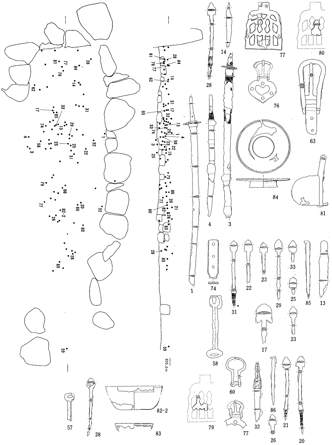
第45図 石室内金属製品出土状況
