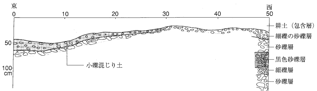
第3図 Aトレンチ土層断面図（木船清氏実測）
