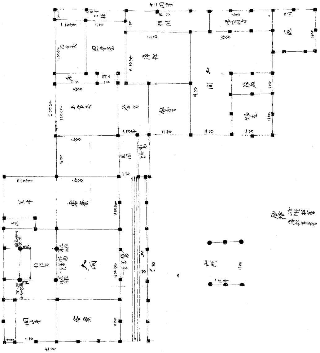
第22圖 長尾組榎村龍峰寺燒失跡礎墨引 (明治元年)
