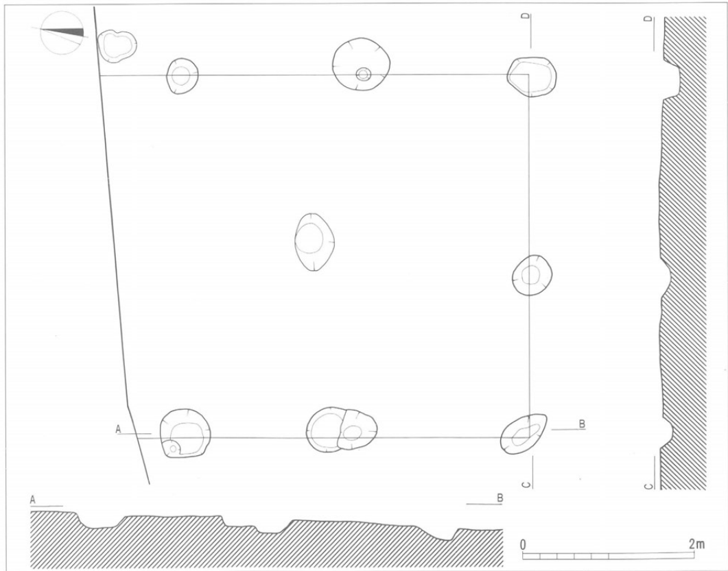
第14図 山道端地籍掘立柱建物跡 (1:60)
