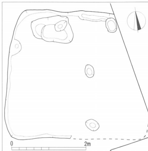
第8図 山道端地籍31号住居跡 (1:60)
