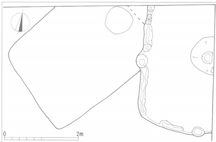
第3図 山道端地籍29・33号住居跡 (1:60)
