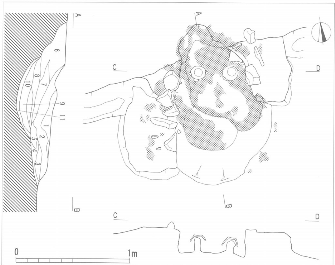
第27図 榎垣外遺跡十王堂地籍1号住居跡カマド平面図 (1:20)
