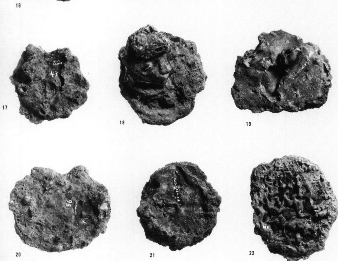
左16羽口付着椀型滓アツブ
