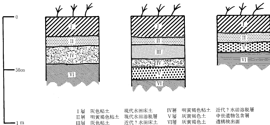
基本土層模式図
