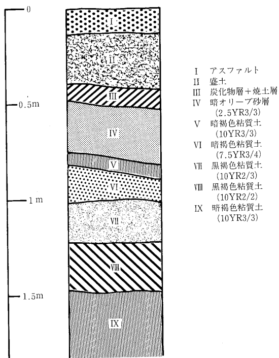
基本土層模式図
