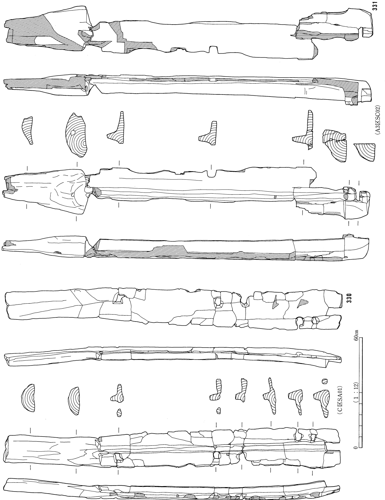
木製品64 (建築部材 楣・蹴放材)
