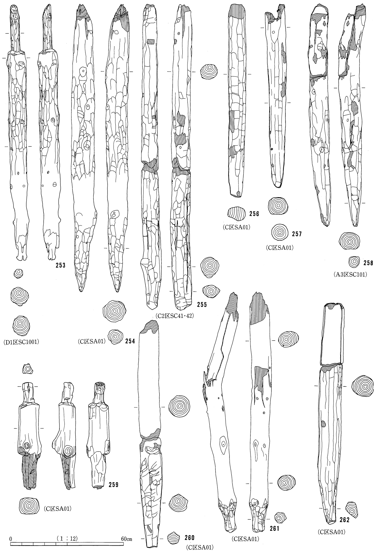
木製品43 (建築部材 縦材)
