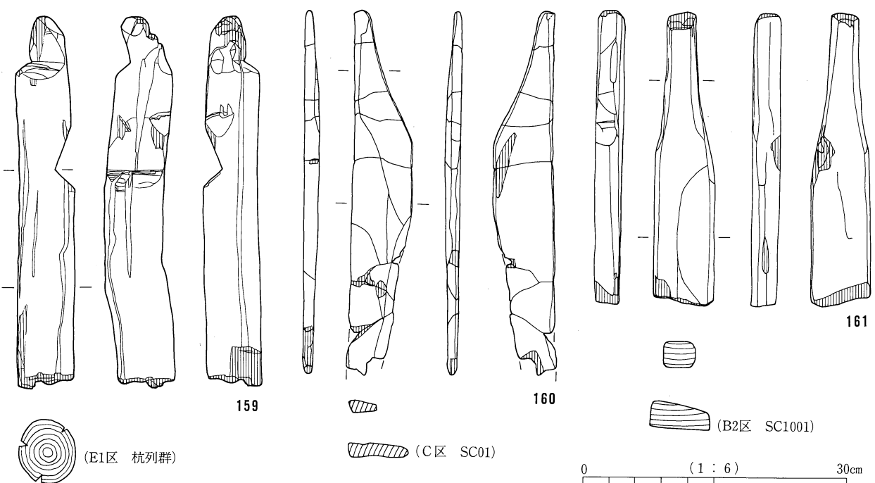
木製品28 (棒状木製品)
