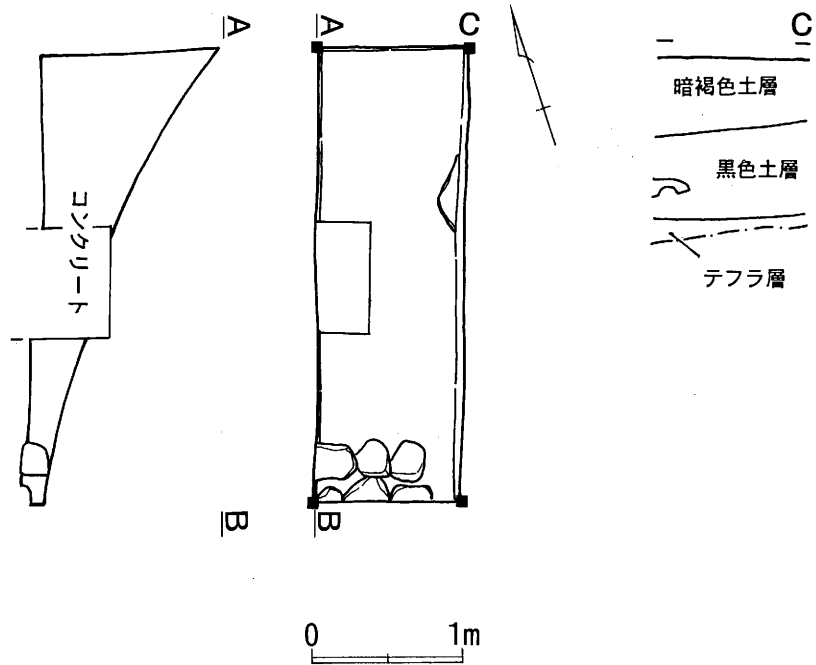
図8 本丸D・Eトレンチ平面図 (1:50)
