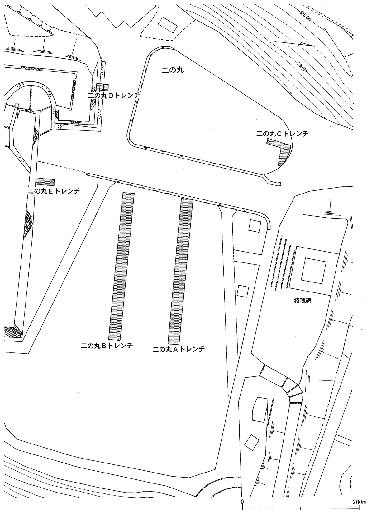
図11 二の丸トレンチ位置図 (1 : 400)
