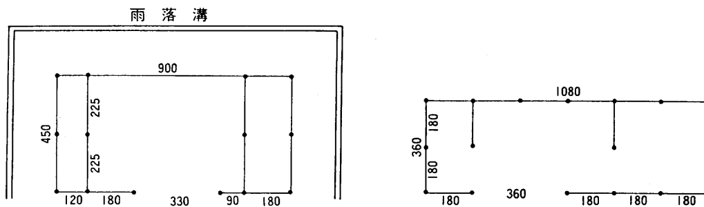
図3 南中門(左)及び駕籠部屋(右)規模模式図(1:200)単位はcm
