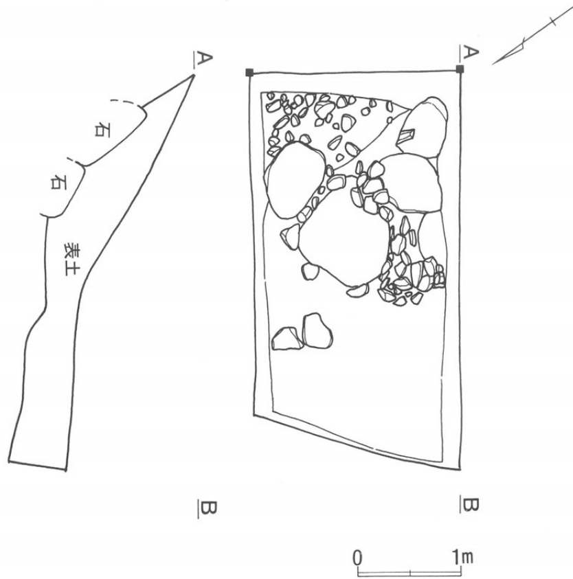
図10 帯曲輪Aトレンチ平面図 (1 : 50)
