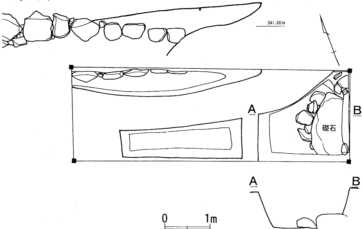
図9 本丸F・Gトレンチ平面図 (1:50)
