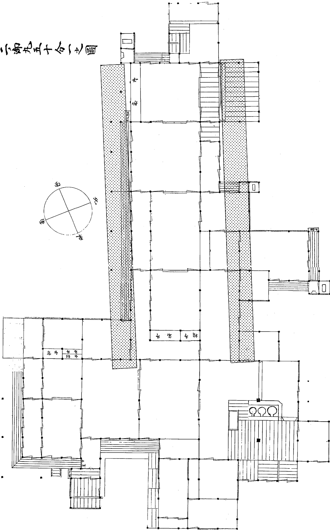
図13 二の丸御殿間取り図及びトレンチ設定対照図 (1:200)
