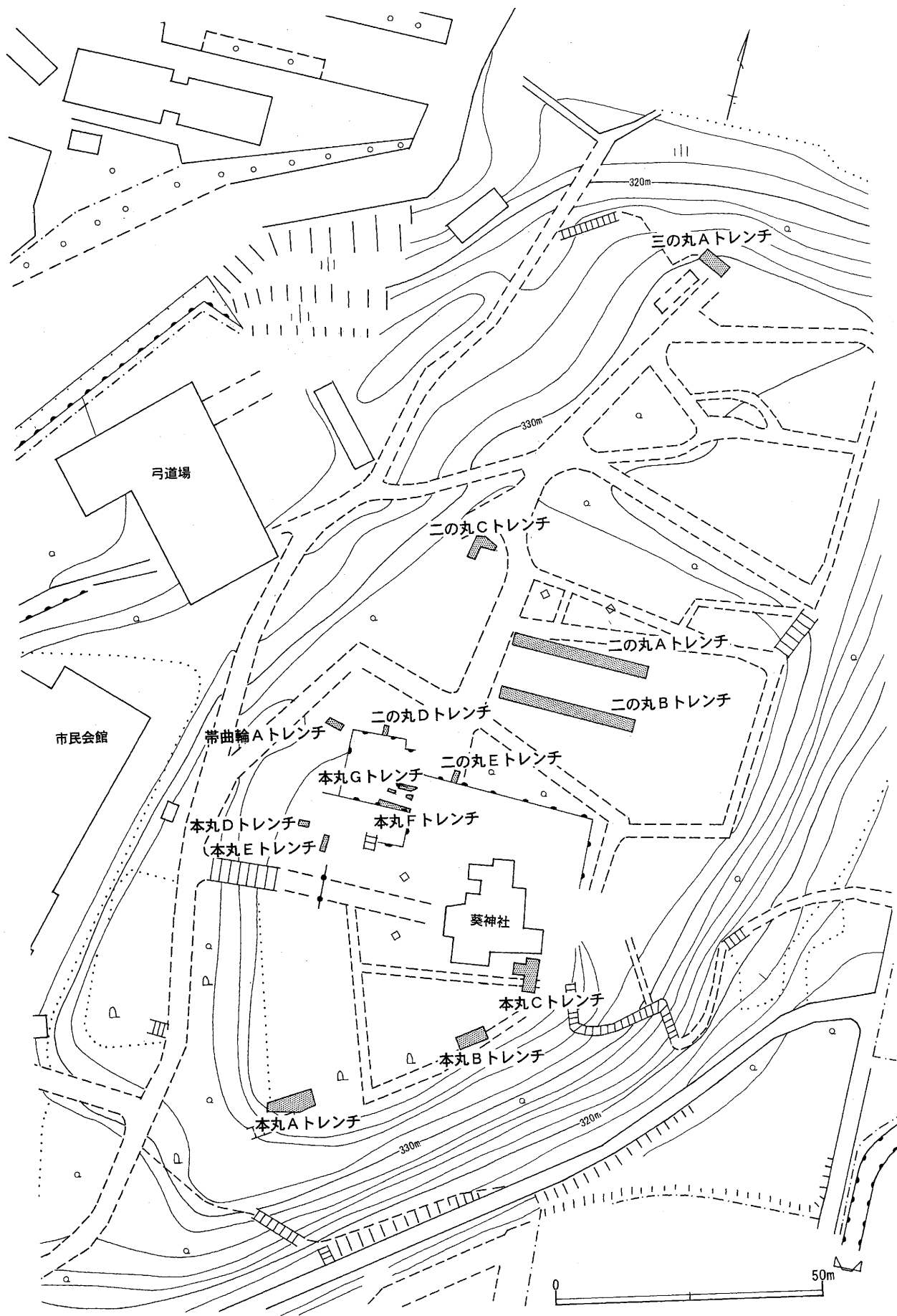
図4 調査区位置図 (1:1000)
