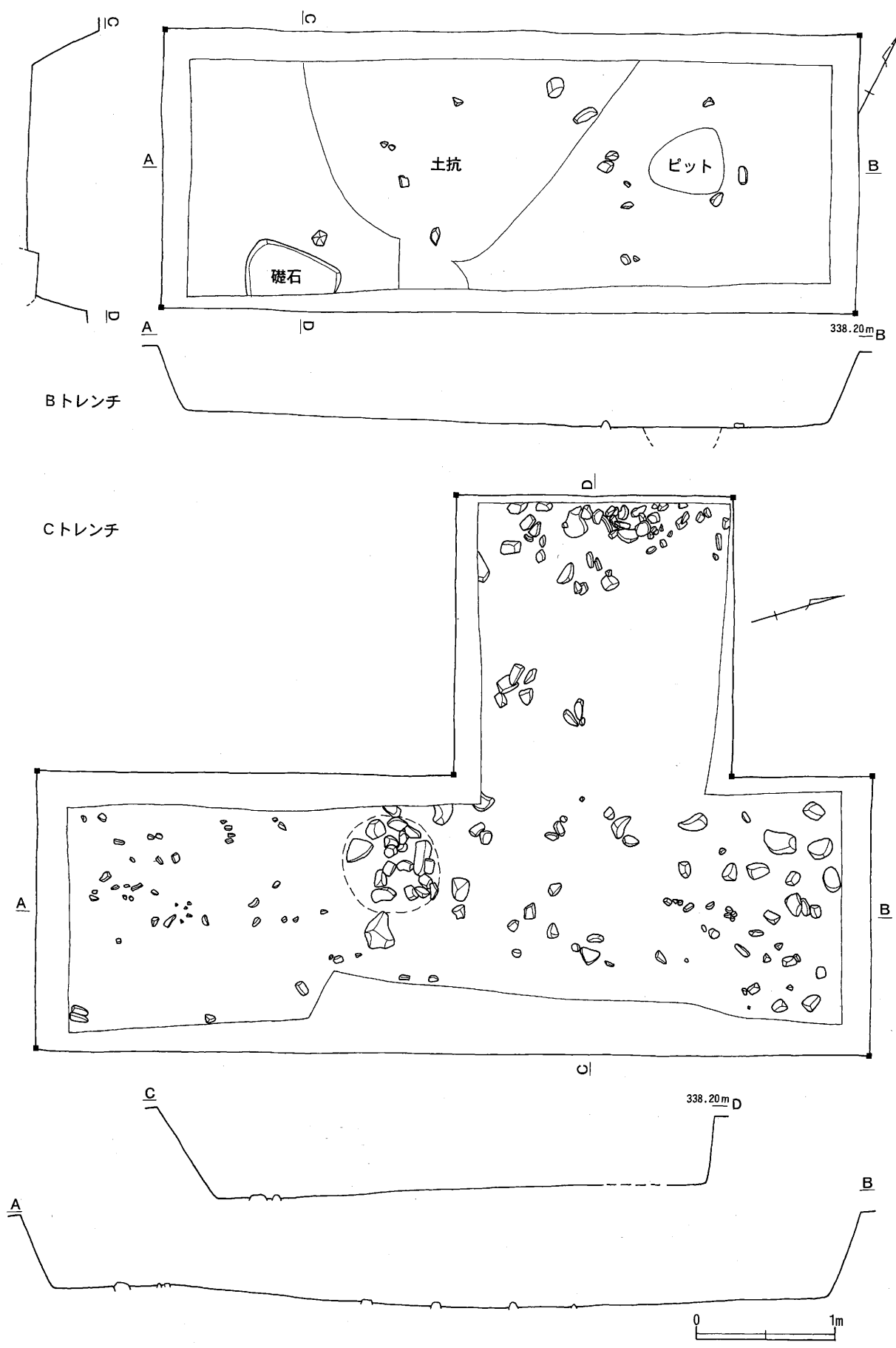
図7 本丸B・Cトレンチ平面図 (1:40)
