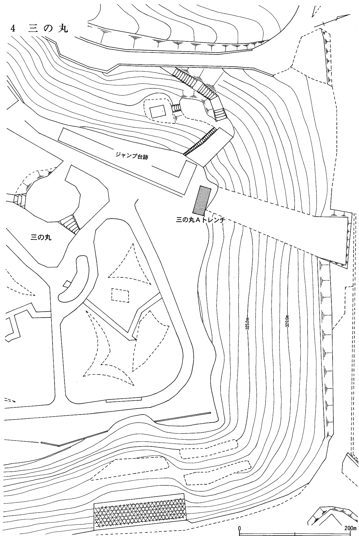
図17 三の丸トレンチ位置図 (1 : 400)
