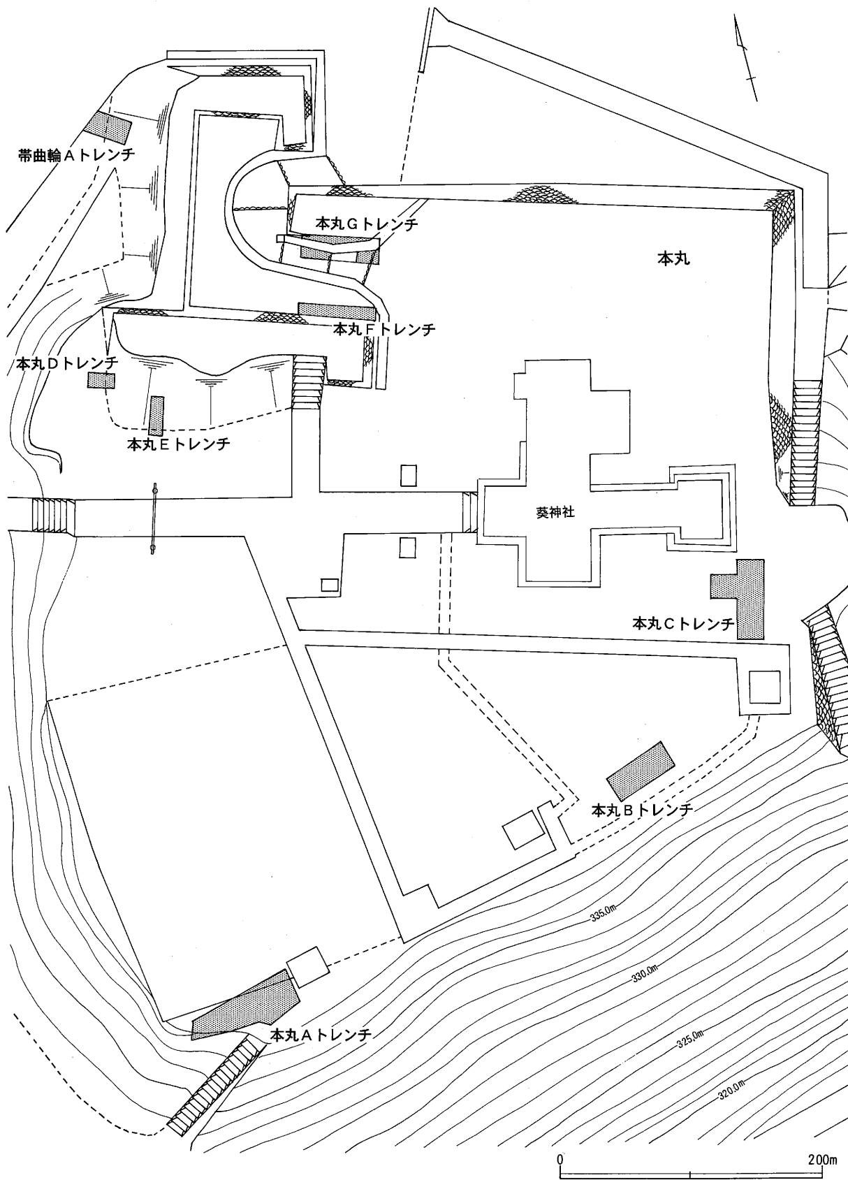
図5 本丸・帯曲輪トレンチ位置図 (1:400)
