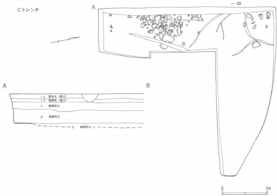
図14 二の丸Cトレンチ平面図 (1:40)
