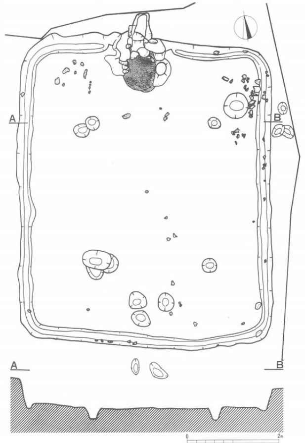
第78図 I号住居跡平面図(1:80)
