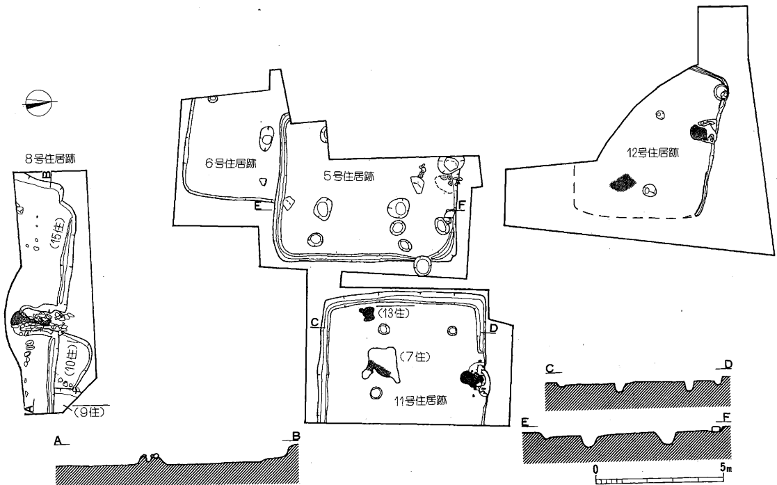
第19図 榎垣外遺跡遺構全体図(1:200)
