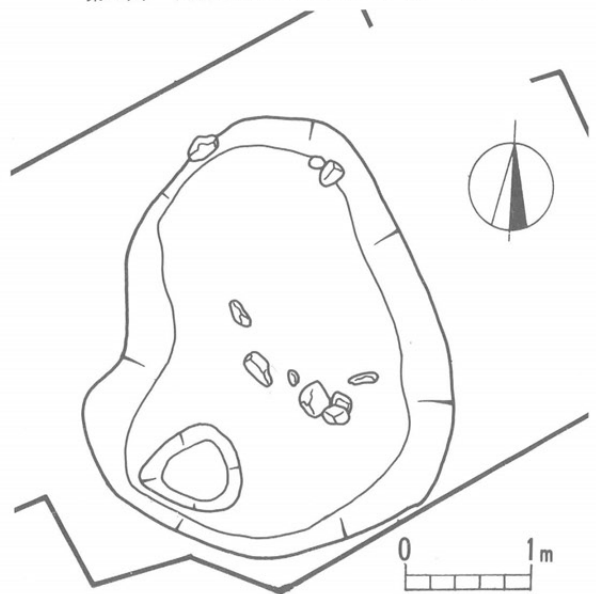
第82図 金山地籍2号住居跡平面図(1:60)
