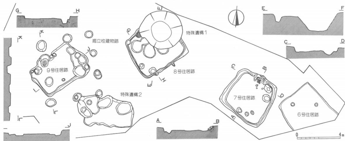
第74図 下片間町地籍 遺構全体図（1：200）
