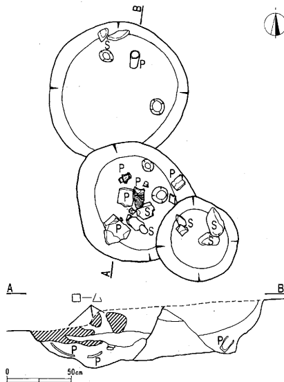
第41図 625P・626P 平・断面図
