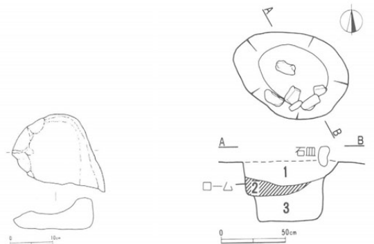
第34図 629P 平・断面図(左) 629P出土石皿(右)
