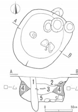
第54図 705 P 平・断面図
