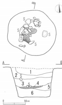
第35図 635 P 平・断面図
