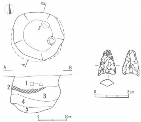
第52図 674 P 平・断面図(左)出土遺物(右)
