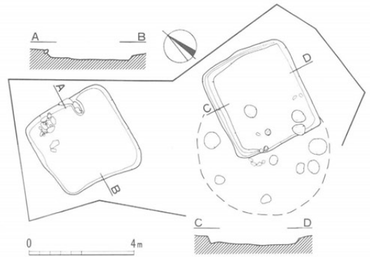
第81図 下片間丁地籍遺構全体図(1:200)
