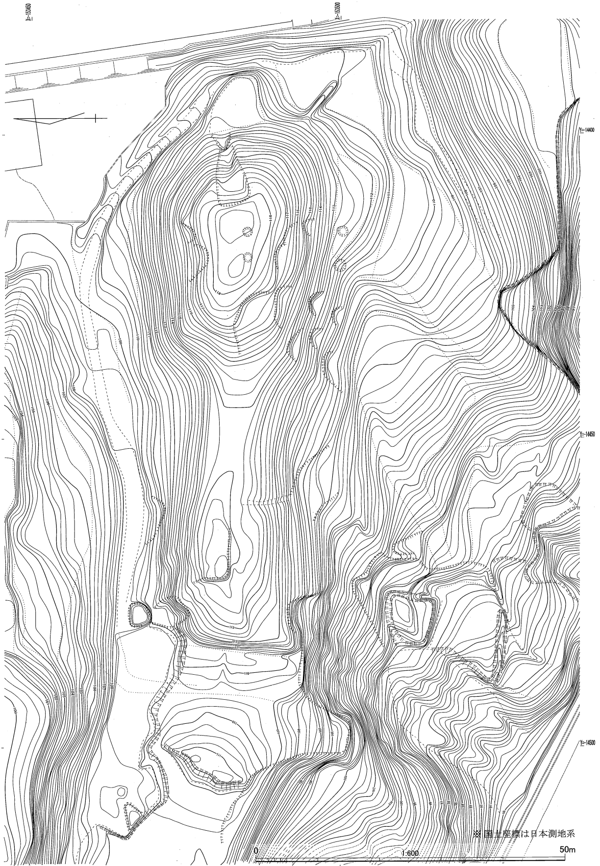
第4図 赤土山古墳測量図
