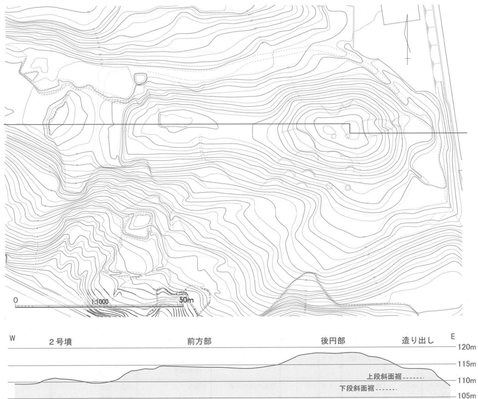
第15図 墳丘エレベーション図
