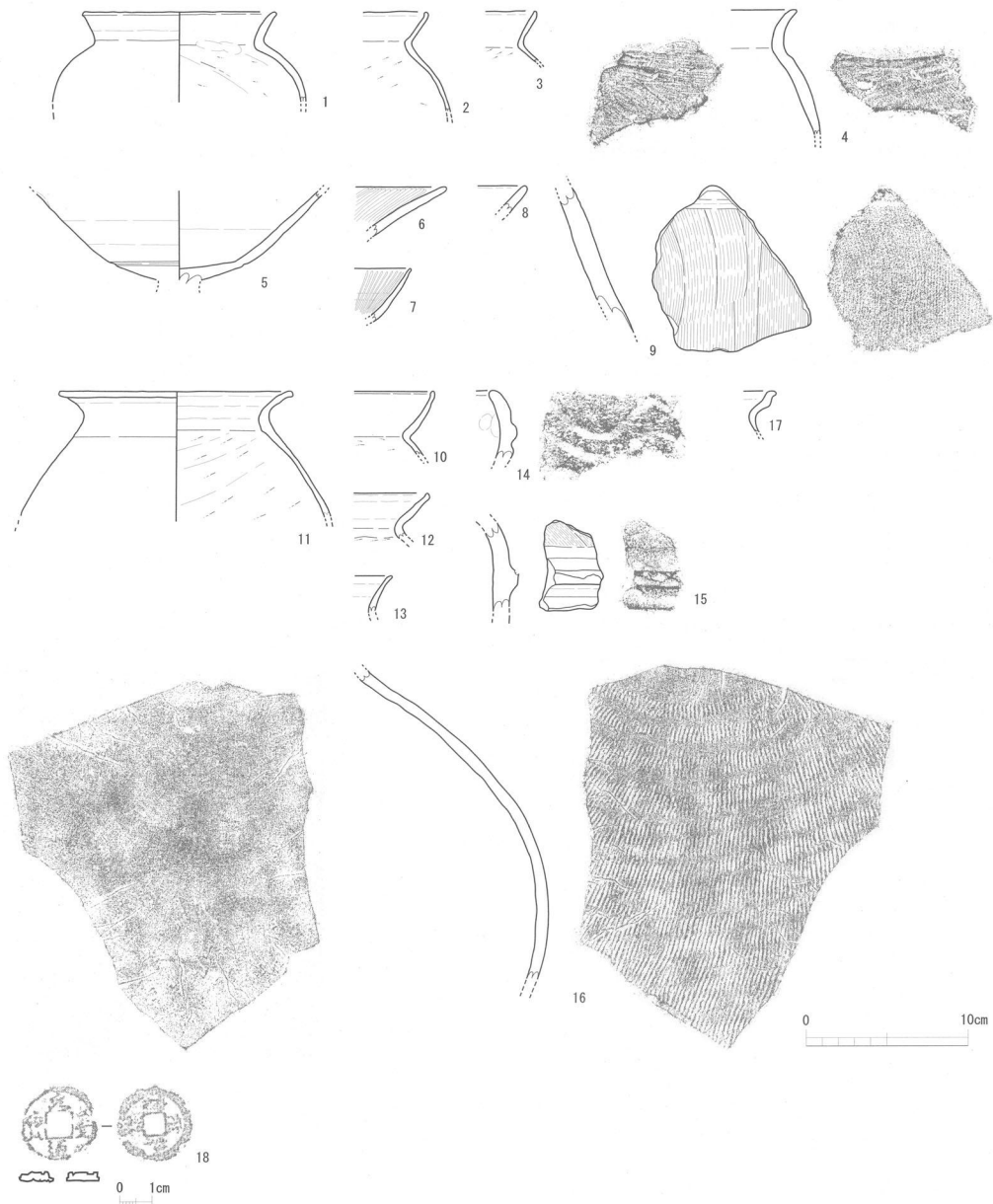
第23図 出土遺物実測図及び拓本（1～17はS=1/4、18は1/2）
