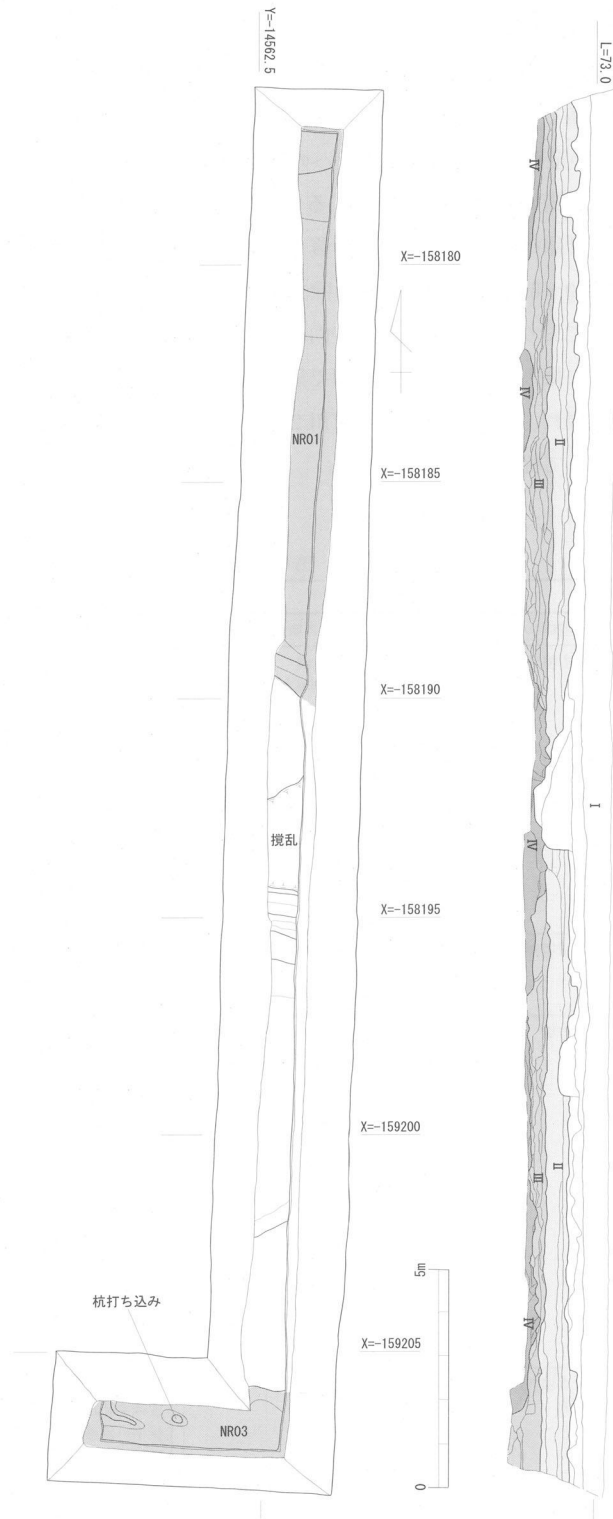
第22図 遺構配置図及び土層断面図 (1/150)
