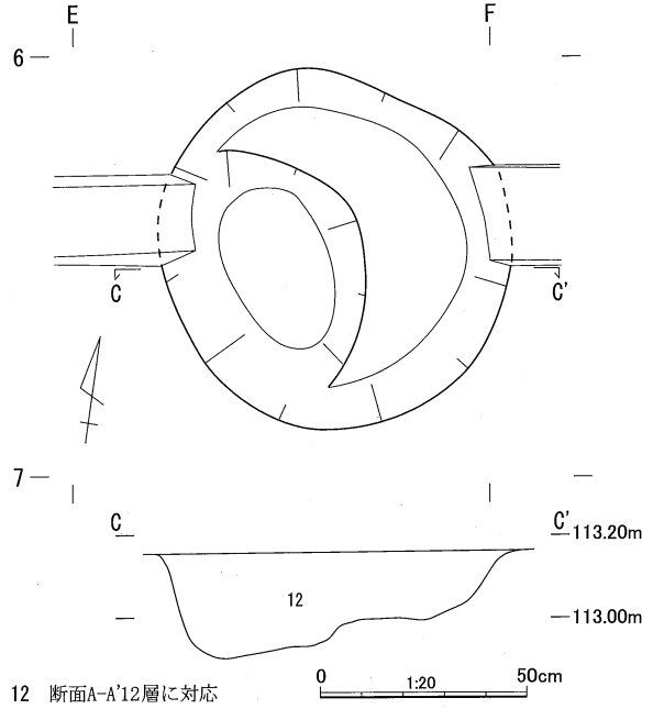
第10図 土坑平面図・土層図
