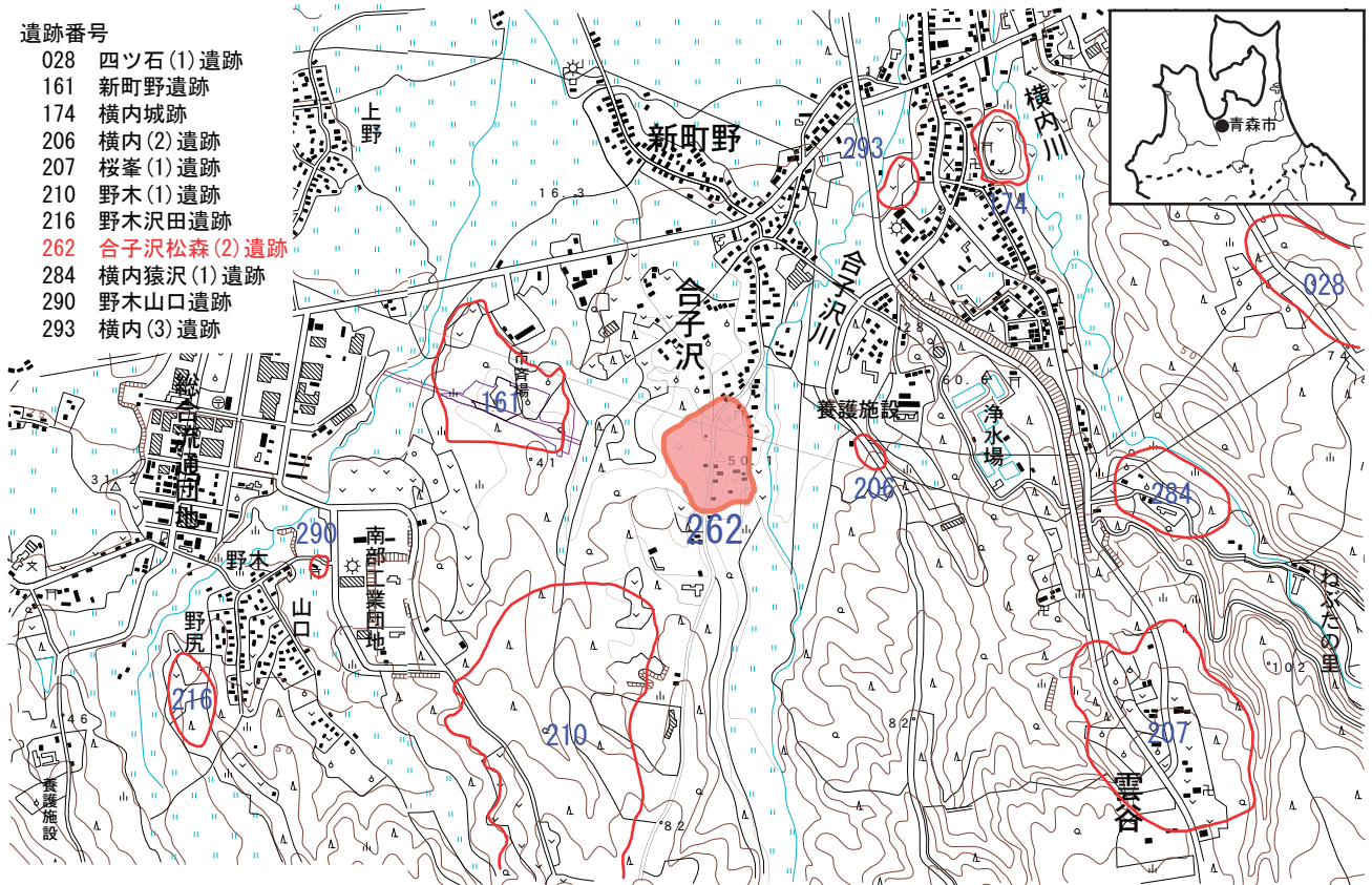
合子沢松森（2）遺跡及び周辺の平安時代の遺跡（1：25,000）
