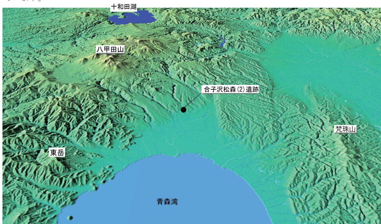
青森湾から見た合子沢松森（2）遺跡と周辺の地形（カシミール3D ver7.7.3を用いて作成）
