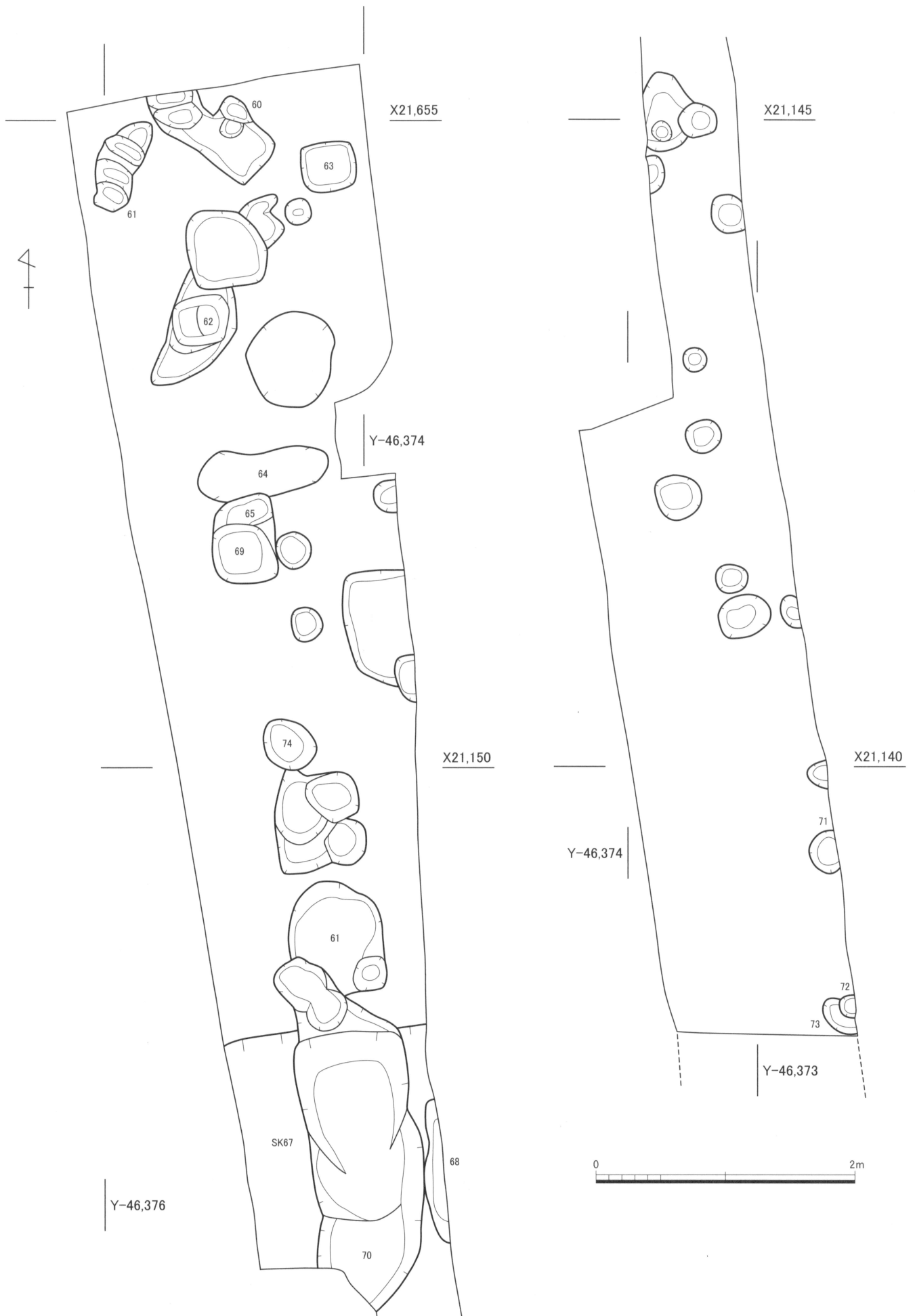
Fig.13 F区遺構全体図 (1/40)
