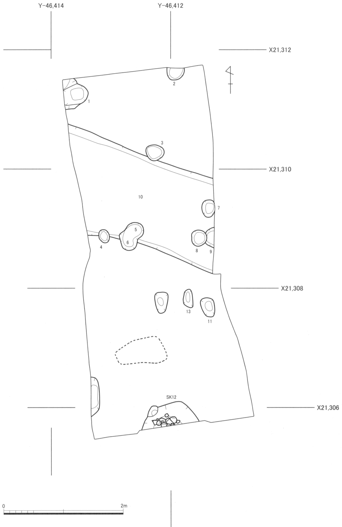
Fig.4 A区遺構全体図 (1/40)
