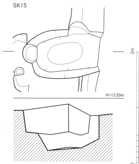
Fig.5 SK15 遺構実測図 (1/40)
