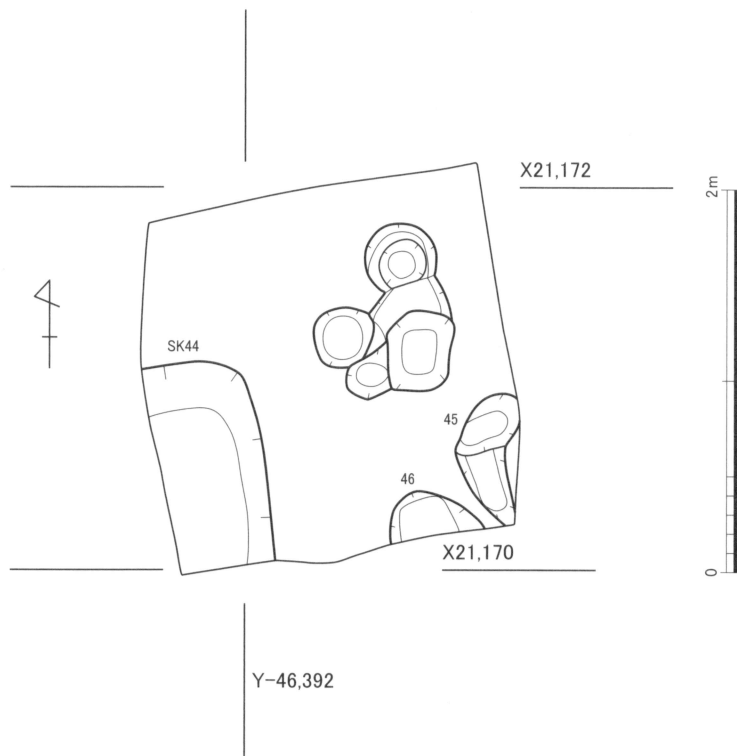
Fig.9 D区-2遺構全体図 (1/40)
