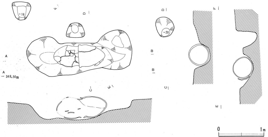
合口甕棺墓実測図
