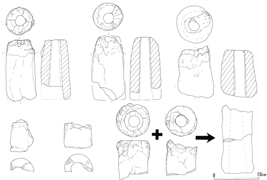
羽口実測図
