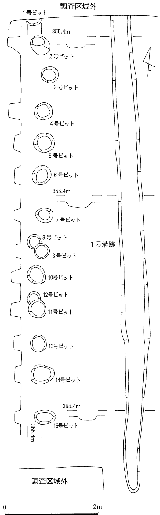
第8図 1号溝跡及びピット列 (1:50)
