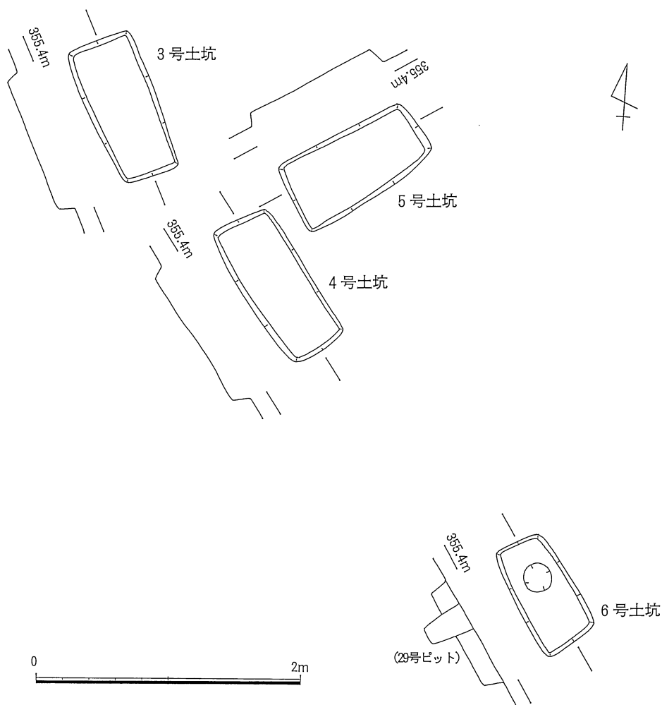
第7図 3号～6号土坑 (1:40)
