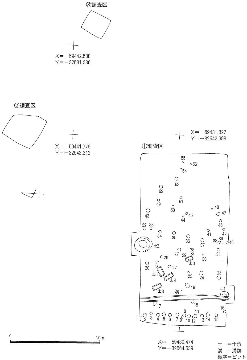
第4図 全体図 (1:200)
