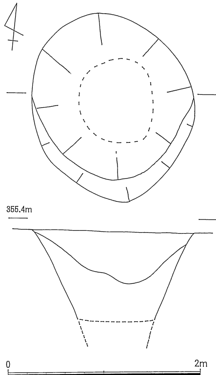
第6図 2号土坑（1：40）
