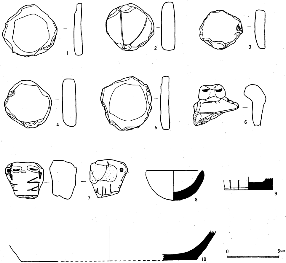
第11図 土製品及び土器実測図
