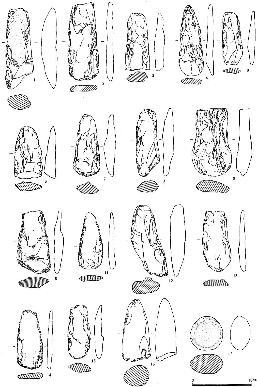
第17图 出土石器实测图
