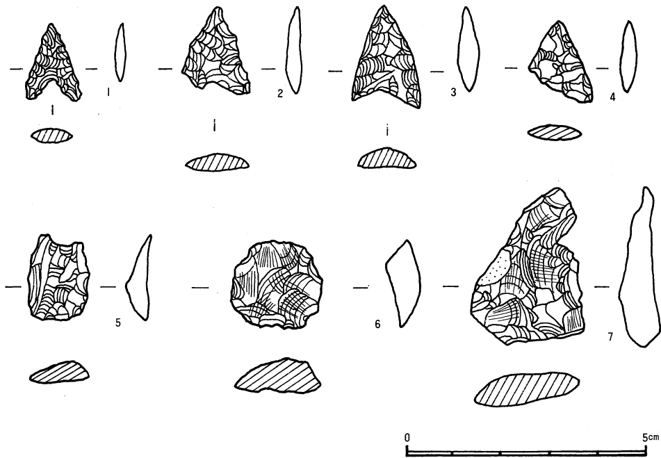
第16図 出土石器実測図
