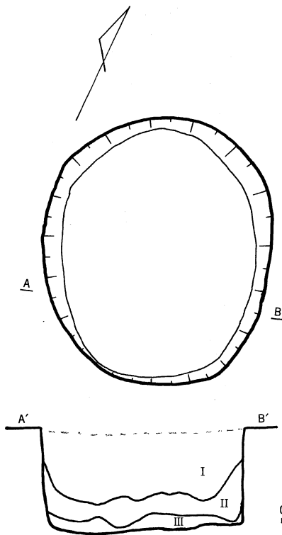
第9図 D-9号土抔実測図
