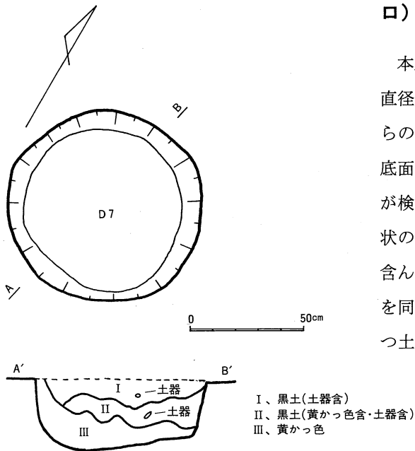
第7図 D-7号土坑実測図
