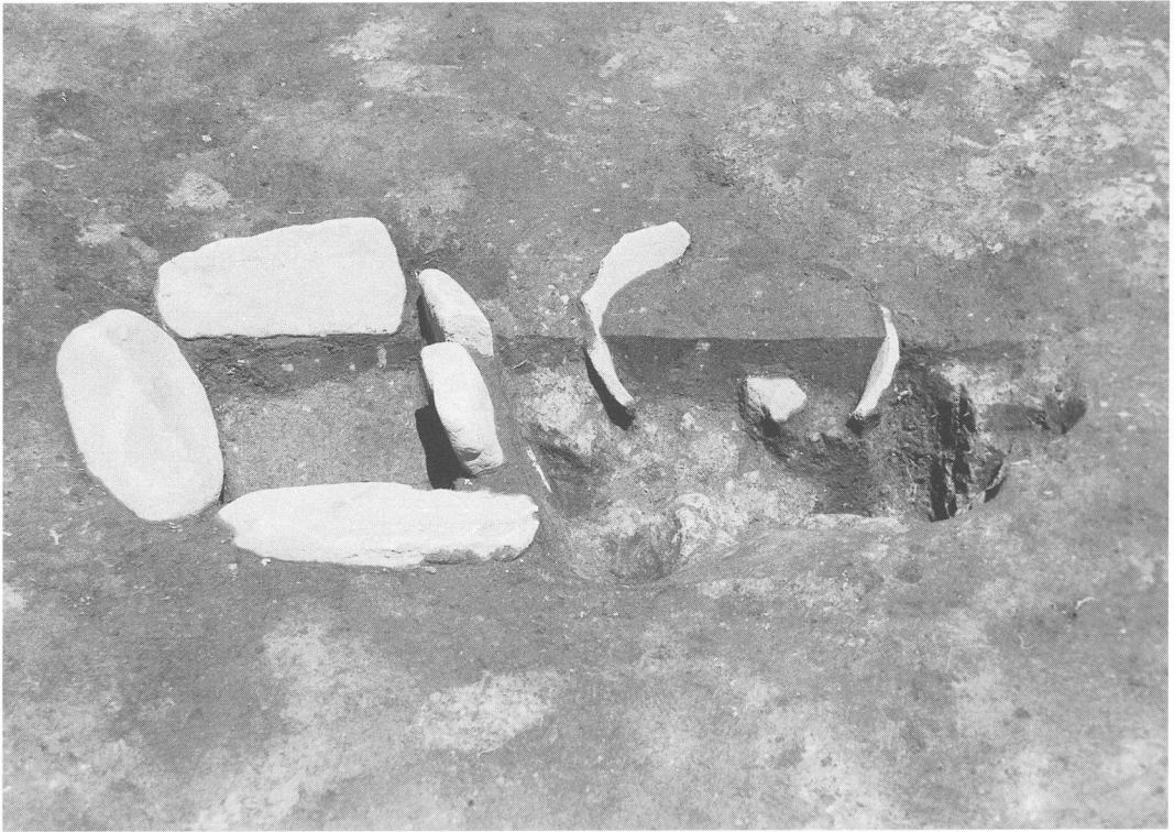
写真10 程久保遺跡第21号竪穴住居址方形石囲炉・埋甕炉（南から）
