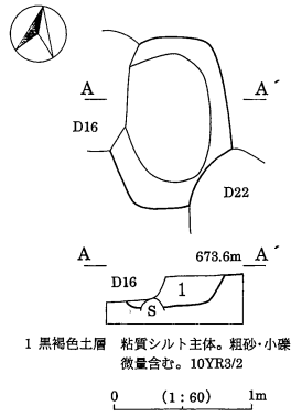
第25図 D18号土坑実測図
