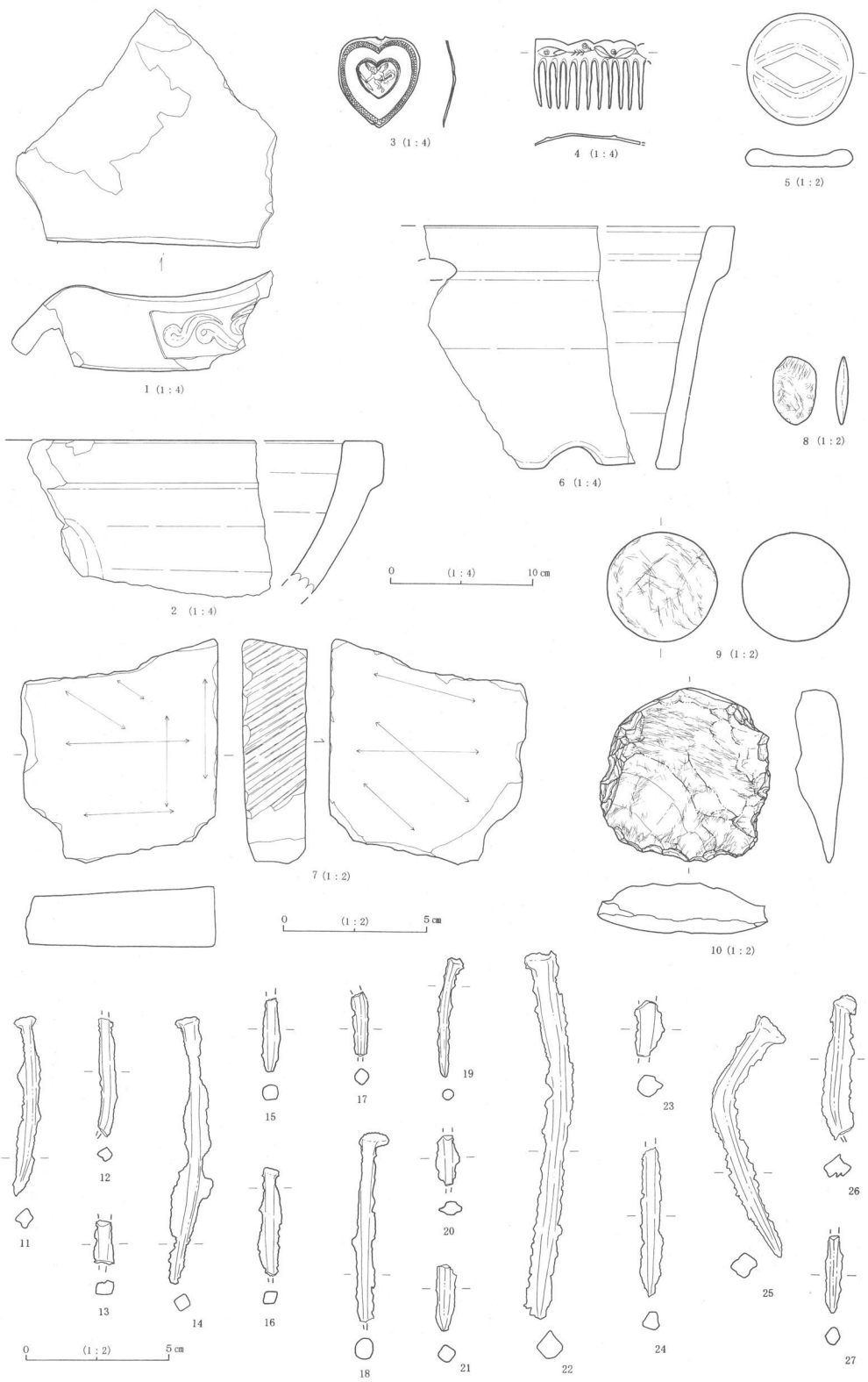
第42图 出土遺物実測図
