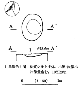
第30図 D25号土坑実測図
