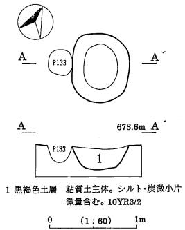
第36図 D30号土坑実測図
