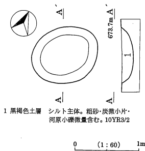
第7図 D1号土坑実測図
