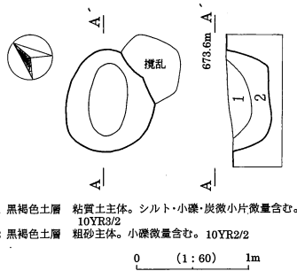
第35図 D29号土坑実測図
