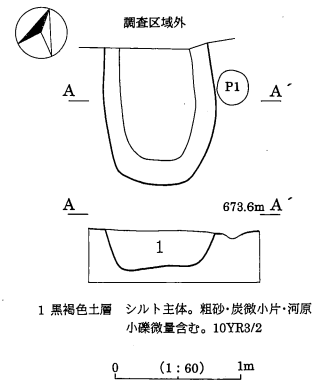
第12図 D5号土坑実測図
