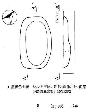
第10図 D3号土坑実測図
