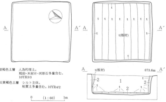
第38图 T1号特殊遗構实测图
