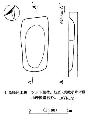
第11図 D4号土坑実測図
