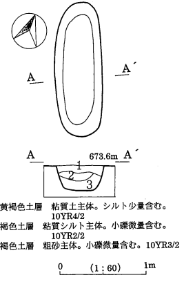
第27図 D21号土坑実測図
