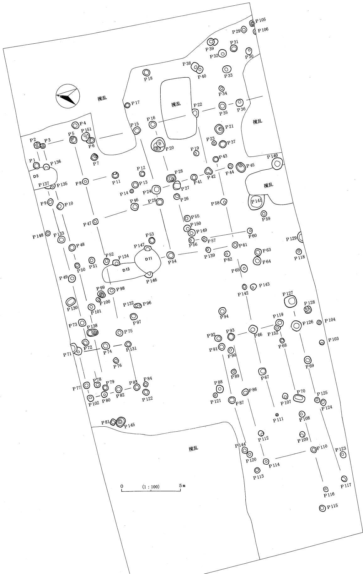
第40图 柱穴址实测图
