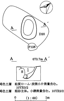
第32図 D26号土坑実測図
