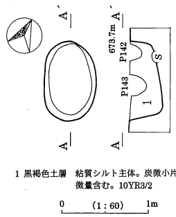
第29図 D24号土坑実測図
