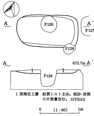
D26図 D20号土坑実測図
