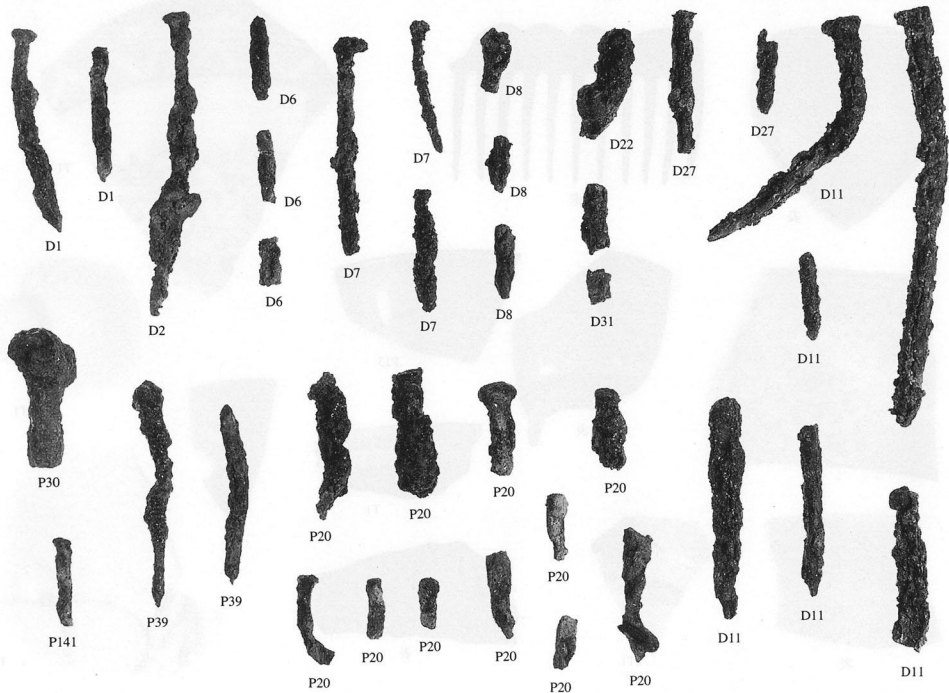
各遺構出土鉄製品（1：2）
