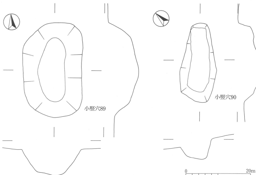
第5図 雁頭沢遺跡小竪穴89・90実測図 (1:60)
