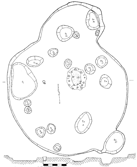
第15図 第8号住居址実測図(S=1/80)
