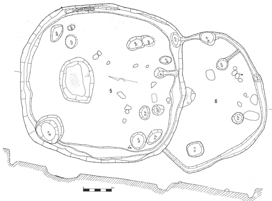
第10図 第5, 6号住居址実測図 (S=1/80)
