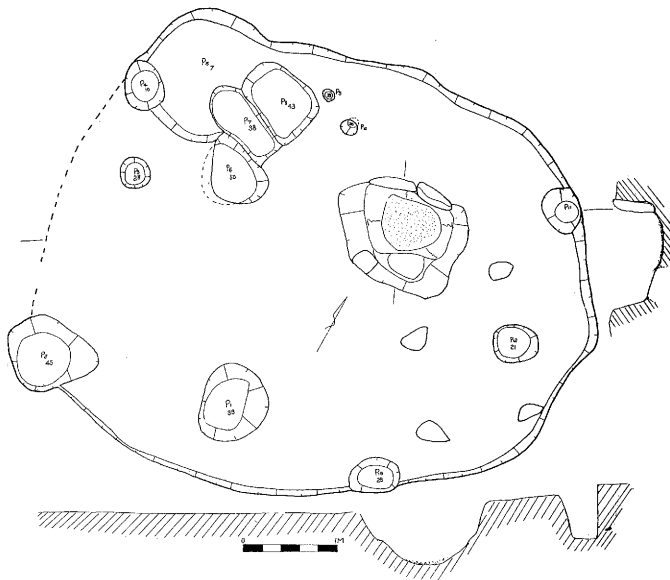
第7図 第3号住居址実測図 (S=1/80)
