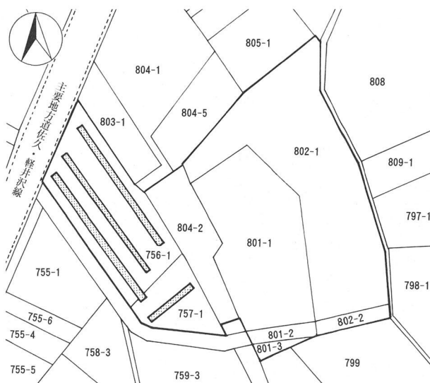
中金井遺跡群4 調査全体図 (1:1,500)
