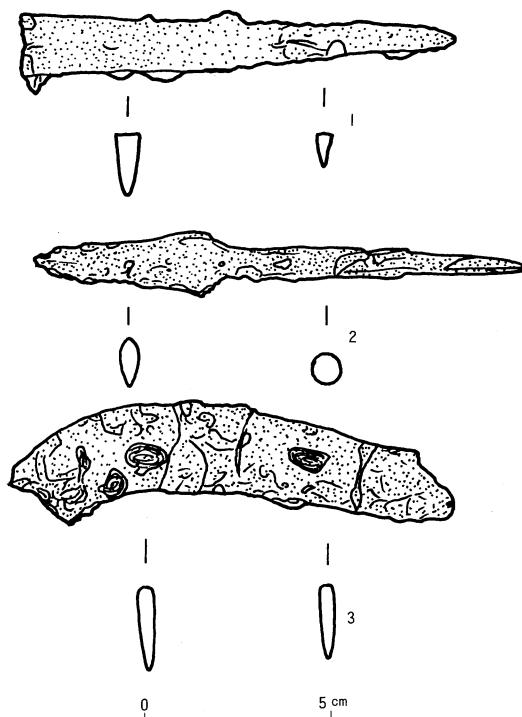
第25図 金属器実測図
