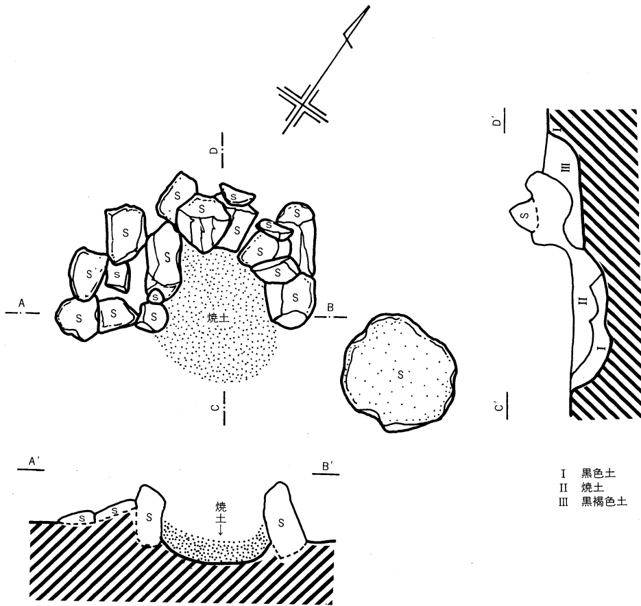
第4図 第1号住居址カマド実測図
