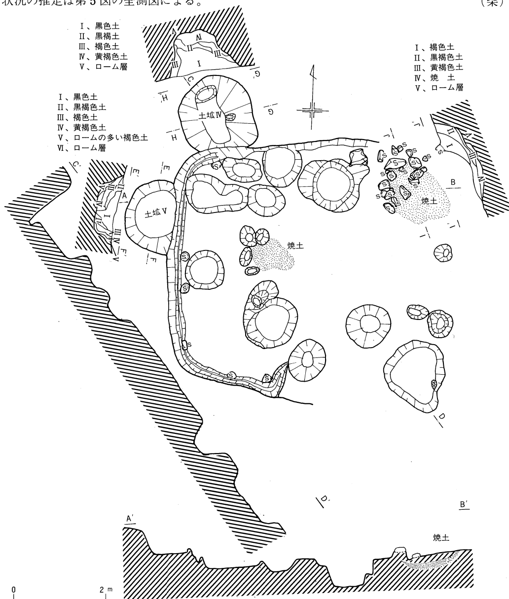
第6図 第1・4号住居址及び土坑Ⅳ・Ⅴ 実測図
