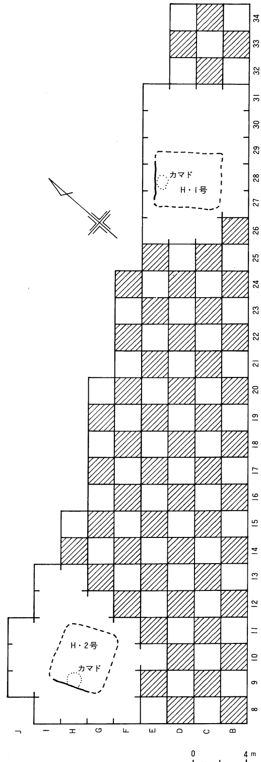
第2図 遺構全測図
