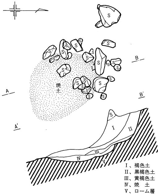
第9図 第1号住居址カマド実測図
