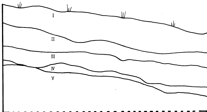
第4図 グリッド3 地層状況図
