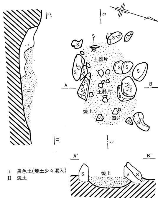
第6図 第2号住居址カマド実測図
