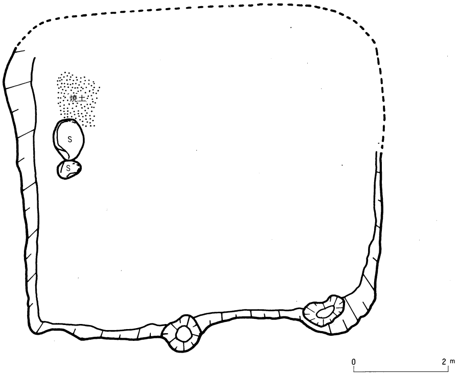
第14图 第6号住居址实测图
