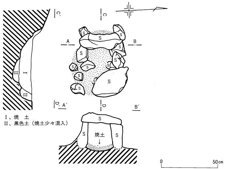
第16図 第5号住居址カマド実測図
