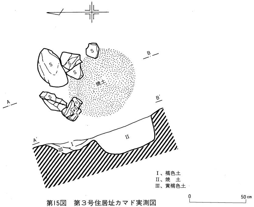
第15図 第3号住居址カマド実測図
