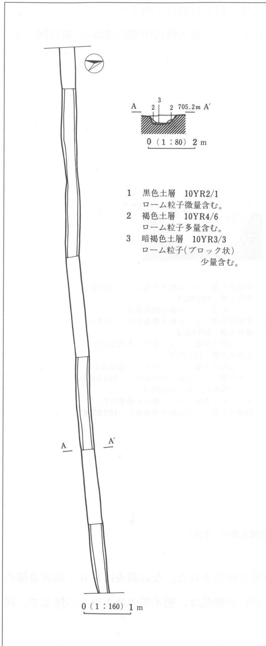
第9図 M1号溝状遺構実測図
