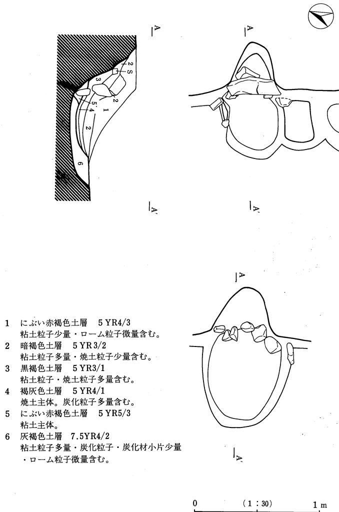
第6図 H1号住居址カマド実測図
