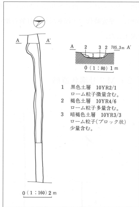
第10図 M1号溝状遺構実測図
