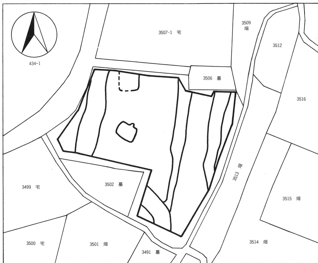
石並城跡試掘調査全体図 (1 : 500)
