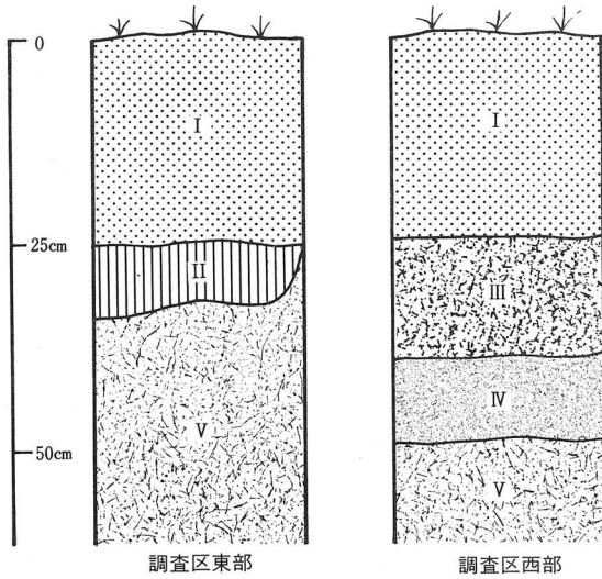
芝宮遺跡群2基本土層模式図
