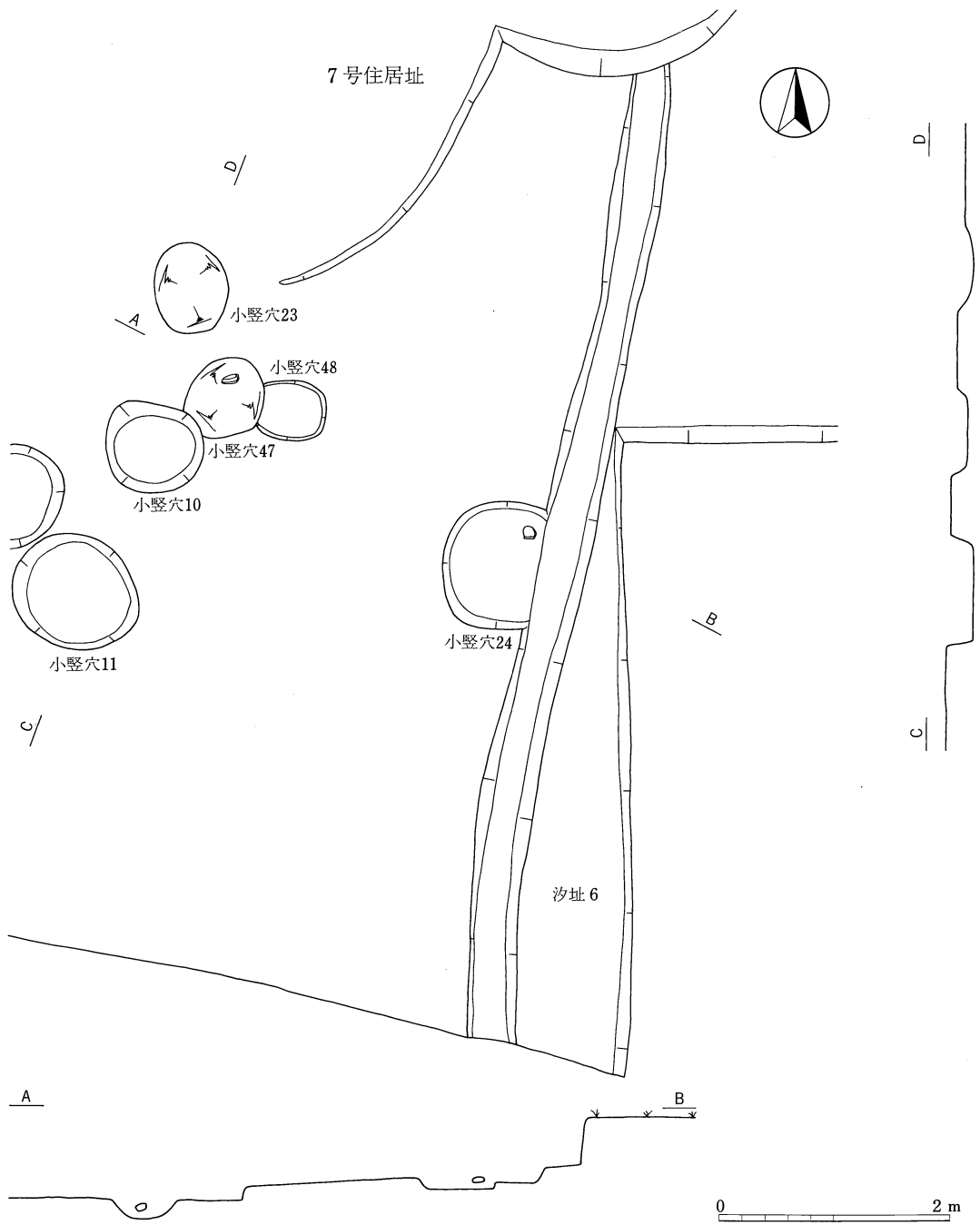
第12图 小竖穴・汐址实测图 (1:60)
