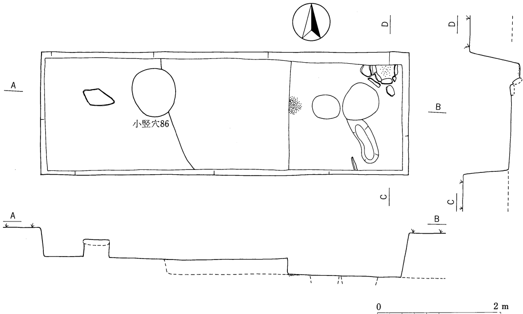
第8図 第4号住居址実測図(1:60)
