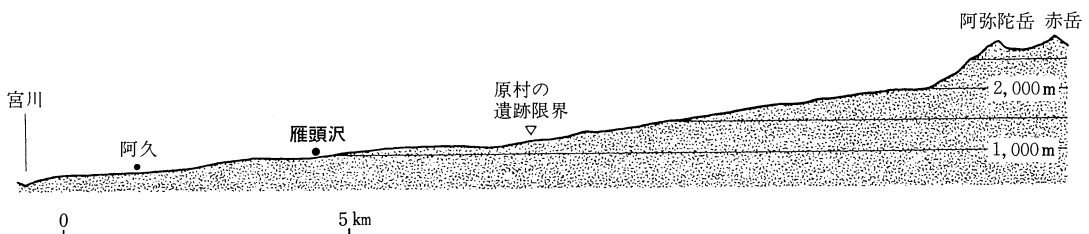
第1図 原村域の地形断面図模式図（赤岳—雁頭沢—宮川ライン）
