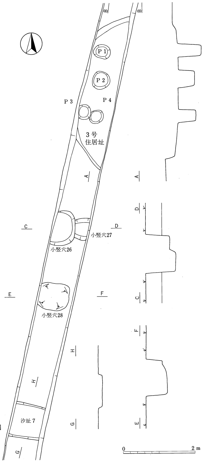
第7図 第3号住居址・ 小竖穴・汐址実測図 (1 : 60)
