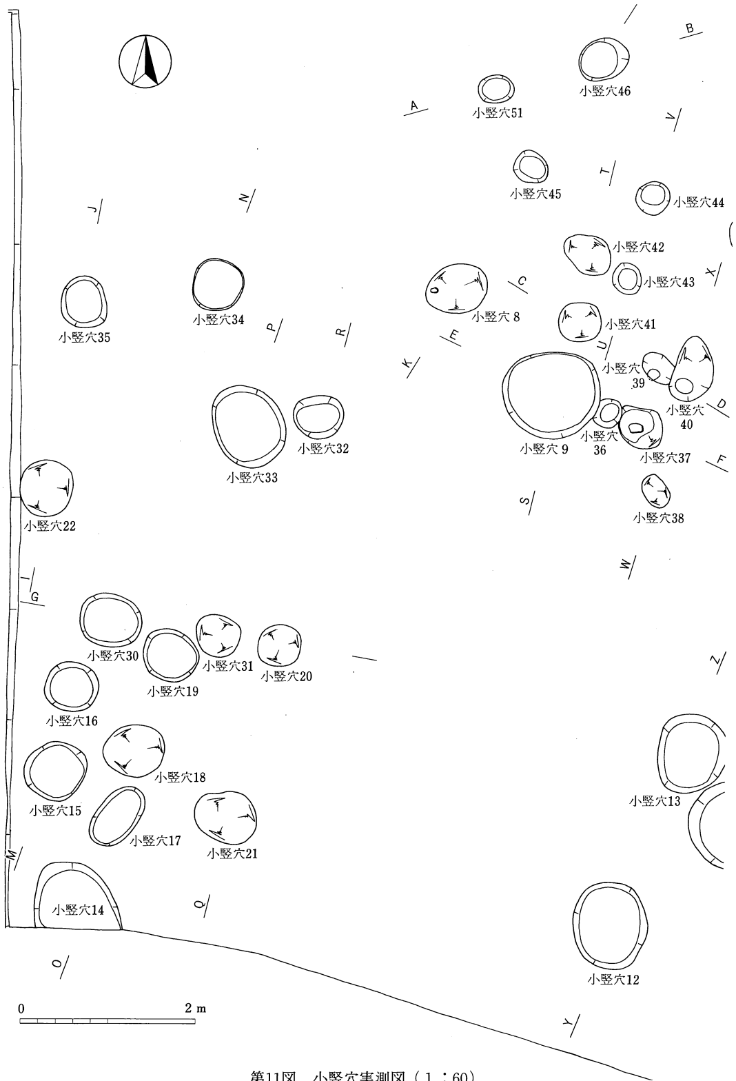
第11图 小竖穴实测图 (1 : 60)
