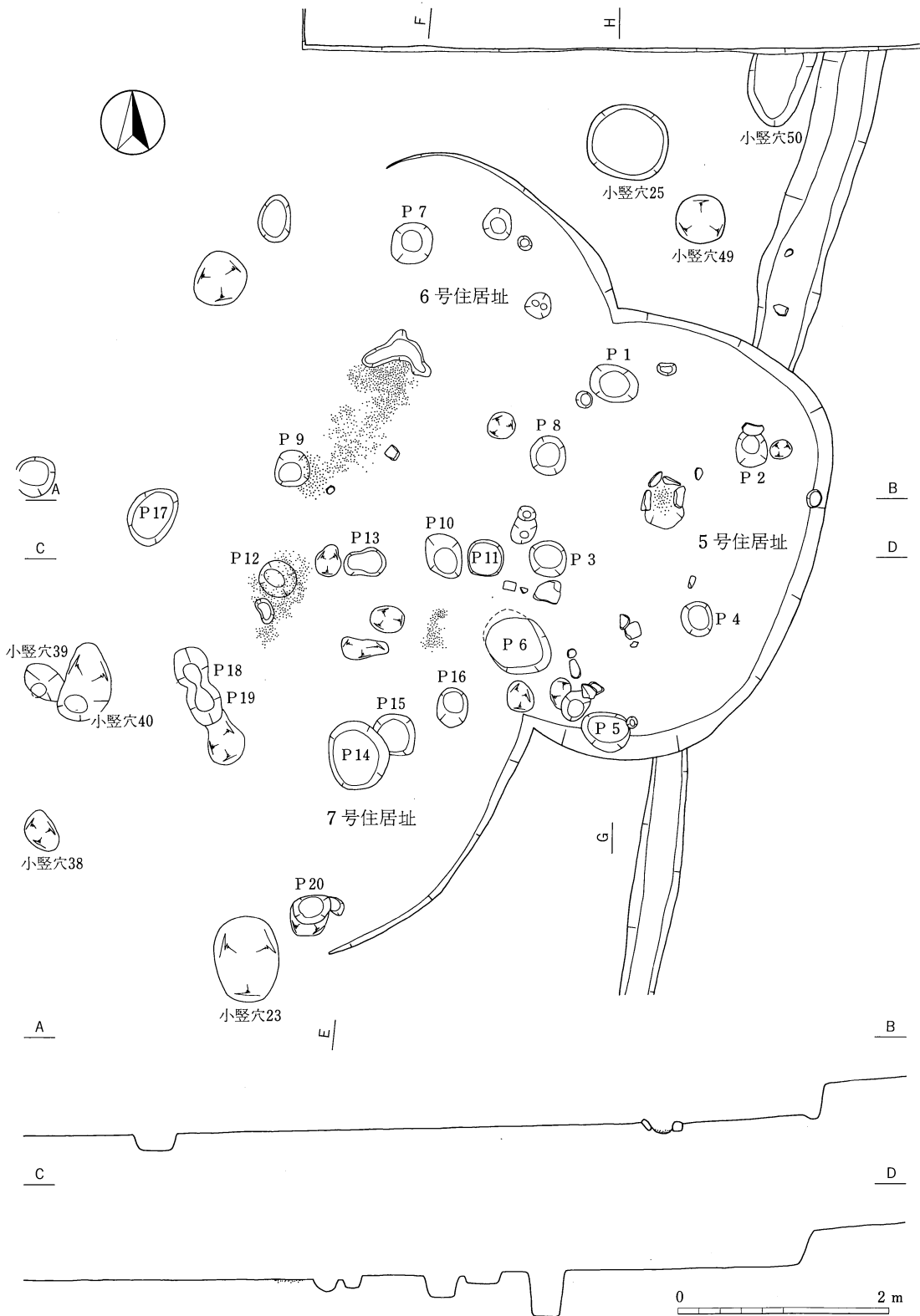
第9图 第5·6·7号住居址·小竖穴·汐址实测图 (1:60)
