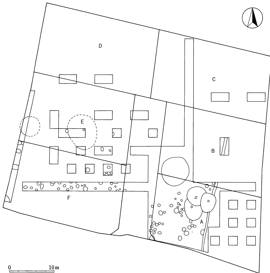
第4図 造成区画と遺構配置図（1：500）
