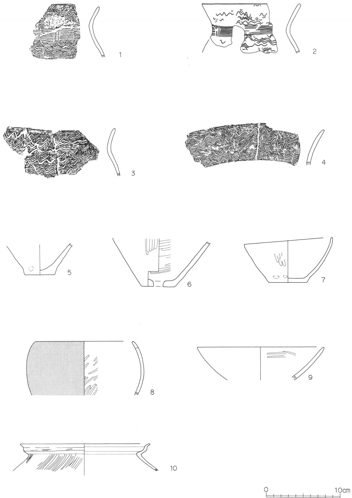
第5図 第1号住居址出土遺物実測図
