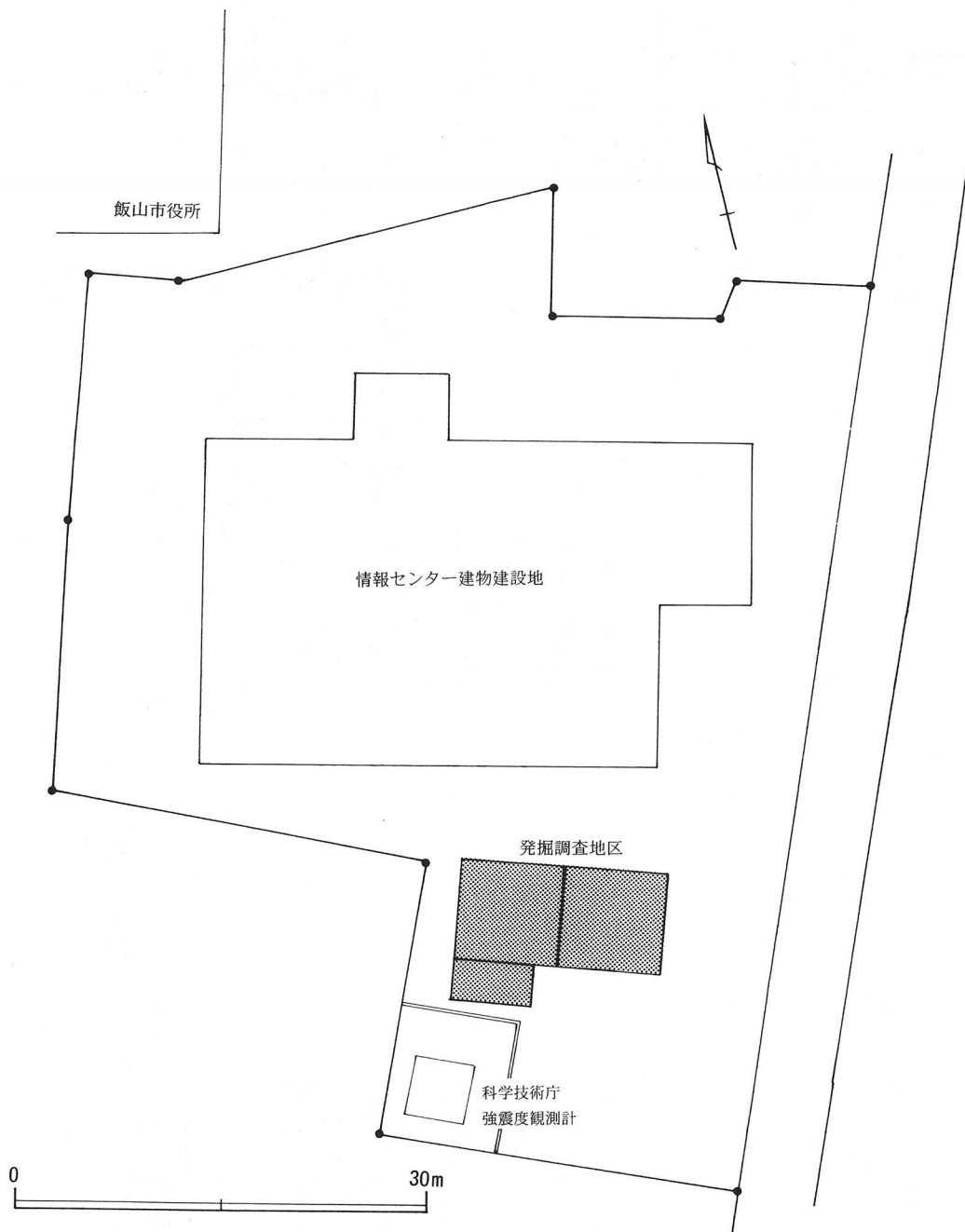
図3 調査地平面図 (1 : 500)
