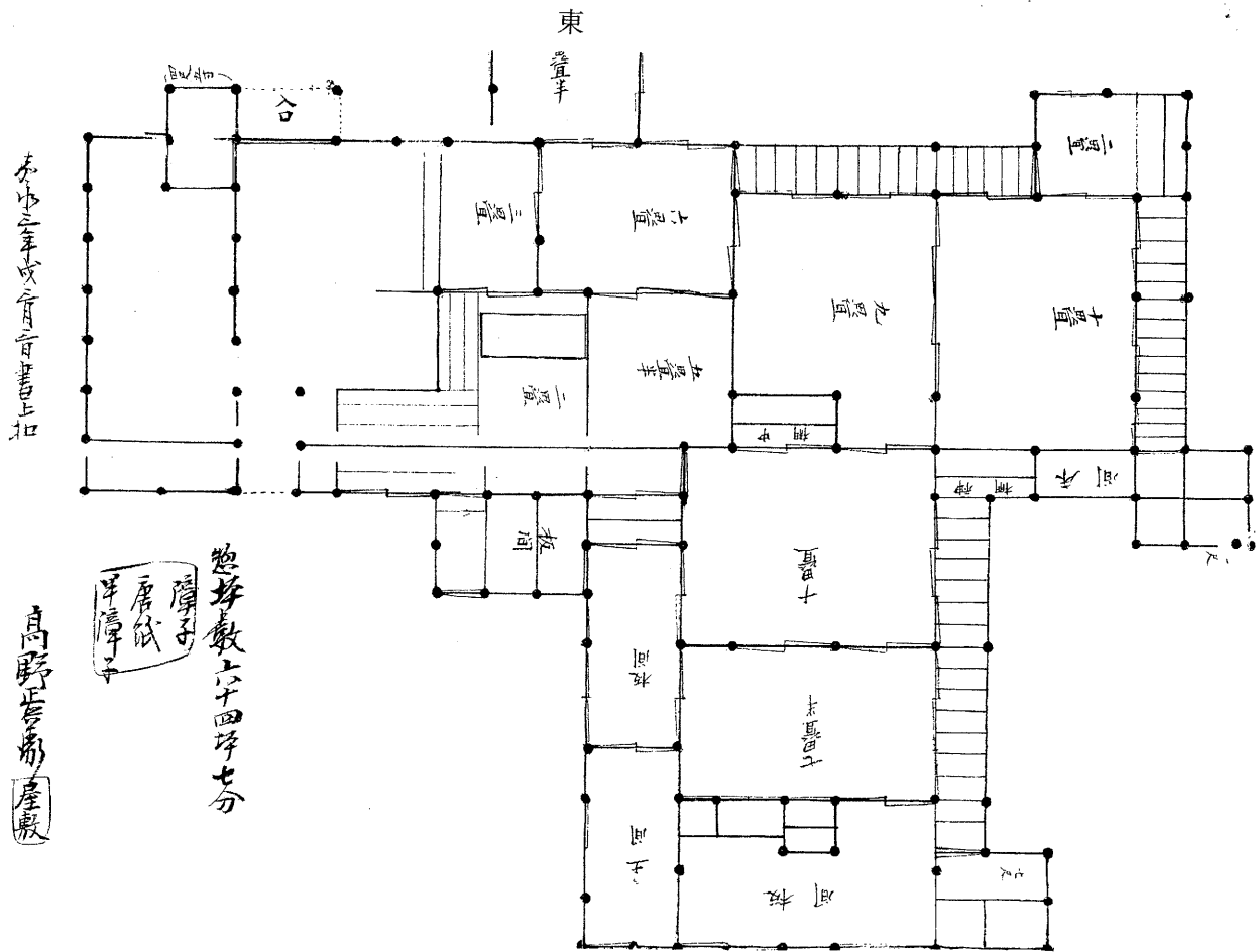
図8 高野正兵衛氏宅間取り図写・縮小（矢口迪子氏所蔵）
