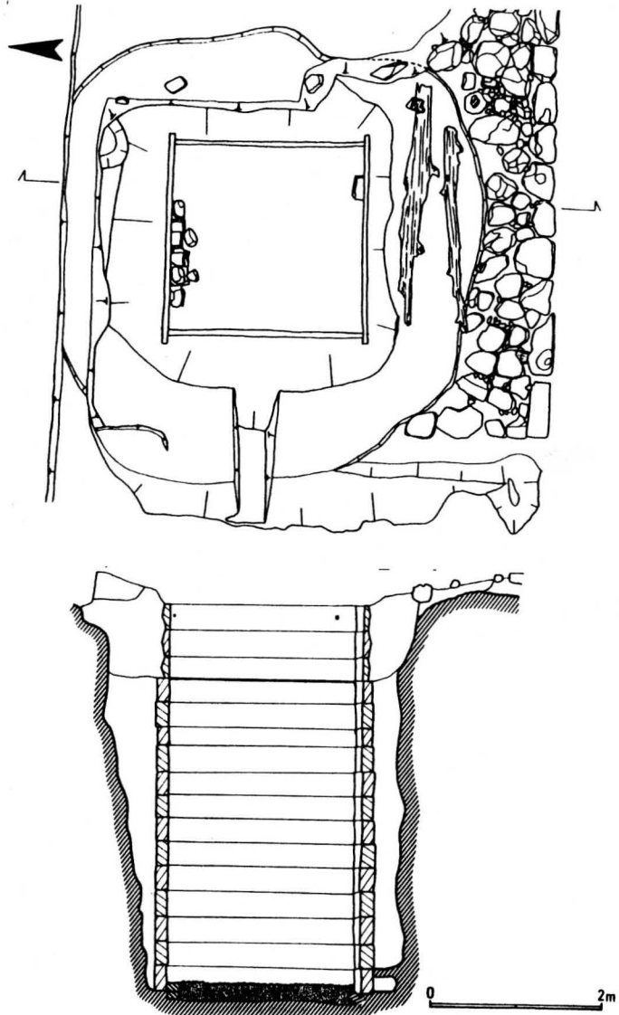
井戸の平面及び断面図 1/80
