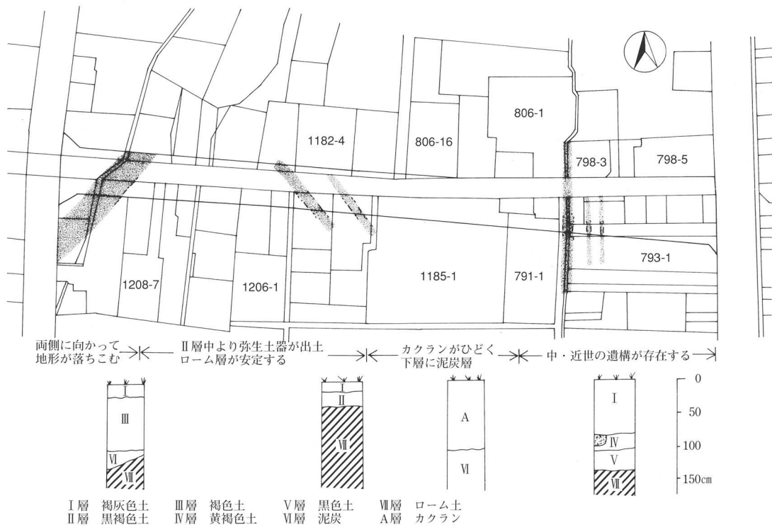
岩村田遺跡群 25 調査全体図 (1:2,000)
