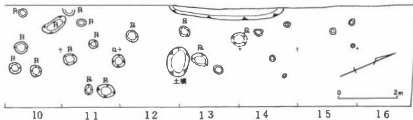
第10図 H地区 遺構配置図(1:120)
