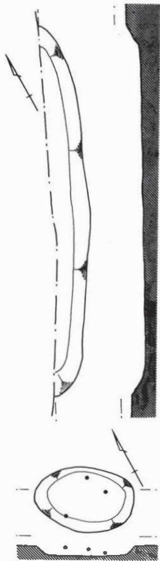
第12図 竪穴遺構・土坑(1:40)
