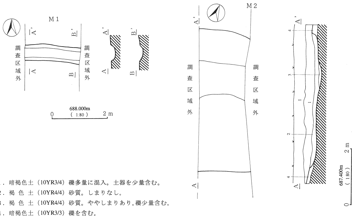
第10図 M1・2号溝状遺構実測図
