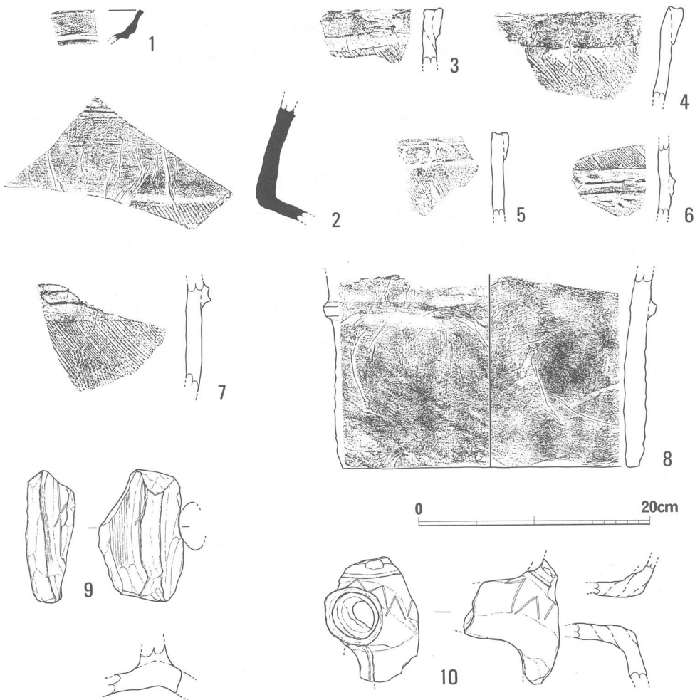
図13 出土遺物実測図1 (S=1/4)
