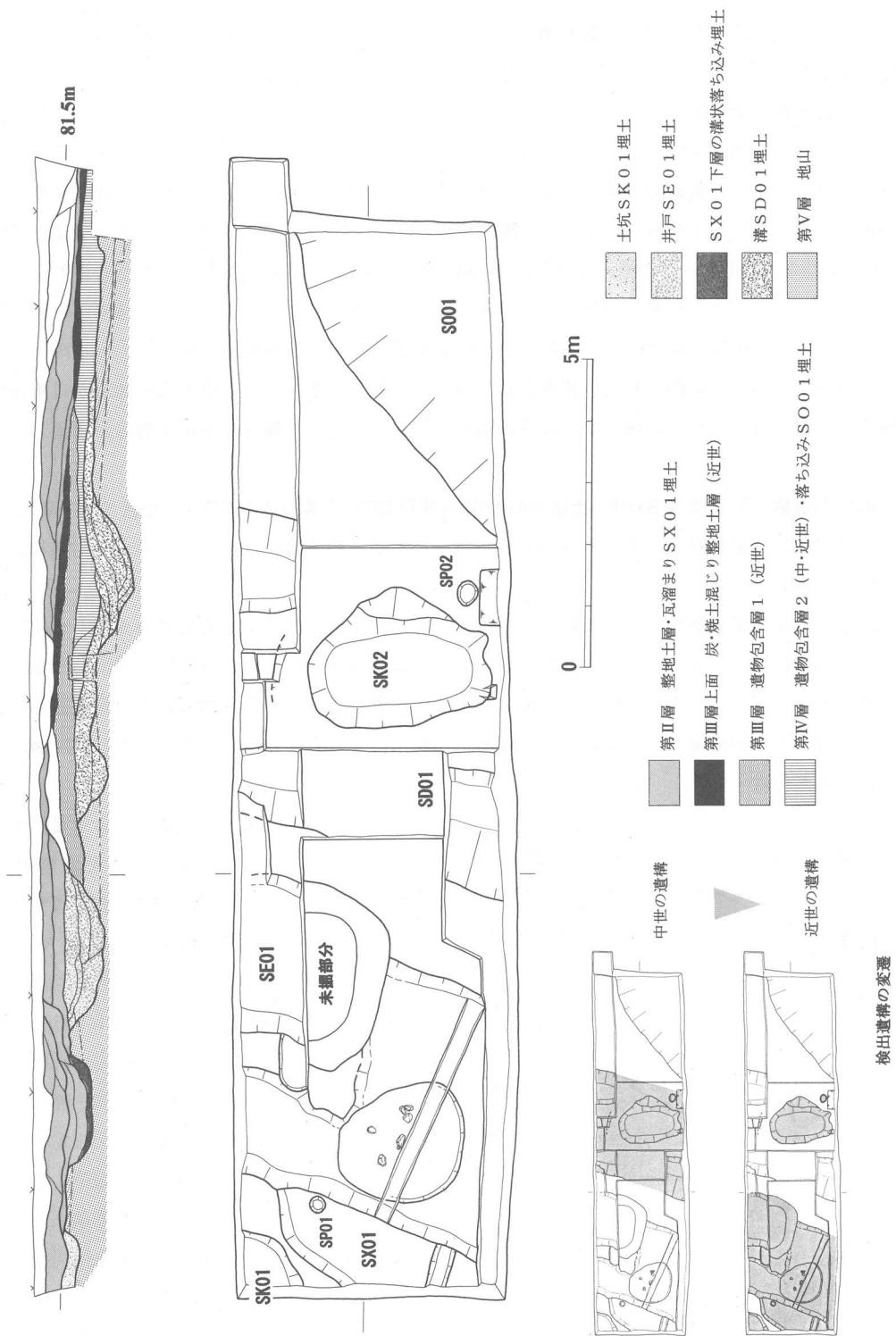
図3 第6次調査区平面・土層図 (S=1/100)
