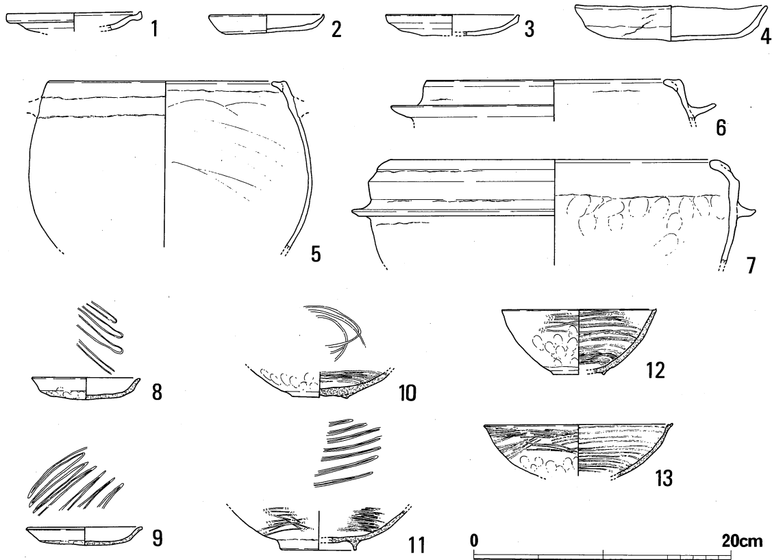
図5 出土遺物実測図1 (S=1/4)
