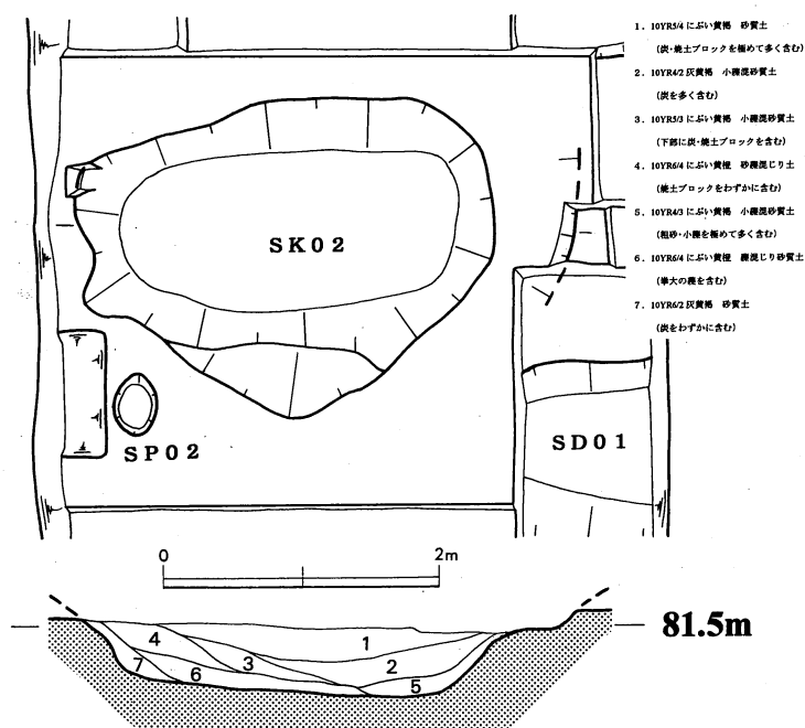
図4 土坑SK-02 平面・土層図 (S=1/60)
