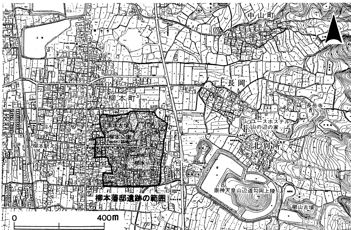
図1 遺跡の位置図 (S=1/10000)
