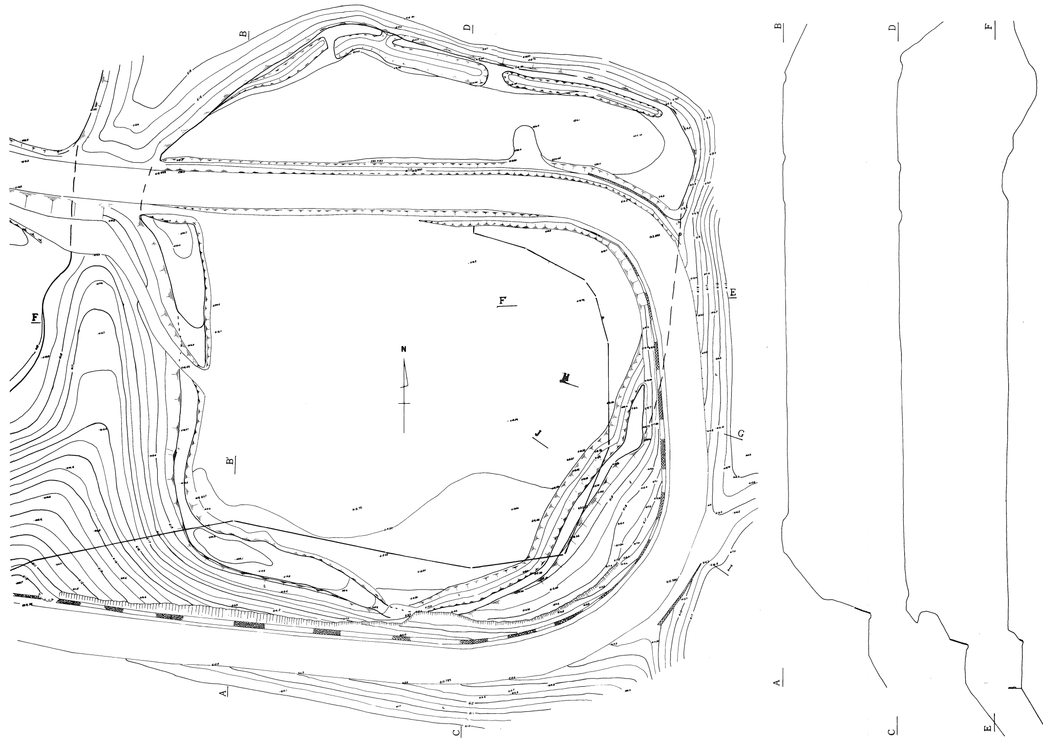
第5図 赤須城本郭跡測量図 (S=1:400) (水糸レベルは620.00m)
