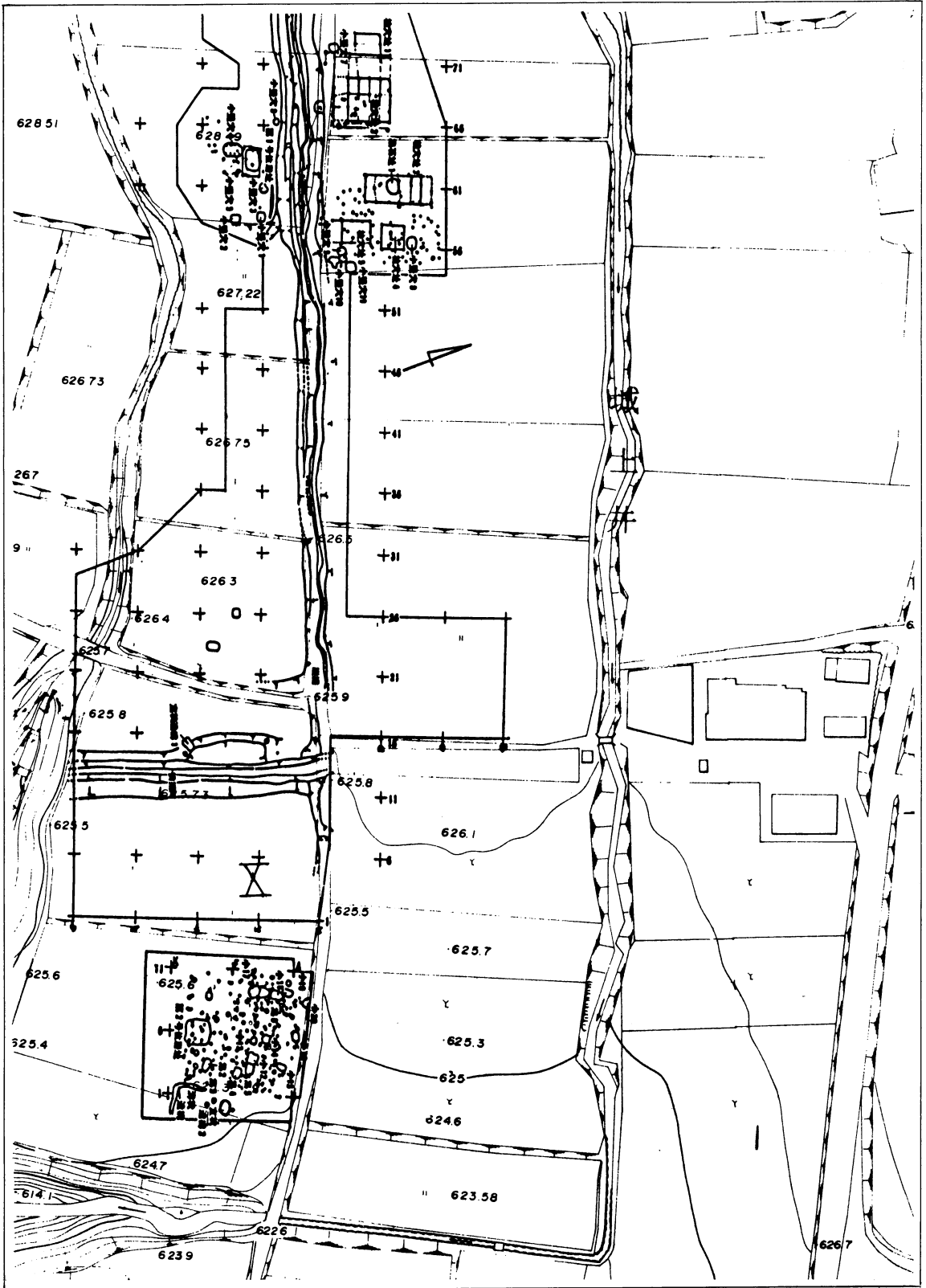
第4図 赤須城第1次調査遺構概略図 (S = 1:1,000)
