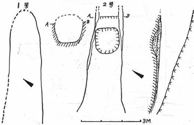
第3図 1、2号窯址実測図
