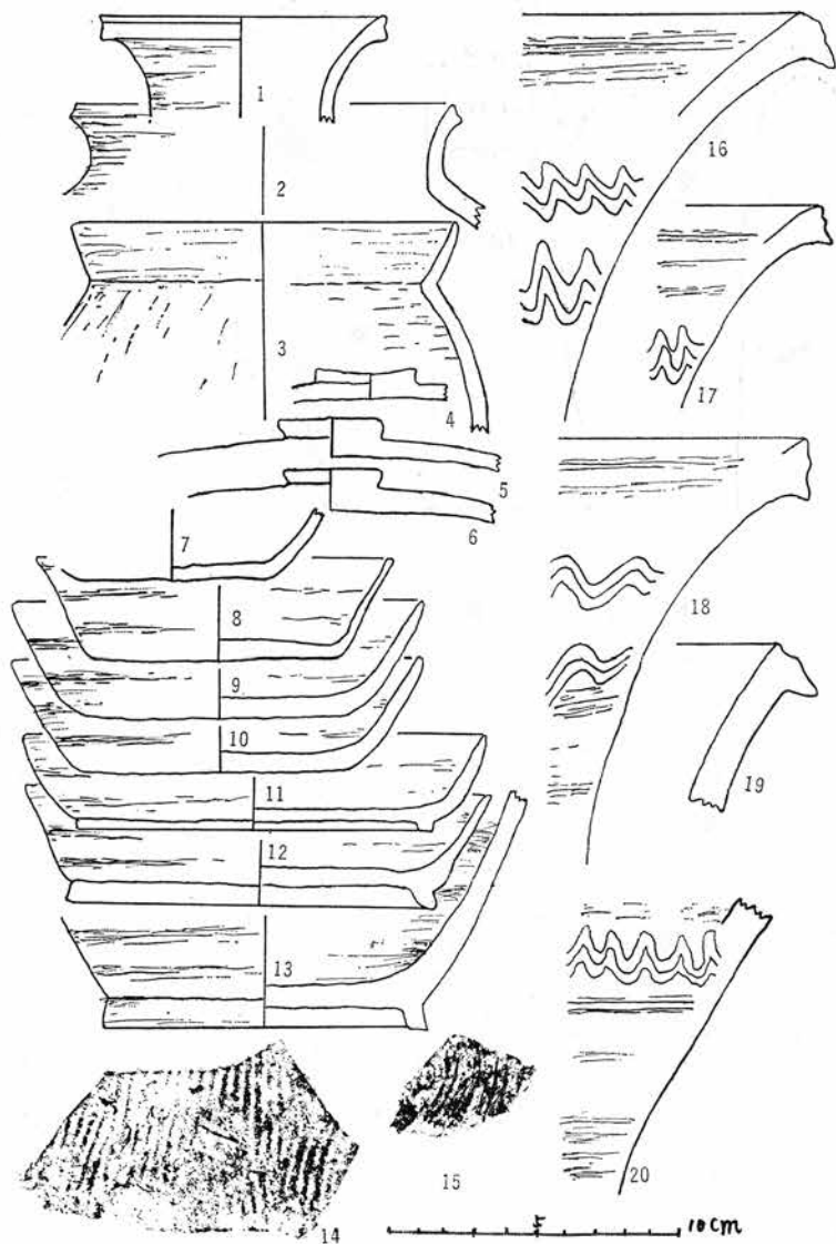
第4図 遺物実測図
