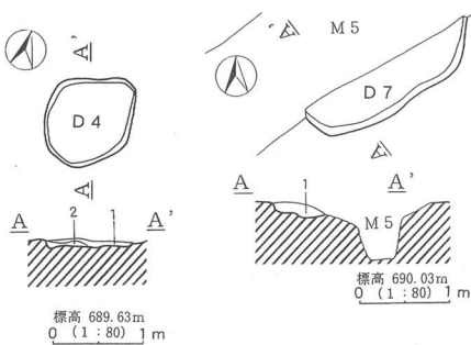
第36図 D 4・D 7号土坑実測図
