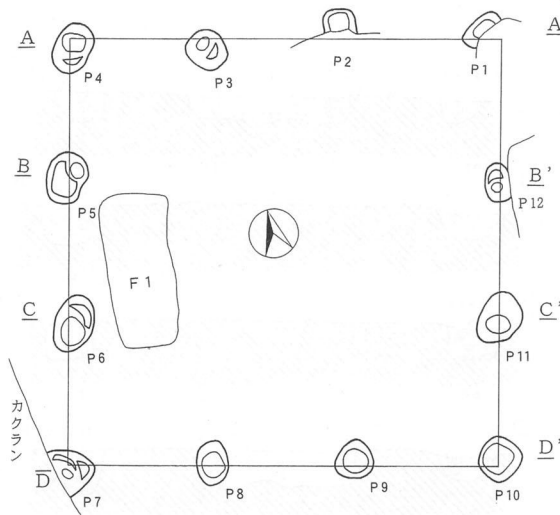
第22図 F5号掘立柱建物址
