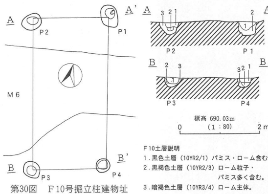
第30図 F 10号掘立柱建物址
