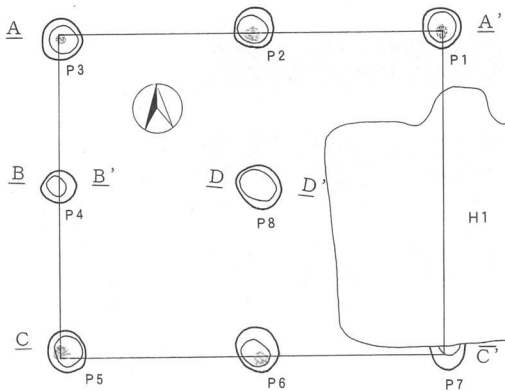
第25図 F 9号掘立柱建物址
