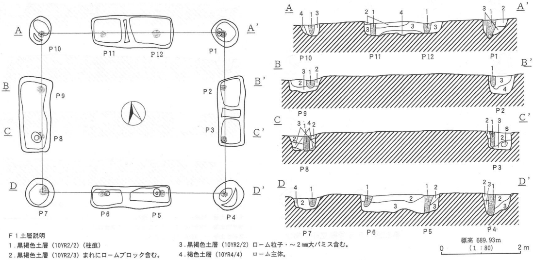
第21図 F 1 号掘立柱建物址
