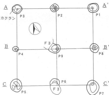
第27図 F 8号掘立柱建物址
