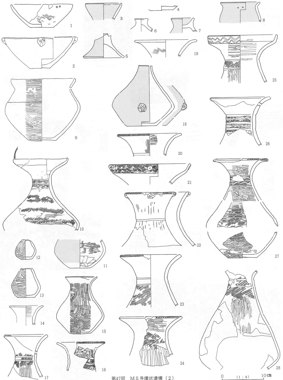
第47图 M5号沟状遗構 (2)
