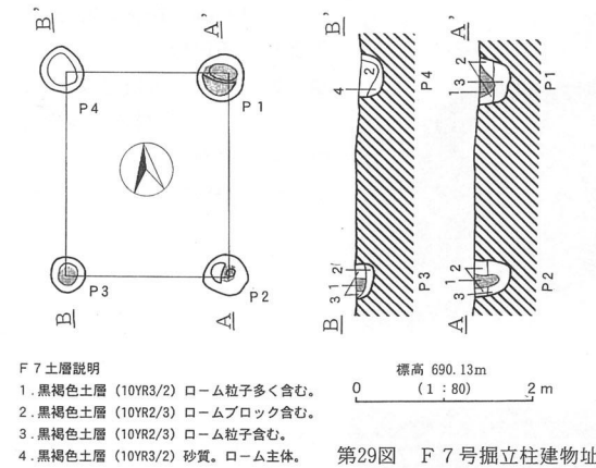
第29図 F 7号掘立柱建物址
