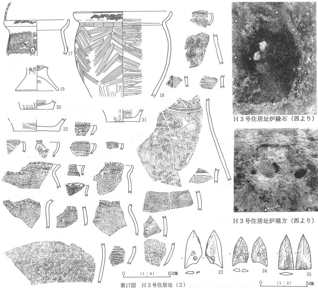
第17図 H3号住居址(2)
