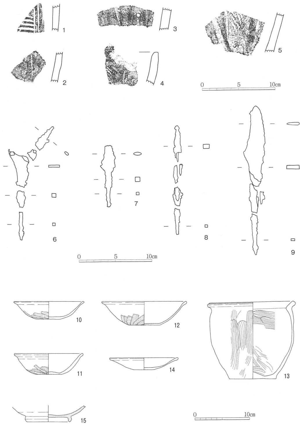
第6図 南長尾遺跡土器拓影・鉄製品・土器実測図 1~9 (1:3)、10~14 (1:4)
