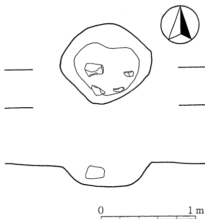
第3図 追分沢遺跡 小竪穴実測図 (1:40)
