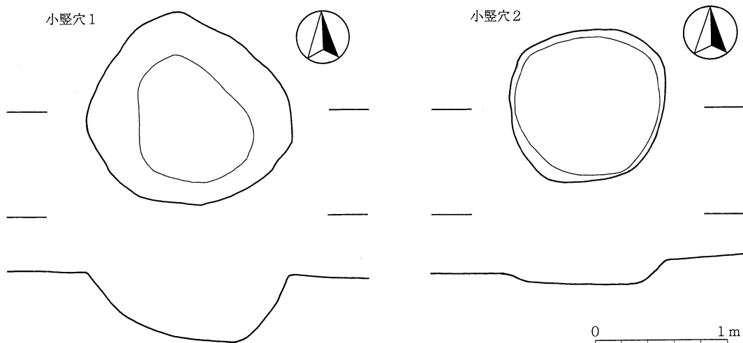
第8図 南長尾遺跡 小竪穴1・2実測図（1：40）
