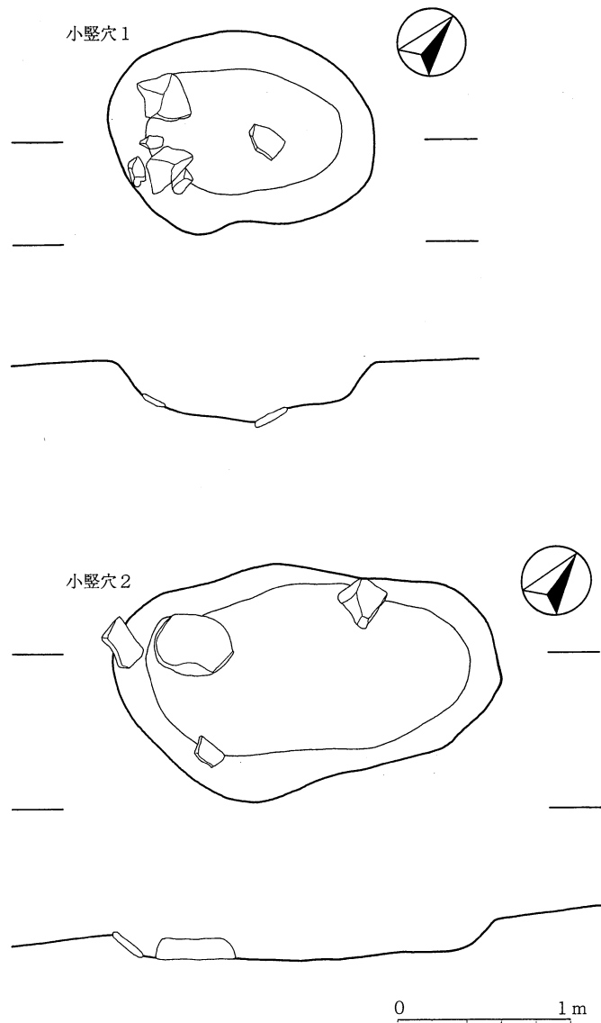
第10図 二枚田遺跡 小竪穴実測図 (1:40)
